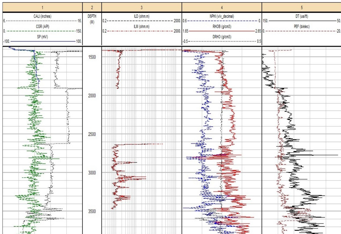
Figura 3.1: Registros geofísicos del pozo Terrígeno A a escala completa.
