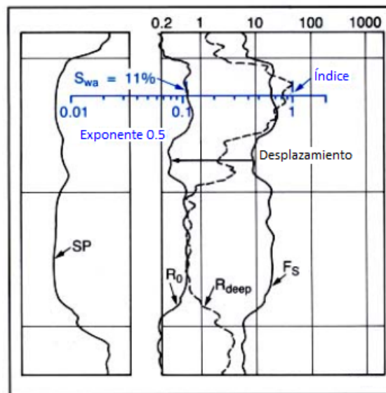
Figura 2.3: Superposición de R_o a partir de una curva F obtenida de un registro sónico. Tomado de Schlumberger (1978).
