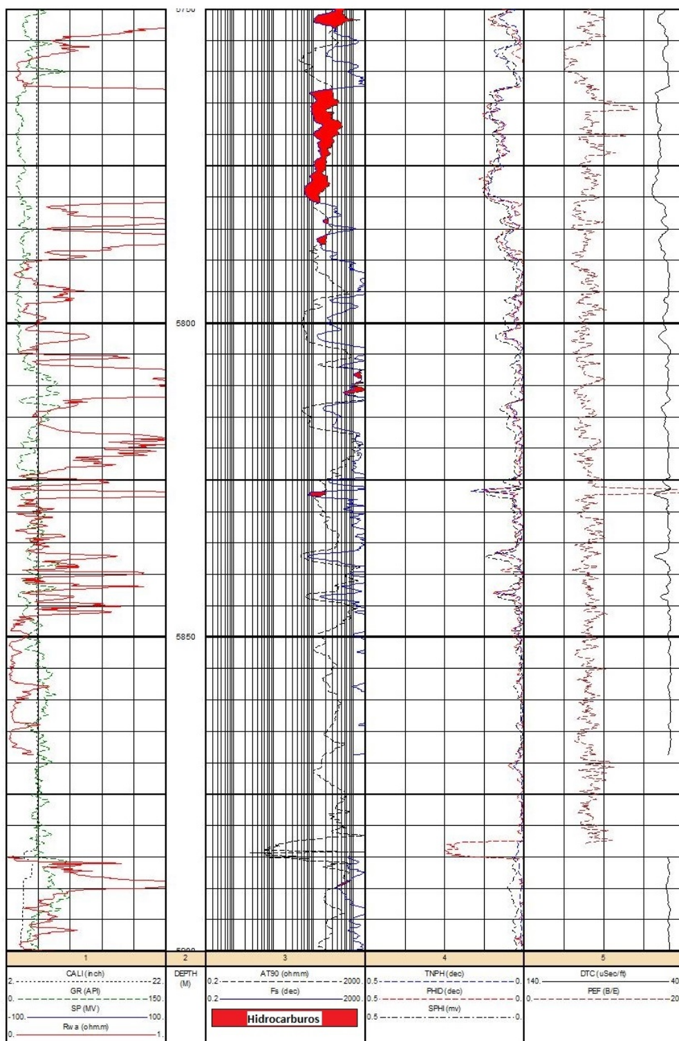
Figura 3.20: Determinación de hidrocarburos en el pozo Carbonato A mediante quick looks en el intervalo de 5,750 m a 5,900 m.
