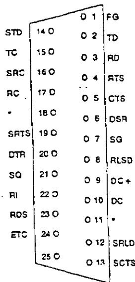
RS-232
