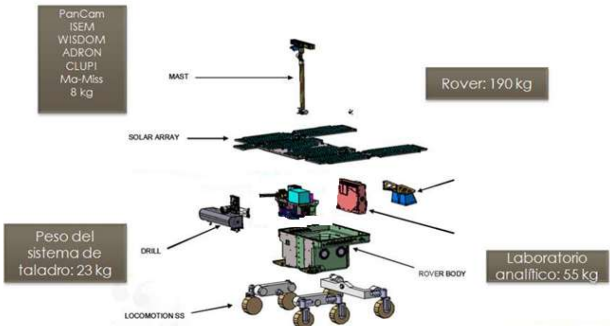
Figura 3.2 Partes del Rover ExoMars. ESA (Modificado de Baglioni, P. Planetary Rover Workshop , 2013).
