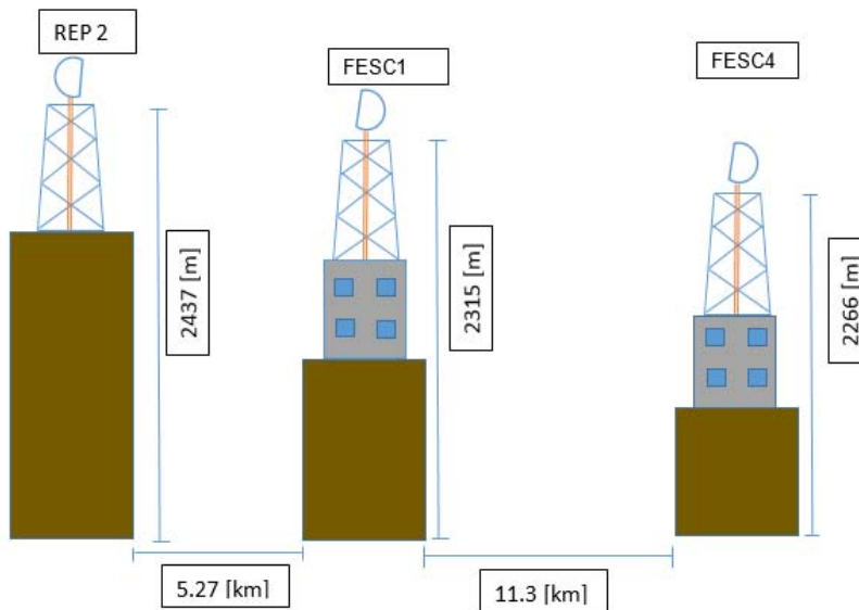
Figura 7.29 Vista General Enlaces Repetidor 2.
