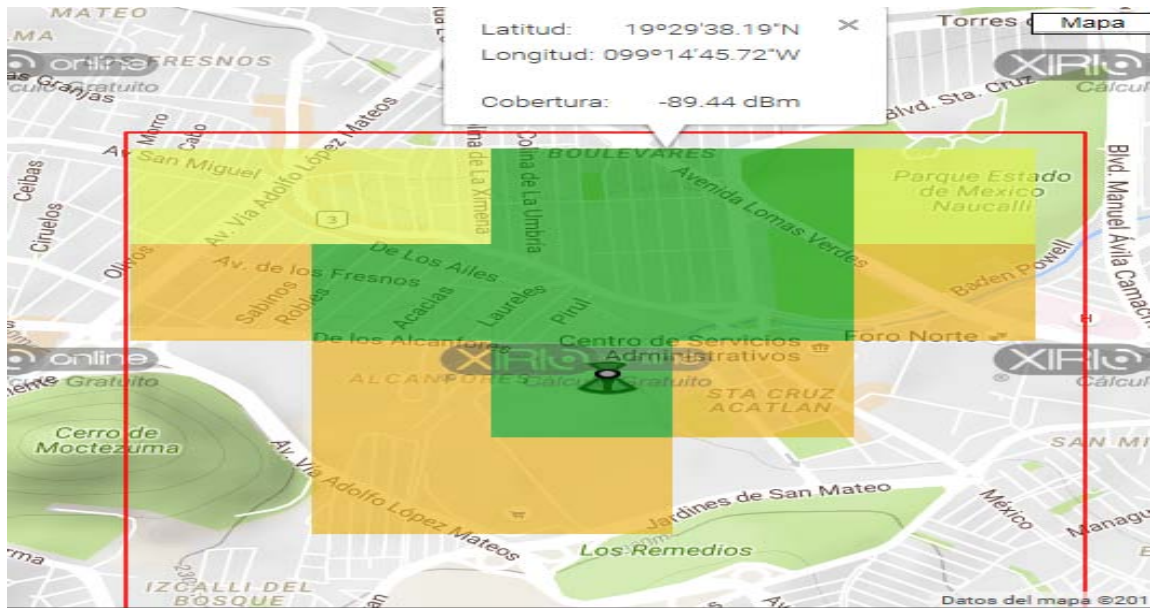
Figura 7.54 Diagrama de cobertura y valor en un punto (Área Verde).
