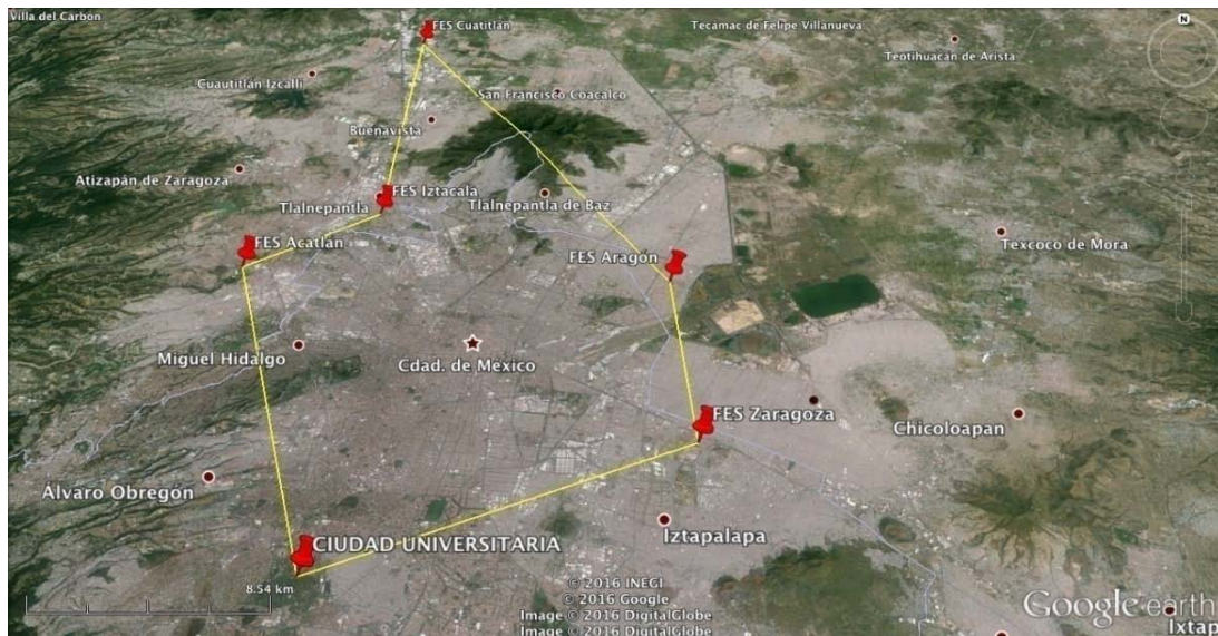
Figura 7.8 Diseño de enlace en forma de anillo.
