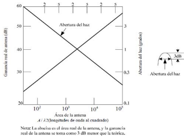
Figura 7.23 Relación entre la ganancia de potencia y la abertura del haz de una antena.
