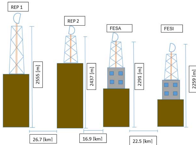
Figura 7.28 Vista General Enlaces Repetidor 1.
