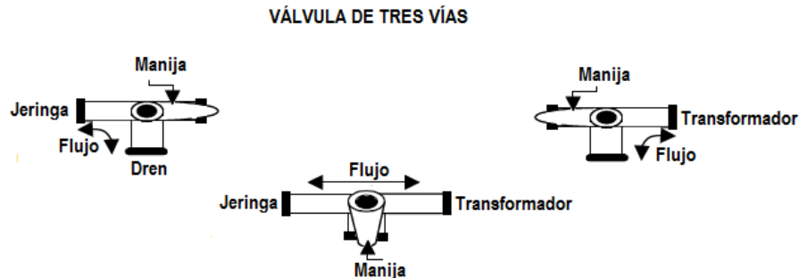
Figura 3.1.- Esquema del funcionamiento de la conexión jeringa–válvula – transformador.
