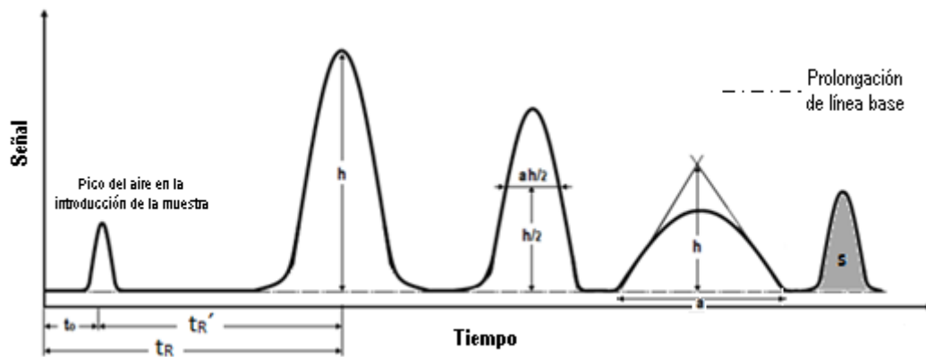
Figura 2.2.- Cromatograma típico.
