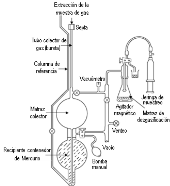
Figura 3.3.- Esquema de equipo de desgasificación.
