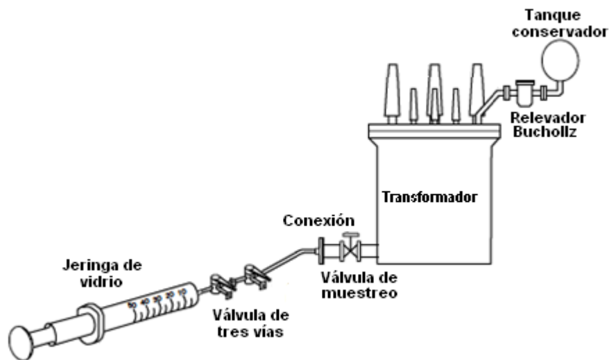
Figura 3.2.- Esquema de conexión jeringa–válvula –transformador.
