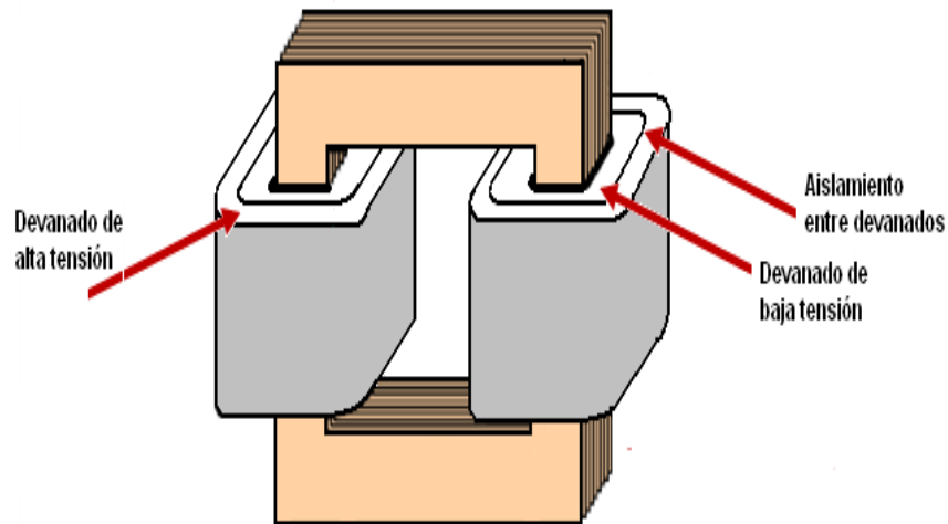
Figura 1.3.- Núcleo tipo columna ó Core.
