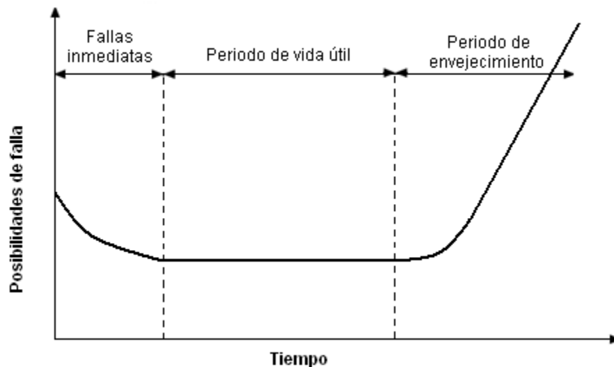
Figura 1.5.- Curva de vida-muerte típica de un Transformador.
