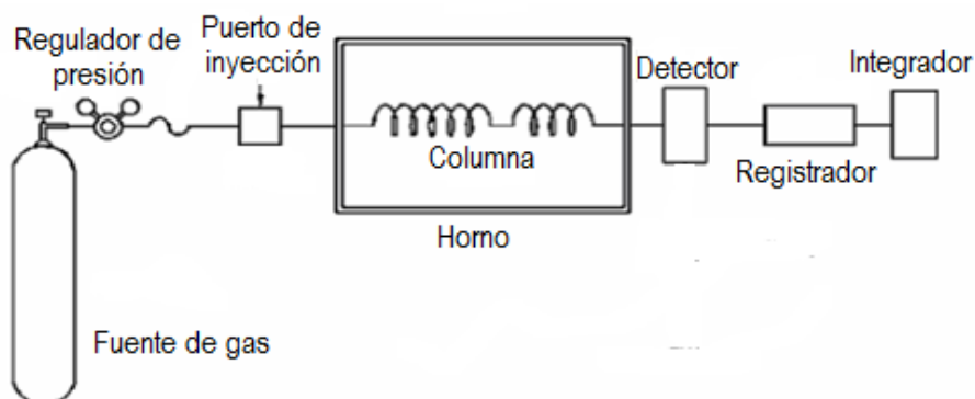
Figura 2.1.- Principales componentes de un cromatógrafo de gases.
