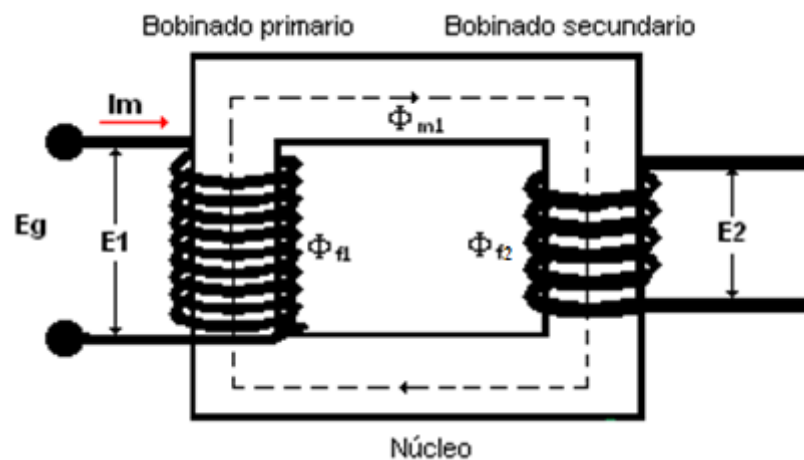
Figura 1.1.- Núcleo y devanados de un Transformador.
