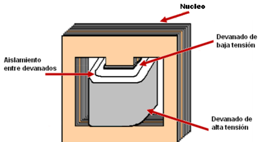
Figura 1.2.- Núcleo tipo acorazado ó Shell.
