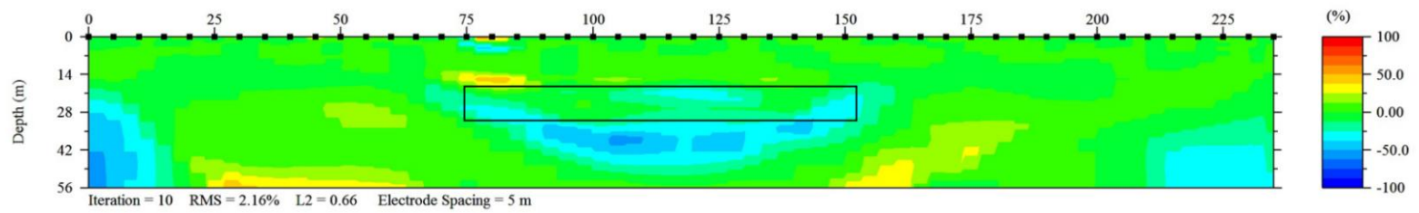
Figura 13. Arreglo Dipolo-Dipolo. Cuerpo en un semiespacio. Porcentaje de diferencia entre los datos de resistividad del caso ideal y los datos multiplicados por el factor de corrección.
