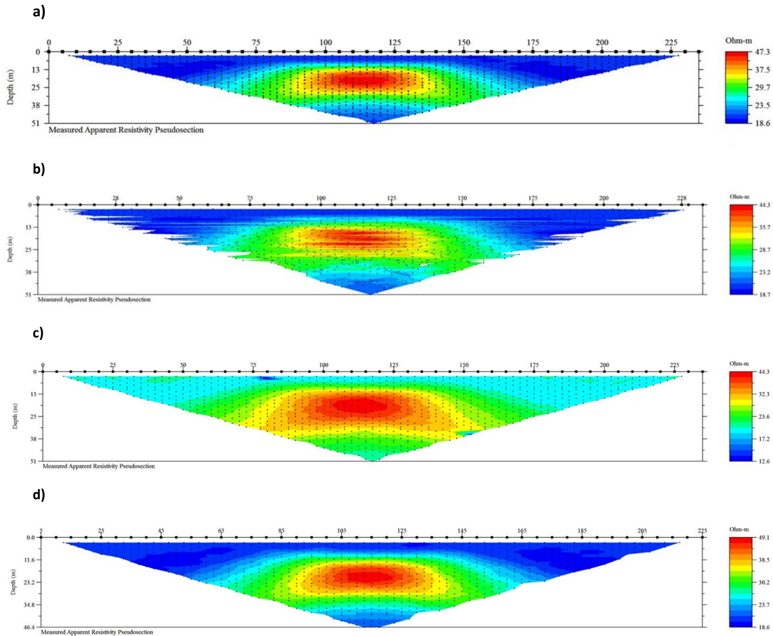
Figura 11. Arreglo Dipolo-Dipolo. Pseudosecciones de resistividad aparente medida. Cuerpo en un semiespacio. a) Caso ideal b) 50% de error aleatorio en la posición electrónica c) Aplicación de factor geométrico de corrección d) Interpolación de datos.
