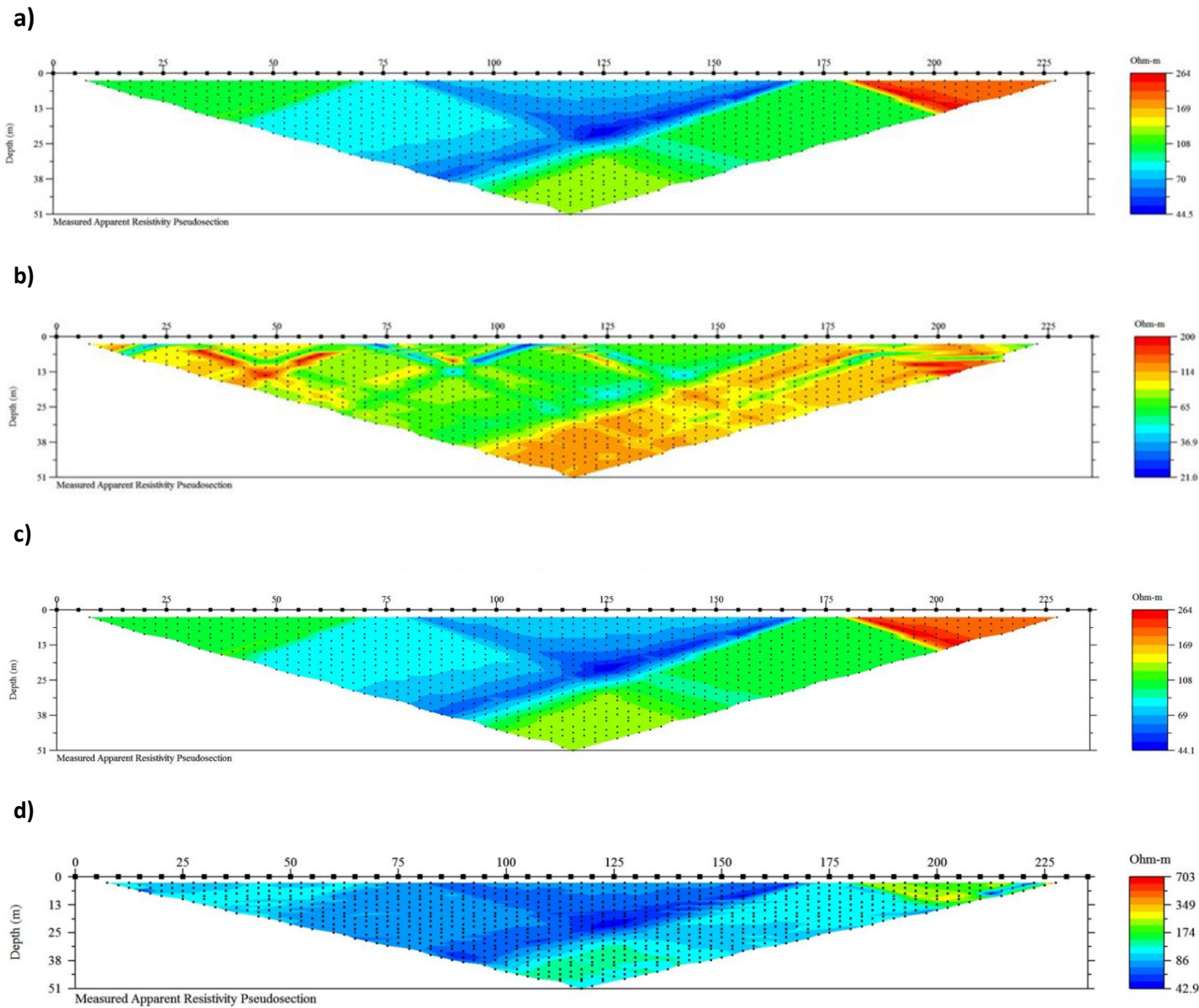
Figura 15. Arreglo Dipolo-Dipolo. Pseudosecciones de resistividad aparente medida. Contacto vertical. a) Caso ideal b) 50% de error aleatorio en la posición eléctrica c) Aplicación de factor geométrico de corrección d) Interpolación de datos.
