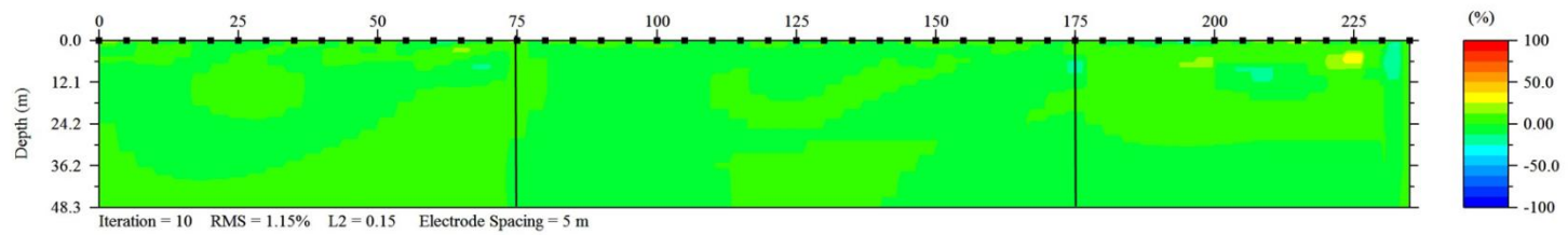
Figura 33. Arreglo Schlumberger. Contacto vertical. Porcentaje de diferencia entre los datos de resistividad del caso ideal y los datos multiplicados por el factor de corrección. La línea continua representa los contactos originales.
