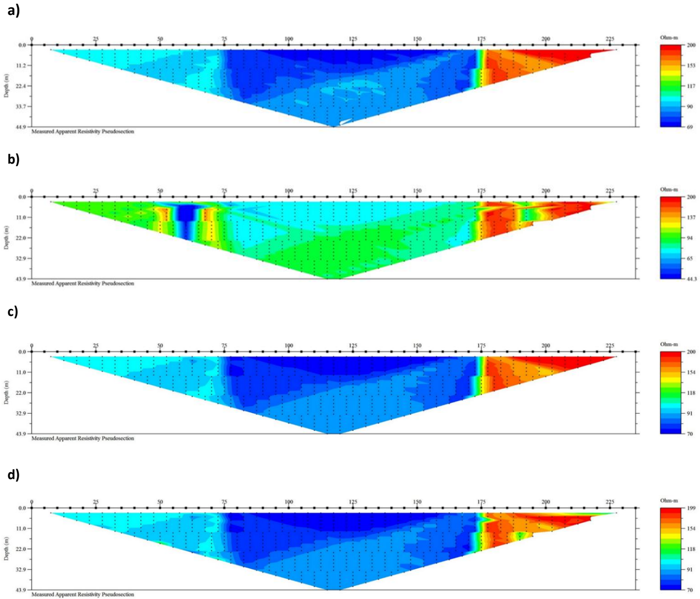
Figura 7. Arreglo Schlumberger. Pseudosecciones de resistividad aparente medida. Contacto vertical. a) Caso ideal b) 50% de error aleatorio en la posición electródica c) Aplicación de factor geométrico de corrección d) Interpolación de datos.
