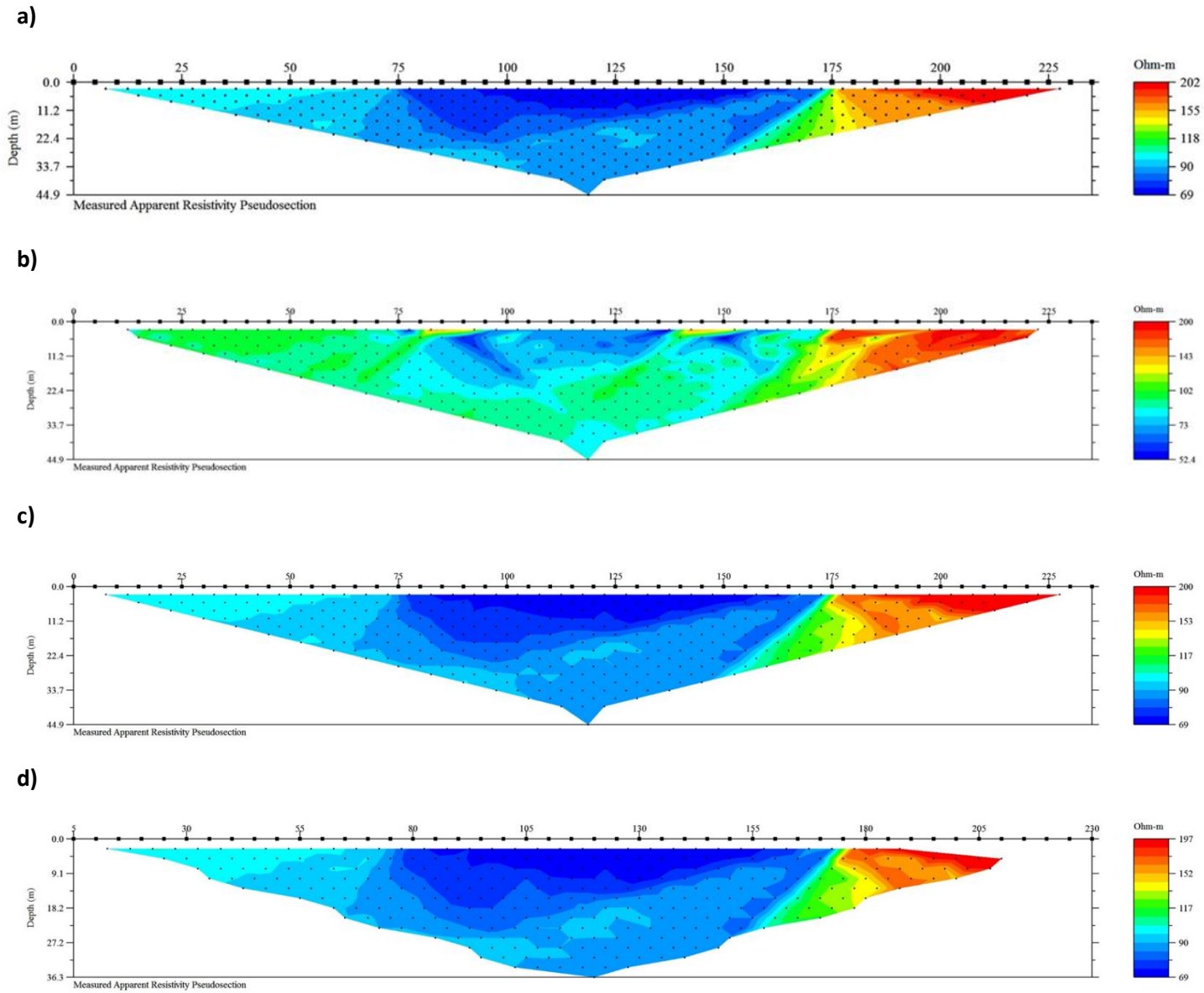
Figura 23 Arreglo Wenner. Pseudosecciones de resistividad aparente medida. Contacto vertical. a) Caso ideal b) 50% de error aleatorio en la posición electrónica c) Aplicación de factor geométrico de corrección d) Interpolación de datos.
