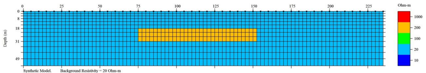
Figura 9. Modelo sintético, cuerpo en un semiespacio.
