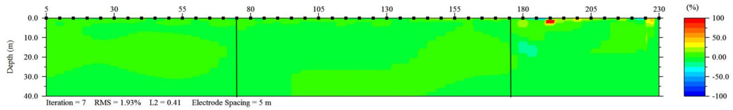
Figura 26. Arreglo Wenner. Contacto vertical. Porcentaje de diferencia entre los datos de resistividad del caso ideal y los datos interpolados. La línea continua representa los contactos originales. La línea continua representa los contactos originales.
