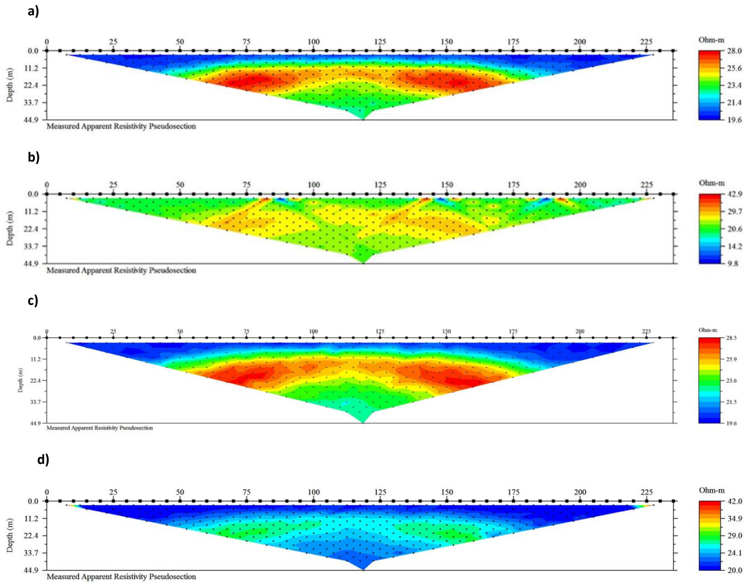
Figura 19. Arreglo Wenner. Pseudosecciones de resistividad aparente medida. Cuerpo en un semiespacio. a) Caso ideal b) 50% de error aleatorio en la posición electrónica c) Aplicación de factor geométrico de corrección d) Interpolación de datos.
