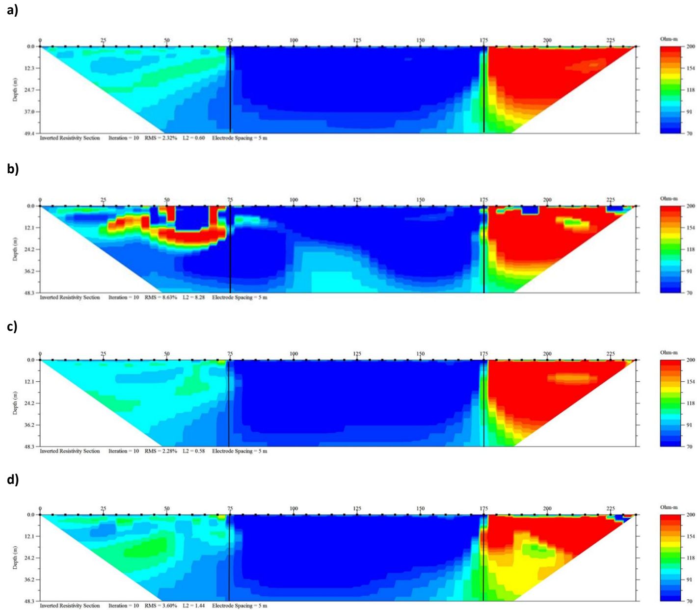
Figura 32. Arreglo Schlumberger. Secciones de resistividad invertida. Contacto vertical. a) Caso ideal b) 50% de error aleatorio en la posición electrodica c) Aplicación de factor geométrico de corrección d) Interpolación de datos. La línea continua representa los contactos originales.
