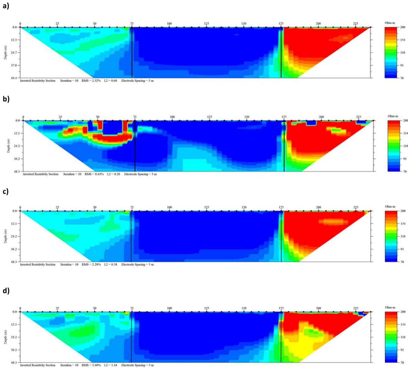
Figura 8. Arreglo Schlumberger. Secciones de resistividad invertida. Contacto vertical. a) Caso ideal b) 50% de error aleatorio en la posición electródica c) Aplicación de factor geométrico de corrección d) Interpolación de datos. La línea continua representa los contactos originales.
