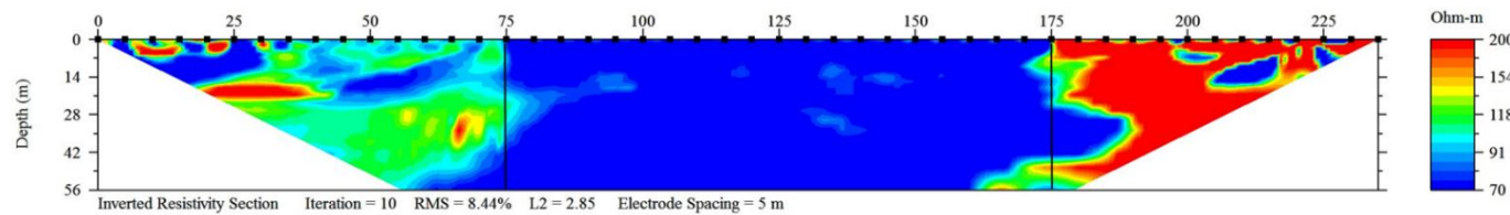
Figura 16. Arreglo Dipolo-Dipolo. Secciones de resistividad invertida. Contacto vertical. a) Caso ideal b) 50% de error aleatorio en la posición electrodica c) Aplicación de factor geométrico de corrección d) Interpolación de datos. La línea continua representa los contactos originales.
