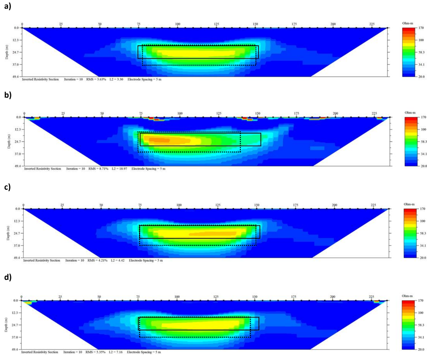
Figura 20. Arreglo Wenner. Secciones de resistividad invertida. Cuerpo en un semiespacio. a) Caso ideal b) 50% de error aleatorio en la posición electródica c) Aplicación de factor geométrico de corrección d) Interpolación de datos. La línea continua representa el cuerpo original, mientras que la línea punteada representa el cuerpo detectado.
