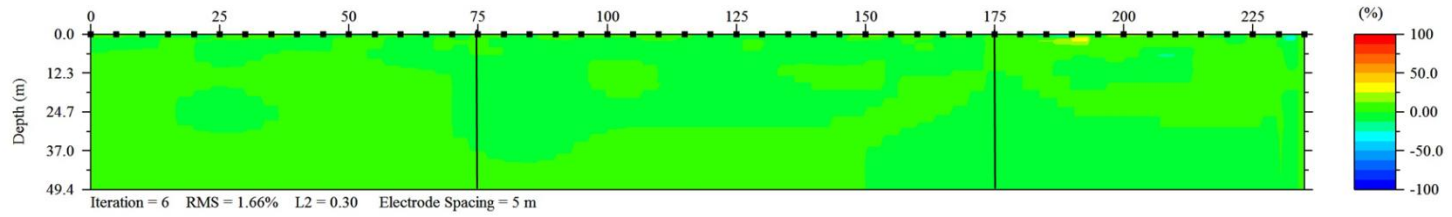
Figura 25. Arreglo Wenner. Contacto vertical. Porcentaje de diferencia entre los datos de resistividad del caso ideal y los datos multiplicados por el factor de corrección. La línea continua representa los contactos originales. La línea continua representa los contactos originales.
