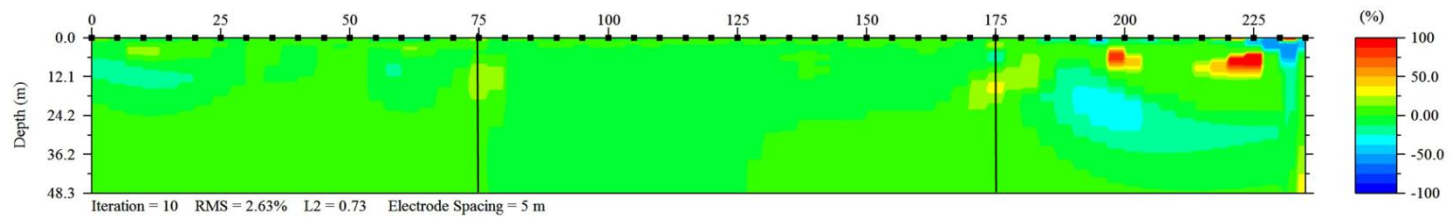
Figura 34. Arreglo Schlumberger. Contacto vertical. Porcentaje de diferencia entre los datos de resistividad del caso ideal y los datos interpolados. La línea continua representa los contactos originales.
