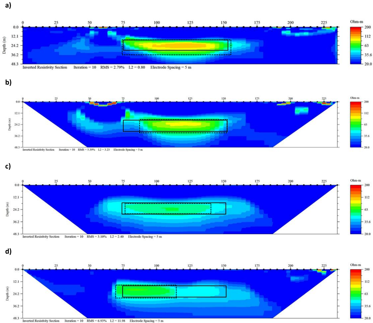
Figura 28 Arreglo Schlumberger. Secciones de resistividad invertida. Cuerpo en un semiespacio. a) Caso ideal b) 50% de error aleatorio en la posición electródica c) Aplicación de factor geométrico de corrección d) Interpolación de datos. La línea continua representa el cuerpo original, mientras que la línea punteada representa el cuerpo detectado.
