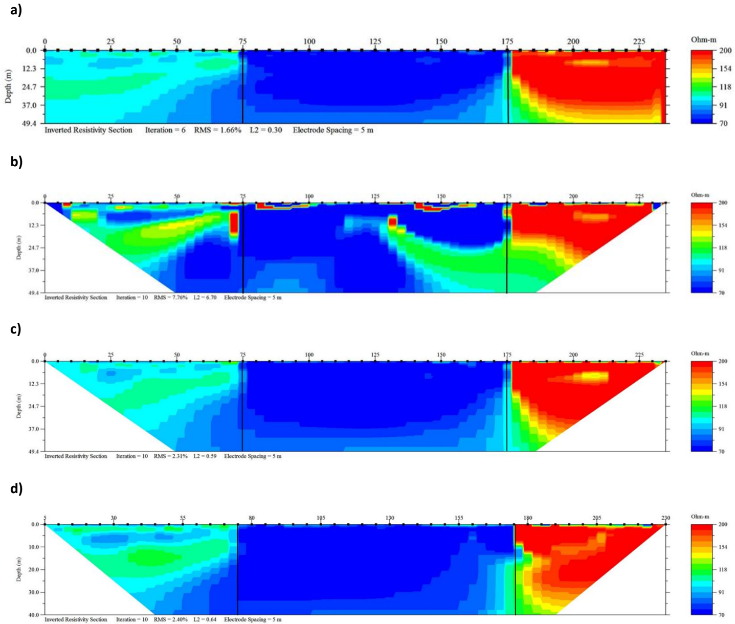
Figura 24. Arreglo Wenner. Secciones de resistividad invertida. Contacto vertical. a) Caso ideal b) 50% de error aleatorio en la posición electrodica c) Aplicación de factor geométrico de corrección d) Interpolación de datos. La línea continua representa los contactos originales.
