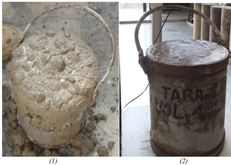
Figura 3.10 Determinación de peso volumétrico de concreto fresco 1. Llenado de recipiente, 2. Mezcla compactada para determinación de su masa.
