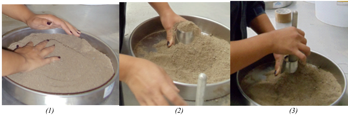
Figura 3.6 Determinación de estado sss para AF 1. Secado de material, 2. Llenado de cono truncado, 3. Compactación de arena.
