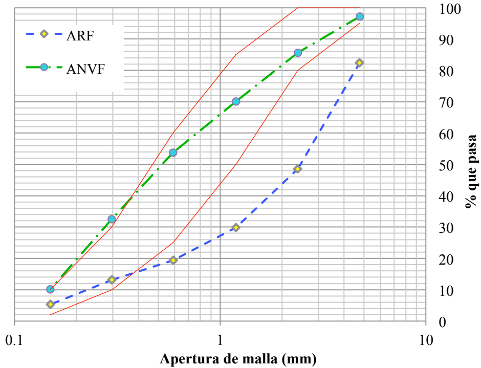
Figura 4.2 Curvas granulométricas de agregados finos Fuente: Elaboración propia
