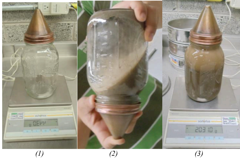
Figura 3.7 Determinación de densidad para AF
