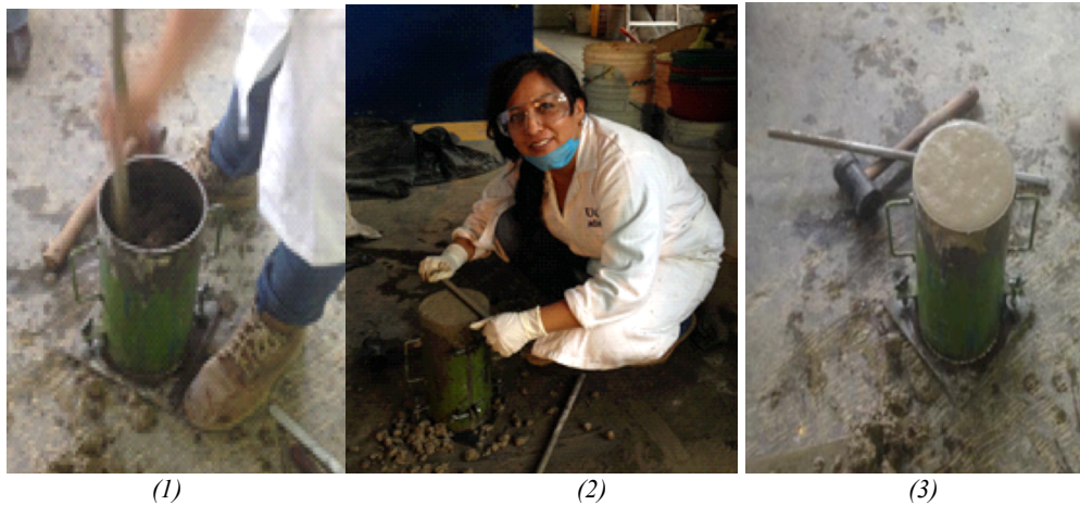
Figura 3.12 Elaboración de especímenes 1. Llenado y compactado de mezcla, 2. Enrase de molde, 3. Cilindro terminado.
