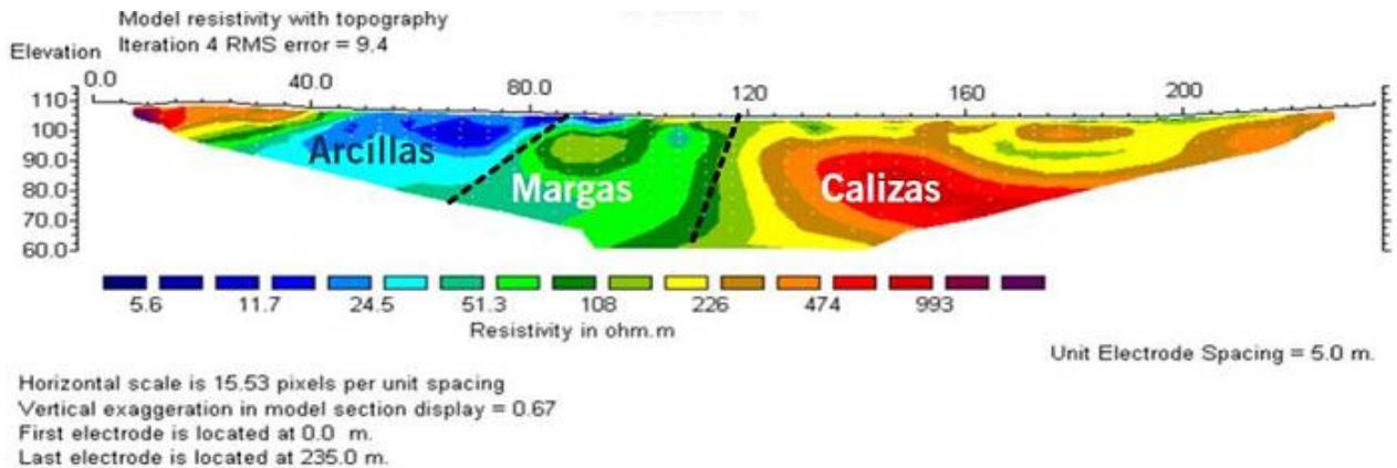
Ilustración 2.-Caso práctico de Tomografía Eléctrica (tomado de Wide World, presentación en Power Point "Prospección Geofísica mediante Tomografía Eléctrica").
