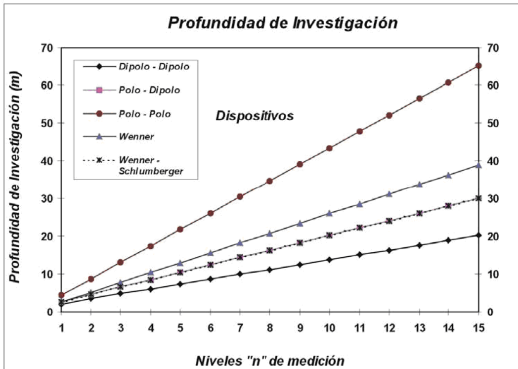
Gráfico. Profundidades medias de investigación sobre un medio homogéneo de resistividad para los dispositivos Dipolo-Dipolo, Polo-Dipolo, Wenner y Wenner –Schlumberger obtenidas para una distancia interelectródica de 5 metros y distintos niveles (Loke, 2002).
