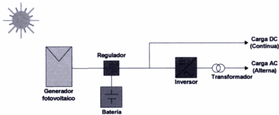
Figura 15. Componentes de un Sistema Fotovoltaico. Fuente: MENDEZ Muñiz, Javier María. CUERVO García, Rafael. Energía solar fotovoltaica. 2da Edición. ECA, Instituto de Tecnología y Formación. Madrid, España. FC Editorial.
