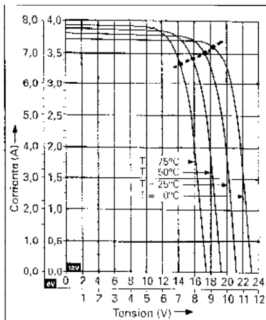
Figura 16. Relación entre corriente y voltaje de salida para un panel fotovoltaico.
