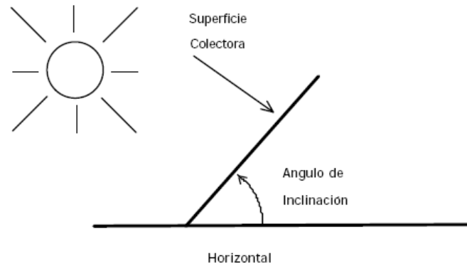
Figura 17. Ángulo de inclinación de los paneles fotovoltaicos. Fuente: L. Gasquet, Héctor. Conversión de la luz solar en energía eléctrica: Manual teórico y práctico sobre los sistemas fotovoltaicos. El Paso, Texas, El Paso Solar Energy, 2004.
