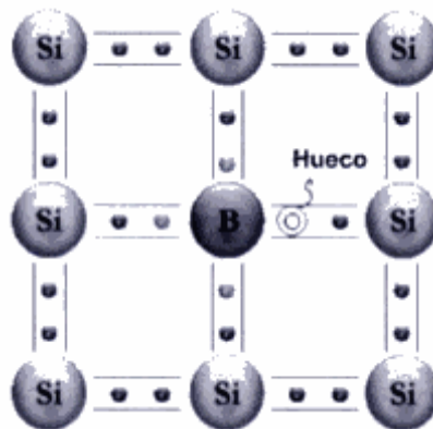
Figura 9. Hueco libre en Red Cristalina. Fuente: MENDEZ Muñiz, Javier María. CUERVO García, Rafael. Energía solar fotovoltaica. 2da Edición. ECA, Instituto de Tecnología y Formación. Madrid, España. FC Editorial.
