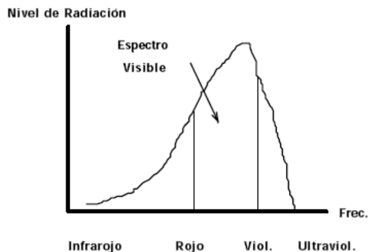
Figura 3. Composición del Espectro Luminoso. Fuente: L. Gasquet, Héctor. Conversión de la luz solar en energía eléctrica: Manual teórico y práctico sobre los sistemas fotovoltaicos. El Paso, Texas, El Paso Solar Energy, 2004
