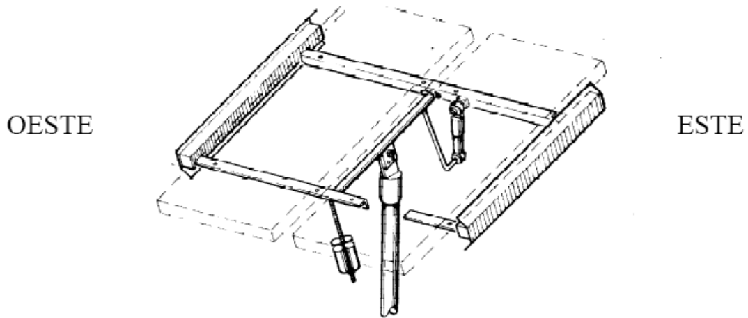
Figura 19. Seguidor de un eje. Fuente: L. Gasquet, Héctor. Conversión de la luz solar en energía eléctrica: Manual teórico y práctico sobre los sistemas fotovoltaicos. El Paso, Texas, El Paso Solar Energy, 2004.
