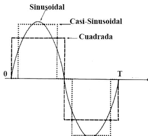
Figura 19. Formas de onda de salida de un inversor. Fuente: L. Gasquet, Héctor. Conversión de la luz solar en energía eléctrica: Manual teórico y práctico sobre los sistemas fotovoltaicos. El Paso, Texas, El Paso Solar Energy, 2004.
