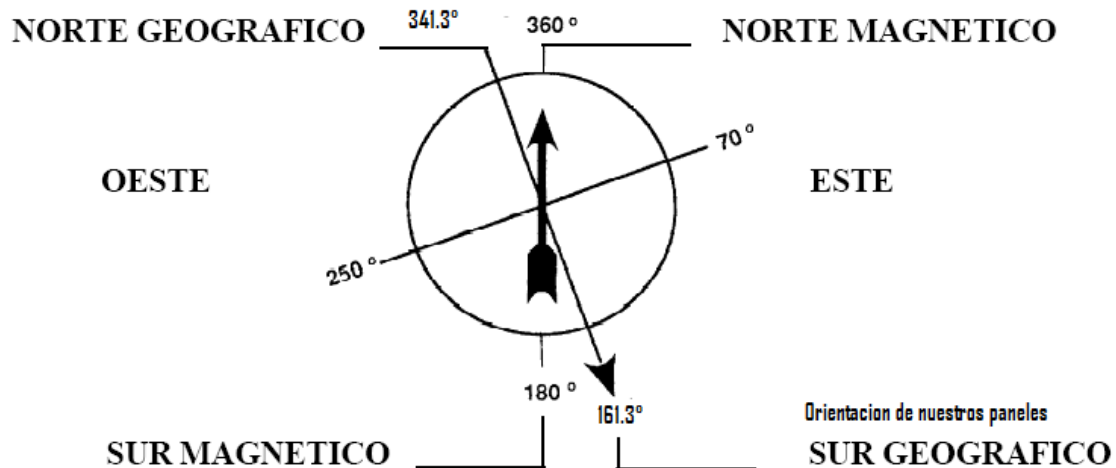
Figura 18. Orientación geográfica de los paneles fotovoltaicos. Fuente: L. Gasquet, Héctor. Conversión de la luz solar en energía eléctrica: Manual teórico y práctico sobre los sistemas fotovoltaicos. El Paso, Texas, El Paso Solar Energy, 2004.
