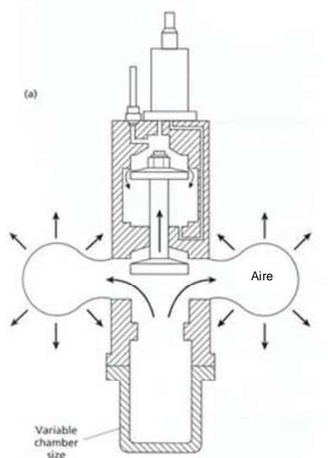
Figura 3.9. Cañon de aire (air gun) empleado en la sísmica de reflexión para generar un frente de ondas acústicas (Tomada de Kearey, Brooks, and Hill, 2002., en Chris Liner.ppt).
