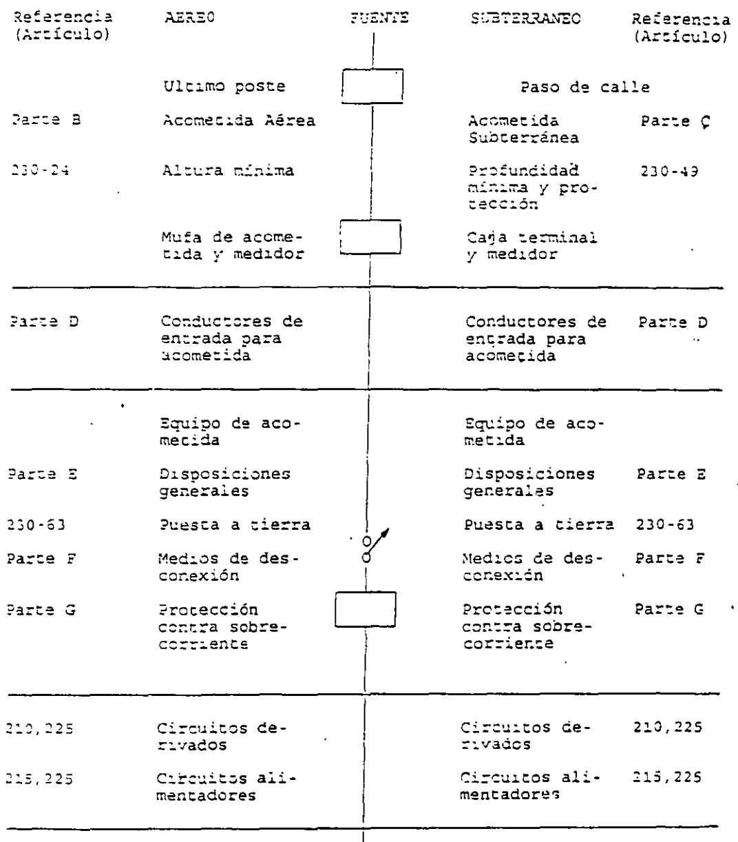
Diagrama 230-1 Acometidas
