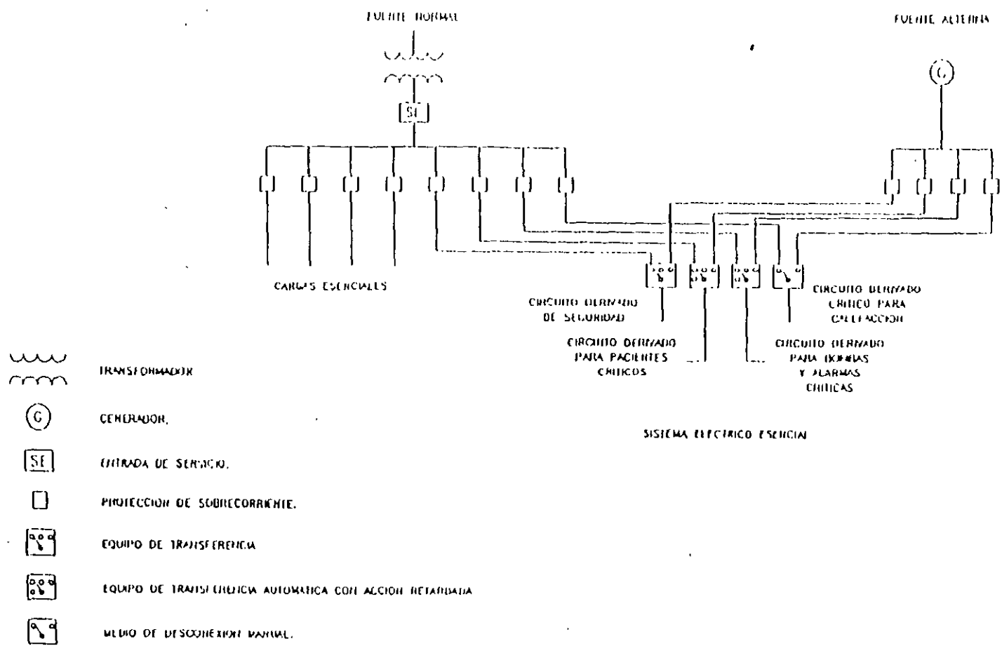
DIAGRAMA 517-41(2)
