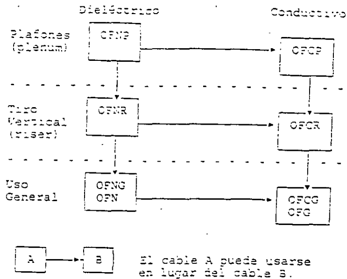
Figura 770-53 Jerarquía de sustitución de cables
