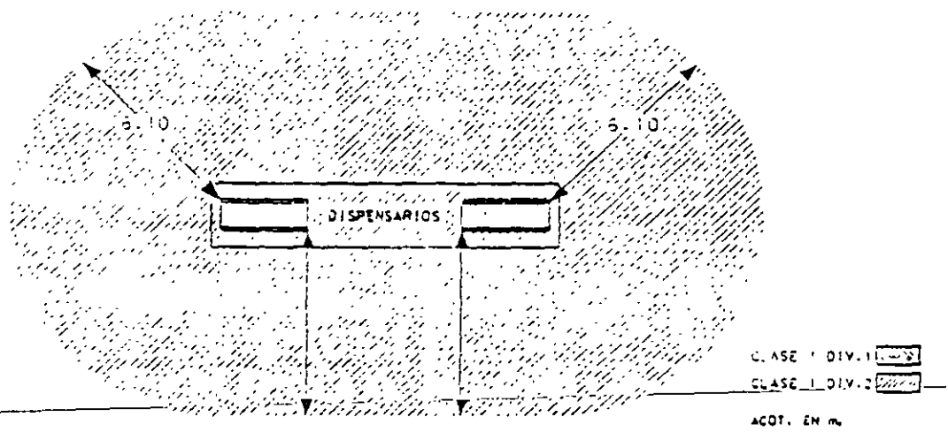
FIGURA 1.- LUGARES CLASIFICADOS ADYACENTES A LOS SURTIADORES & DISPENSARIOS COMO SE DETALLA EN LA TABLA 514-2.
