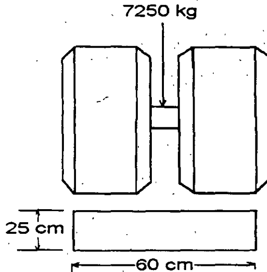
a)Área de carga de una rueda
