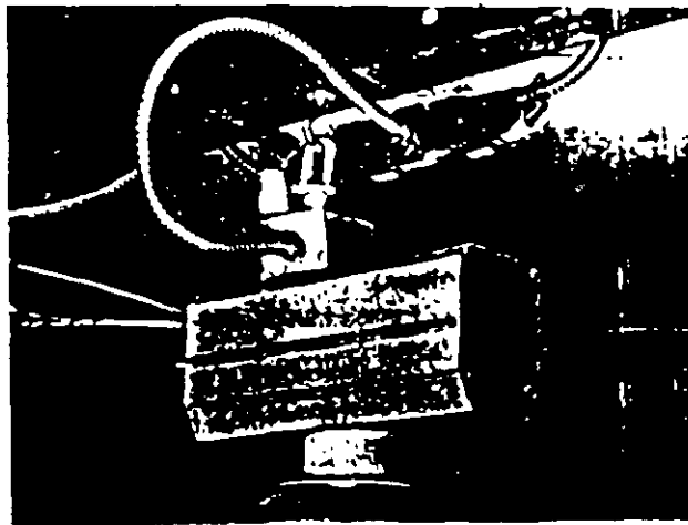
EJEMPLO DE CABLE CON CUBIERTA METALICA DE NO MAS DE 1.83 m DE LARGO, CONTENIENDO CONDUCTORES DE 12 AWG O MENORES PERMITIDO POR LA EXCEPCION 1.
