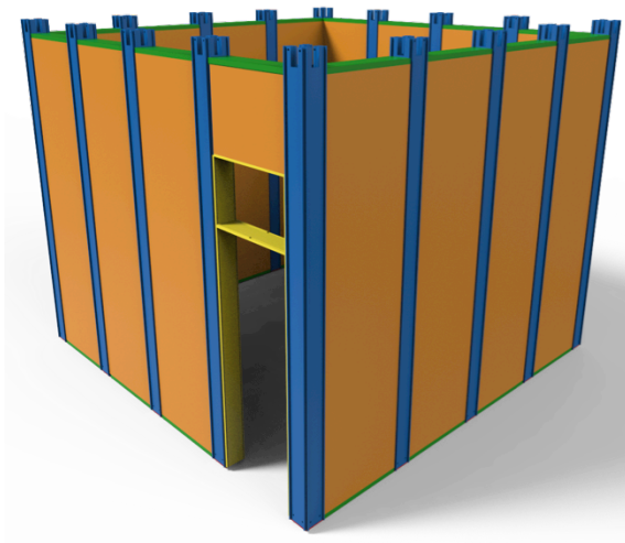
Fig. 18. Instalación de Rigidizadores superiores.
