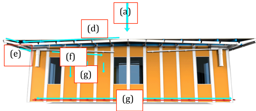
Fig. 7. Manejo de agua en una vivienda fabricada con el Sistema constructivo propuesto pasos (e) al (g).
