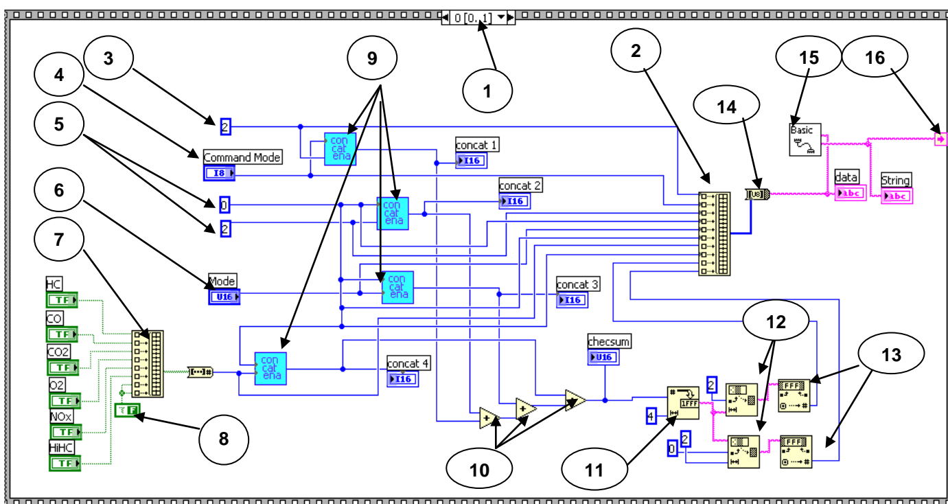
Figura VI.3. Instrumento Virtual Calibración (solicitud).
