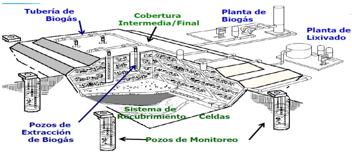
Figura 3.4: Componentes de un relleno sanitario moderno con quema de biogás. Fuente: (EPA, 2015).
