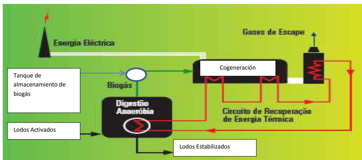
Figura 3.6: Esquema de instalación del sistema de generación de electricidad a partir del biogás en las plantas de tratamiento de aguas residuales. Fuente: (Limón Macías, 2013)
