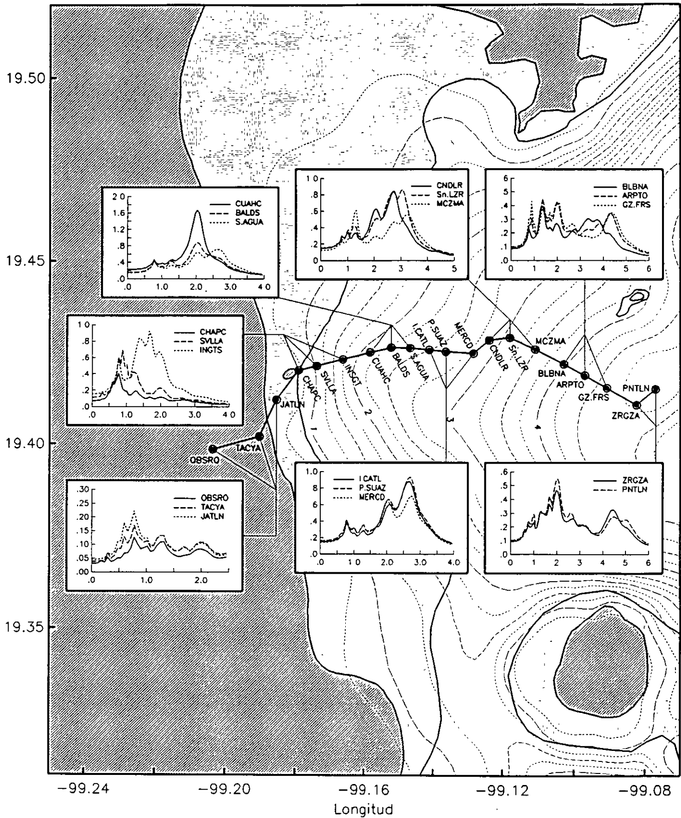
Figura 9. Espectros de respuesta para las estaciones de la Línea 1 del Sistema de Transporte Colectivo de la Ciudad de México. Se indican algunas curvas de isoperiodos dominantes del Terreno como referencia adicional.
