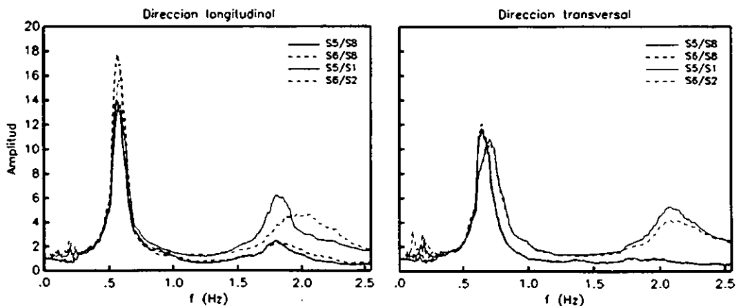
Figura 6 Funciones de trasferencia de azoteas relativas a: a) campo libre (líneas gruesas) y b) sótanos (líneas gruesas)
