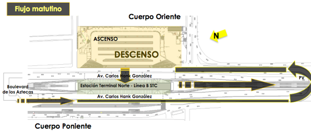
Figura 4.5 Flujo matutino durante la segunda etapa de construcción.
