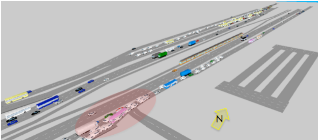
Figura 4.4 Imagen de la simulación de la situación esperada durante el proceso de construcción de la ETRAM. En rojo, problemas viales sobre la lateral.
