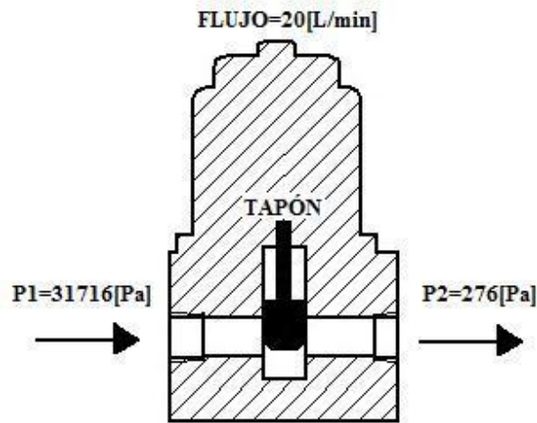
1.4 Flujo de gas dentro de la válvula proporcional.
