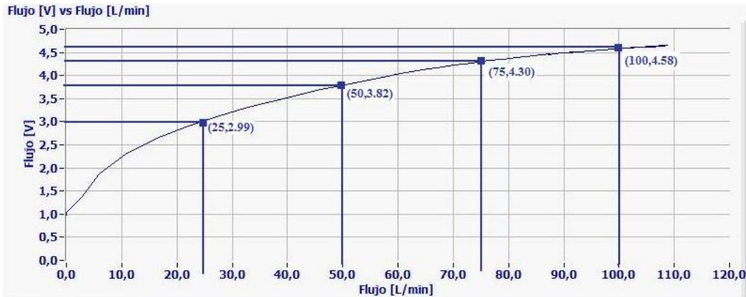
Figura 1.1. Validación del sensor de flujo.
