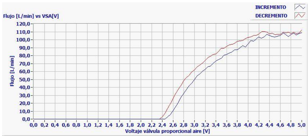
1.2. Flujo vs Voltaje válvula proporcional de aire.
