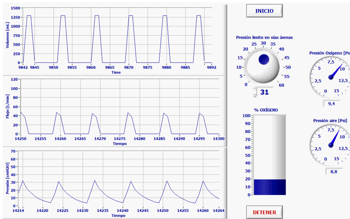
Figura 1.5. Validación del sensor de presión en vías áereas.
