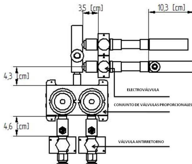
Figura 1.3 Circuito neumático sobre el cual se hará un análisis matemático de pérdidas de presión.
