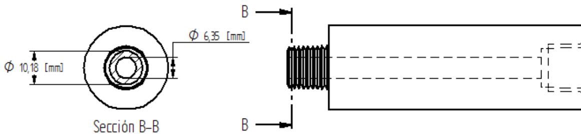
Figura 1.5 Vista a detalle del conector de entrada de gases.
