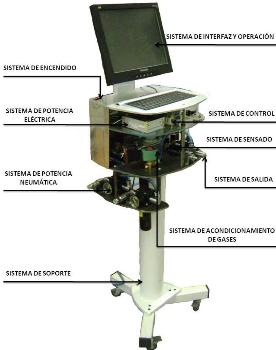
Figura 1.1 Ensamble general.
