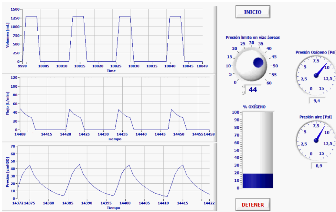
Figura 1.6. Validación del sensor de presión de vías áereas.
