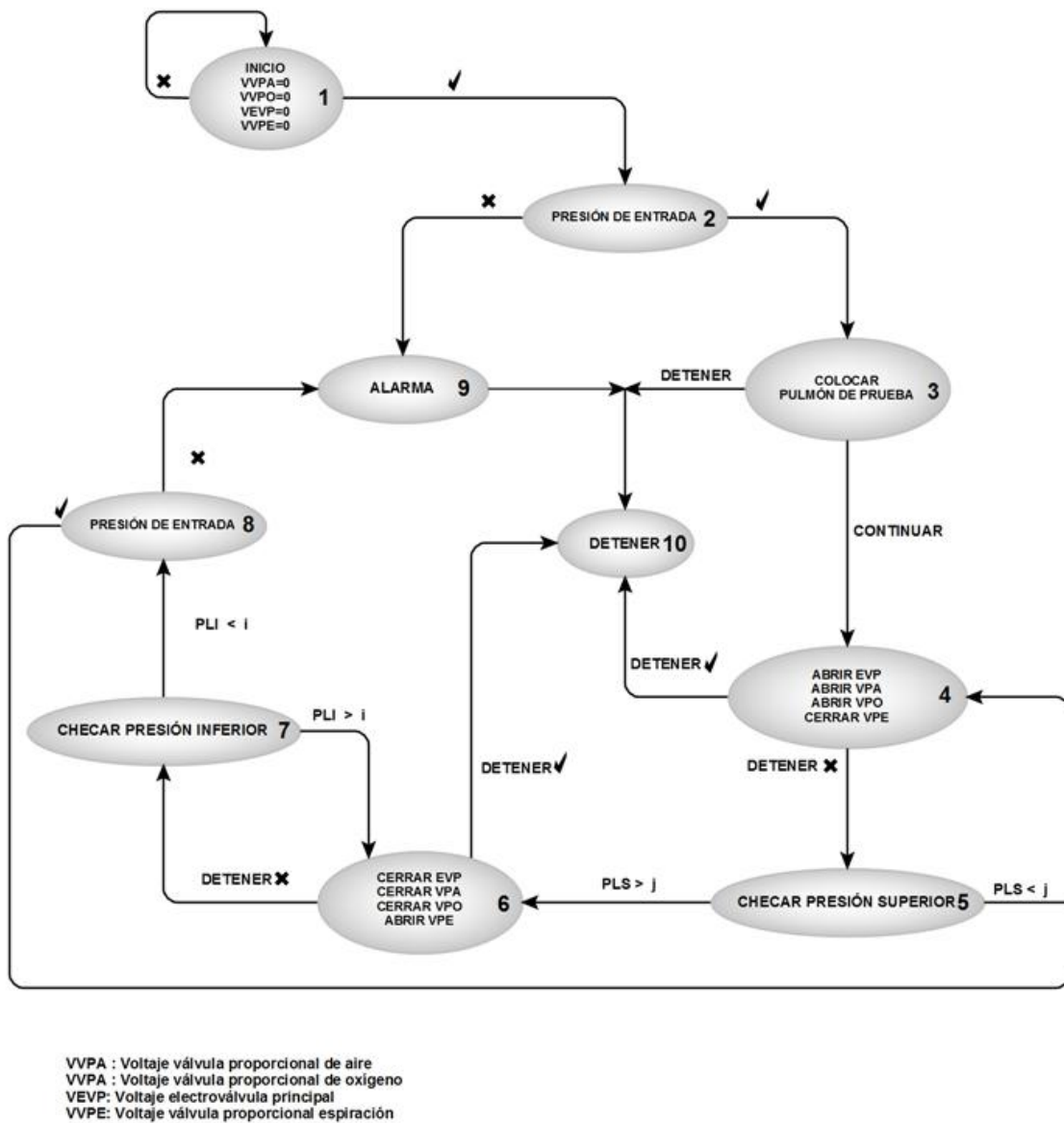
Diagrama 1.3 Máquina de estados para la prueba de “Inicialización sensor de presión de las vías aéreas”.
