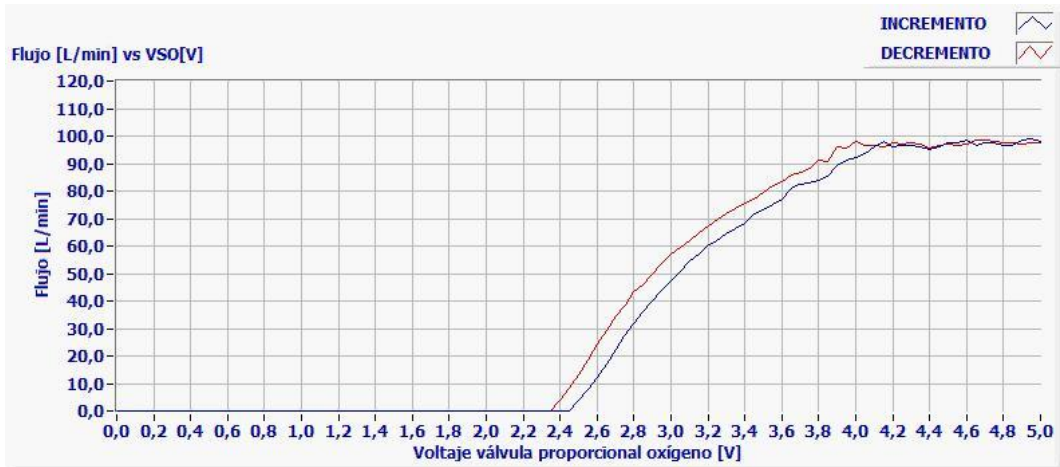
Figura 1.3 Flujo vs Voltaje válvula proporcional de oxígeno.
