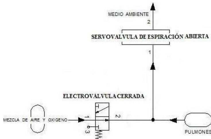
Figura 1.11 Estado de los elementos durante la fase de espiración para la 2º propuesta.
