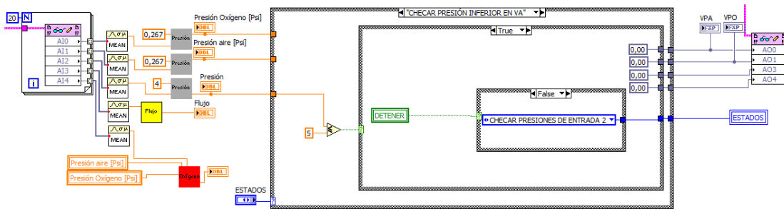
Figura A5.20 Estado 7 de la prueba de validación del sensor de presión en vías aéreas.
