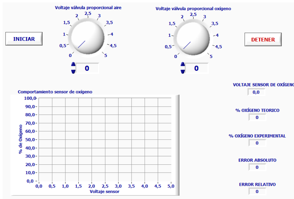
Figura 1.9 Interfaz para validación del sensor de oxígeno.
