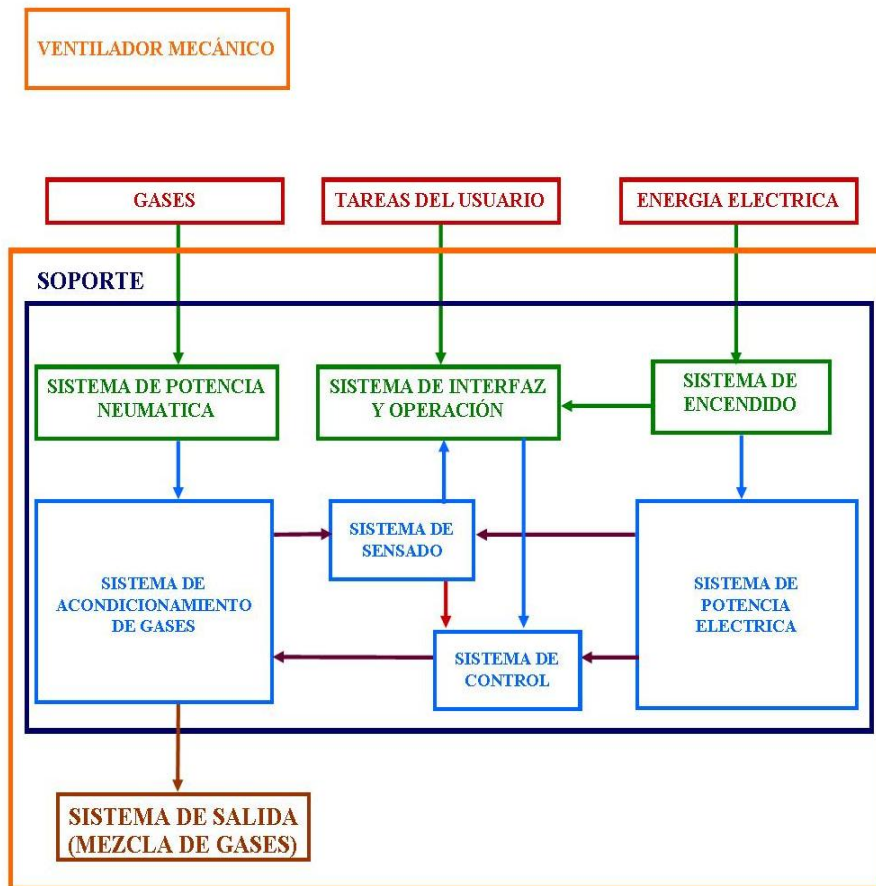
Figura 1.2 Conexión entre sistemas involucrados en la ventilación mecánica.
