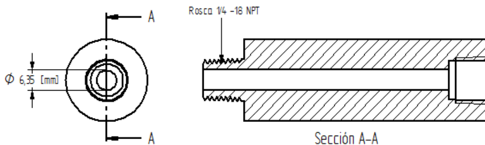
Figura 1. 4 Vista lateral del conector para entrada de gases.
