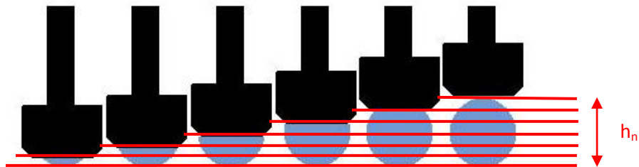
Figura 1.4. Variación del área transversal de la sección por donde pasa el fluido dentro de la válvula proporcional.
