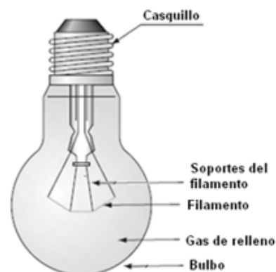
Figura 1.12 Elementos de una lámpara incandescente.
