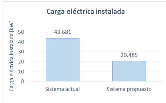
Gráfico 4.7 Reducción en la carga instalada de iluminación y aire acondicionado.
