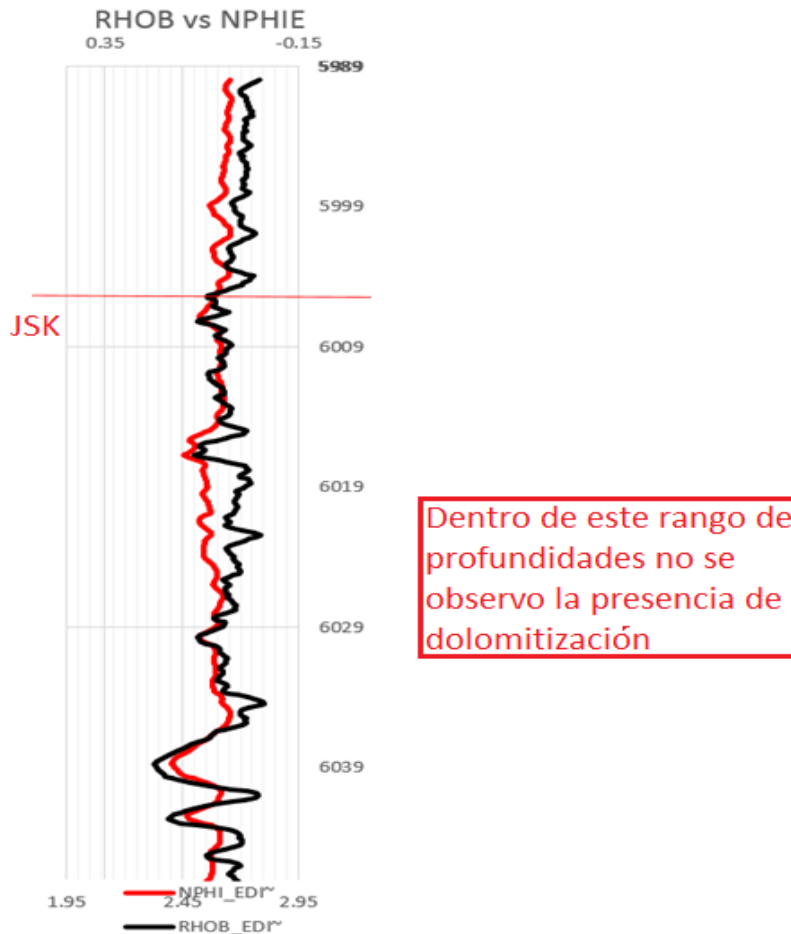
Figura 96.- Integración de datos: registro geofísico curvas (RHOB vs NPHIE); ya que dentro del rango del registro graficado no se encontró dolomitización nos apoyamos en muestras de canal (desafortunadamente no se tienen fotos del informe petrográfico).
