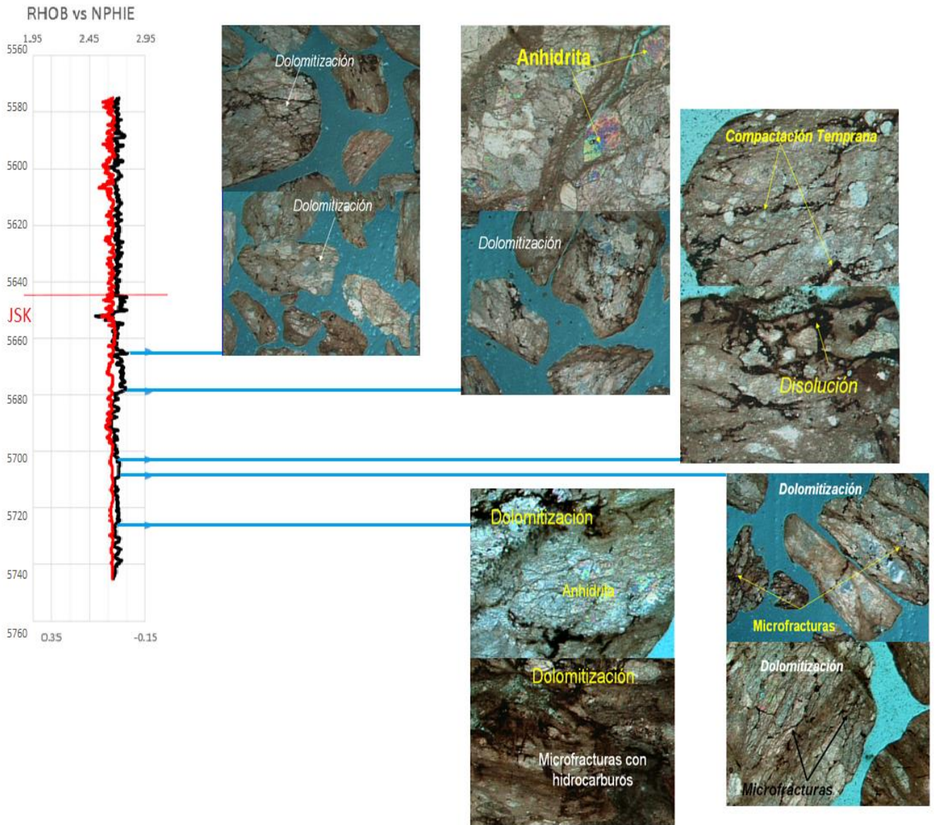
Figura 104.- Integración de datos: registro geofísico curvas (RHOB vs NPHIE) contra muestras de canal, observándose intervalos dolomitizados.
