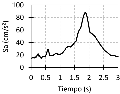
Fig. II.63. Espectro de respuesta ID 34 SCT101294 EW.
