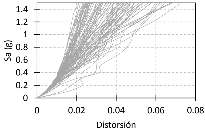
Fig. 2.3. Curva IDA.
