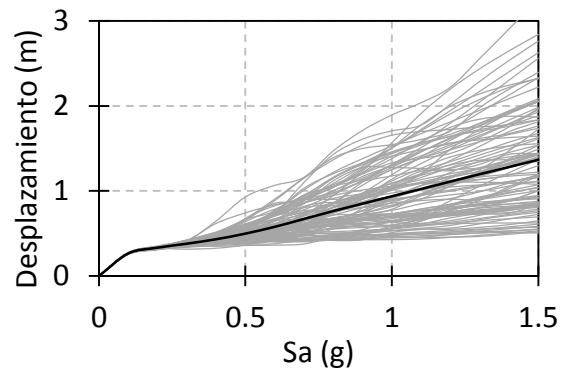
Fig. 4.2. Media geométrica de la curvas IDA Desplazamiento vs Sa, con asentamiento de 10 cm, para el marco de 15 niveles.
