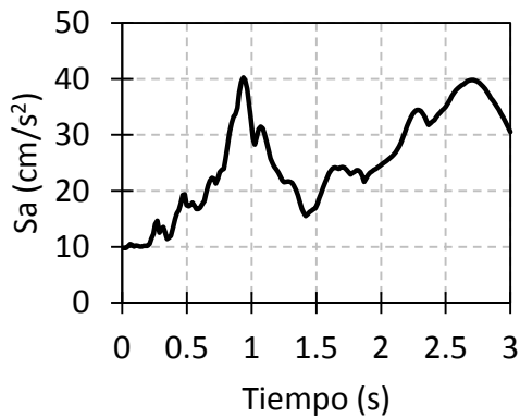
Fig. II.95. Espectro de respuesta ID 24 XP241093 EW.
