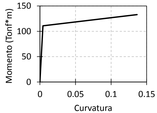
Fig. I.61. Curva Momento-Curvatura para la viga V49i del marco de 25 niveles.
