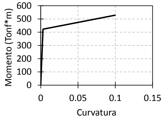
Fig. I.71. Curva Momento-Curvatura para la viga V17i del marco de 25 niveles.
