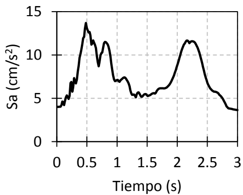
Fig. II.53. Espectro de respuesta ID 33 ROMBS101294 EW.
