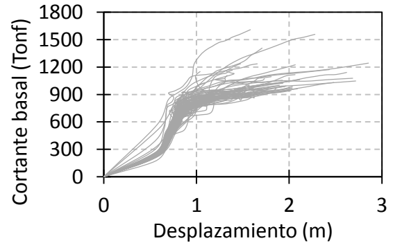
Fig. 3.30. Curvas IDA Cortante basal vs Desplazamiento, con asentamiento de 21 cm, para el marco de 17 niveles.
