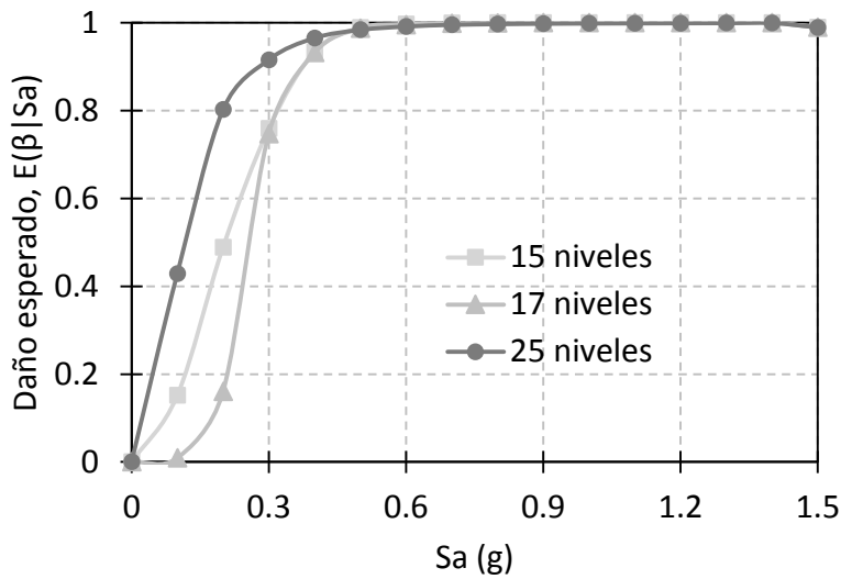
Figura 4.78. Funciones de vulnerabilidad, con asentamiento de 10 cm, para los marcos de 15, 17 y 25 niveles.
