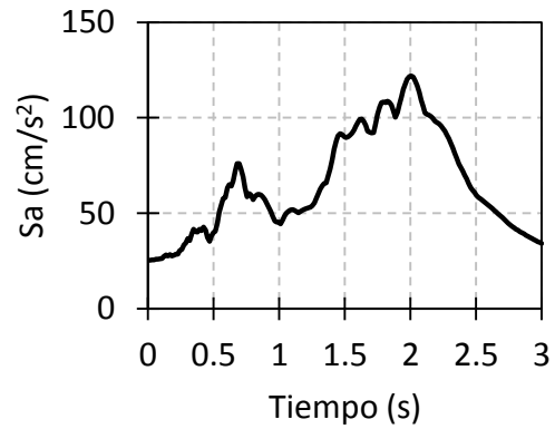
Fig. II.18. Espectro de respuesta ID 39 CJ140995 NS.
