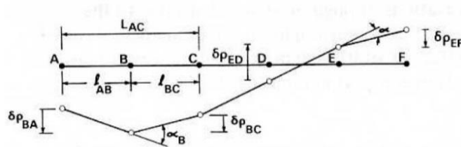
Fig. 1.15. Definición de deformación angular, deflexión relativa y relación de deflexión o parámetro de curvatura. (Burland y Wroth, 1974)
