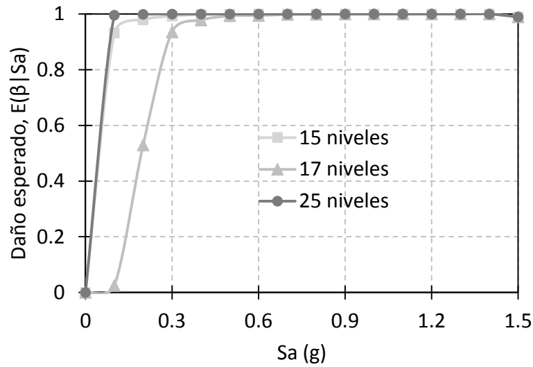
Figura 4.79. Funciones de vulnerabilidad, con asentamiento de 21 cm, para los marcos de 15, 17 y 25 niveles.
