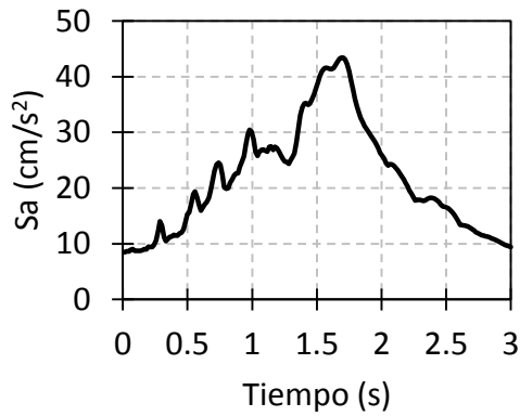
Fig. II.79. Espectro de respuesta ID 21 TL241093 EW.
