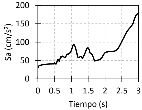
Fig. II.16. Espectro de respuesta ID 4 CA250489 NS.
