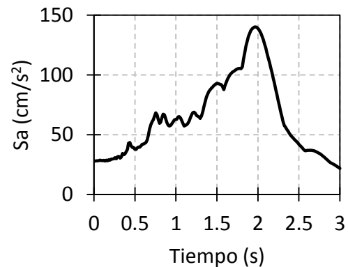
Fig. II.78. Espectro de respuesta ID 49 TL140995_2 NS.
