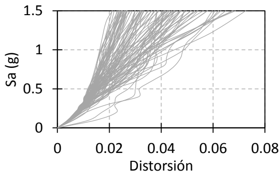
Fig. 3.25. Curvas IDA Sa vs Distorsión, sin asentamiento, para el marco de 17 niveles.
