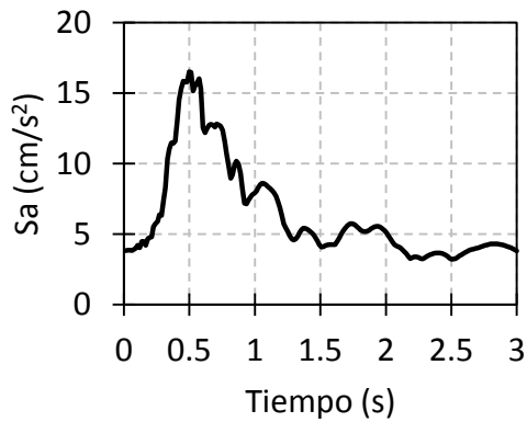
Fig. II.57. Espectro de respuesta ID 18 ROMBS241093 EW.
