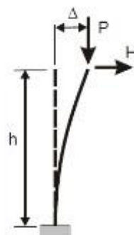
Fig. 1.19. Efecto P-delta en columna
