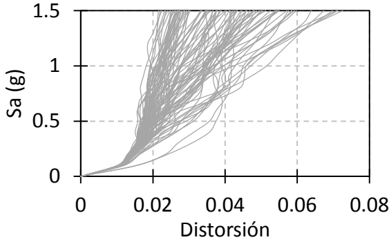
Fig. 3.27. Curvas IDA Sa vs Distorsión con asentamiento de 21cm, para el marco de 17 niveles.
