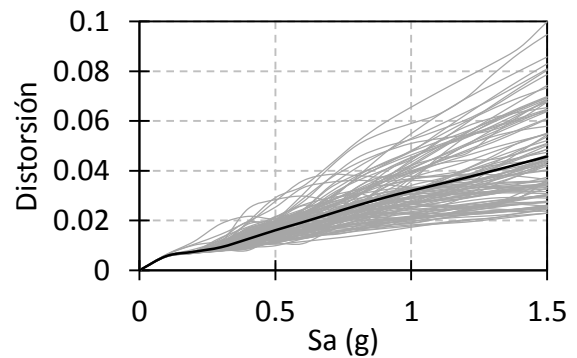
Fig. 4.8. Media geométrica de las curvas IDA Distorsión vs Sa, con asentamiento de 10cm, para el marco de 15 niveles.
