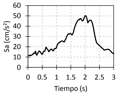
Fig. II.64. Espectro de respuesta ID 34 SCT101294 NS.
