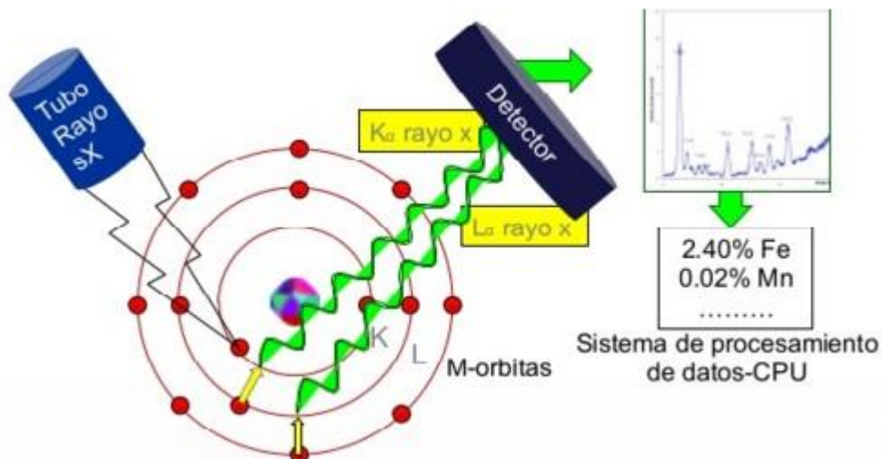
Figura 129. Recuperada de http://es.slideshare.net/OlympusIMS/analizadores-geoquimicos-de-frx , 12 ago. 2014. En la imagen se muestra el tipo de gráfico obtenido a partir del cual se realizan las interpretaciones de una muestra analizada.
