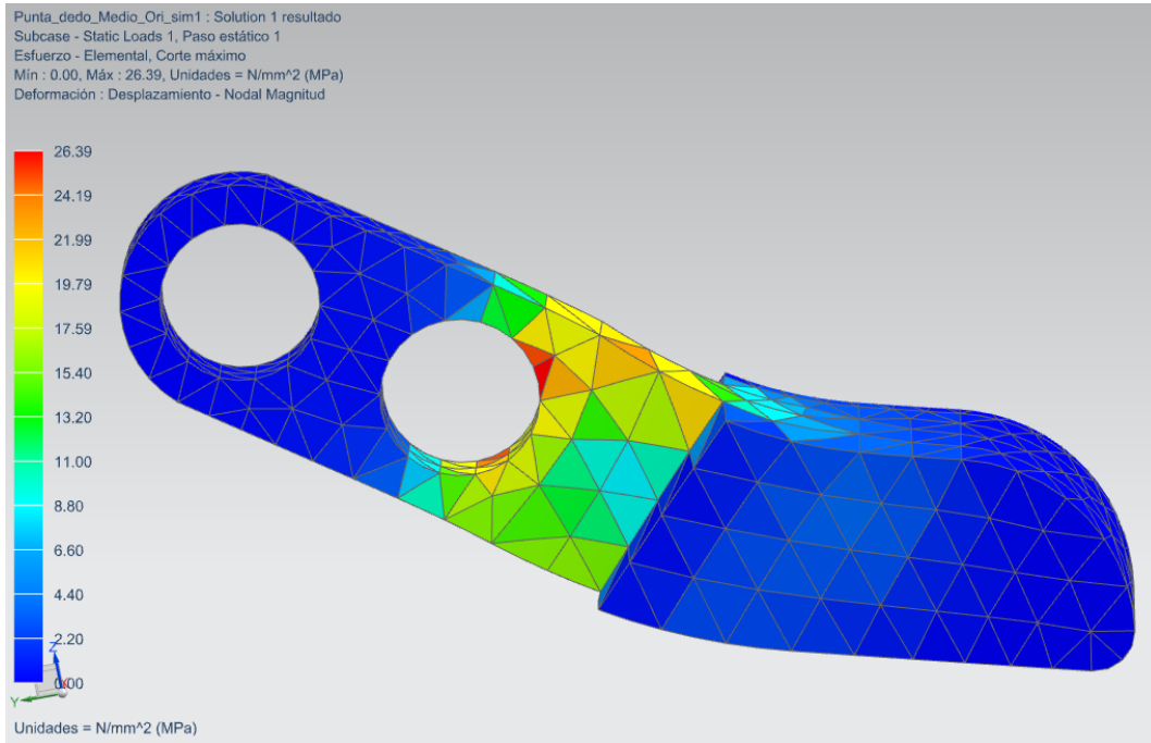
Fig. 46 Esfuerzo de corte máximo NX
