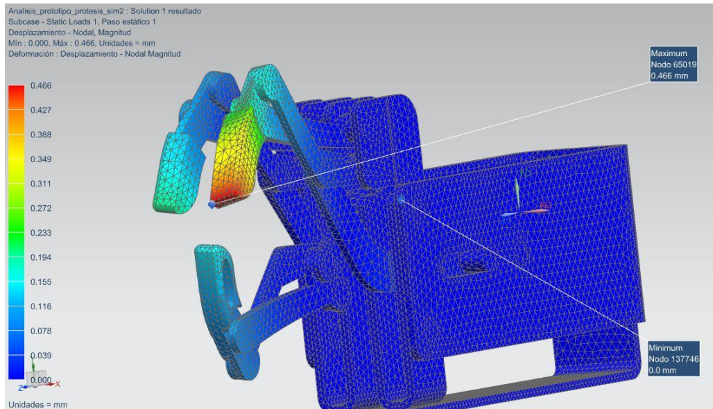
Fig. 51 Análisis desplazamiento del prototipo en NX con carga (completa)
