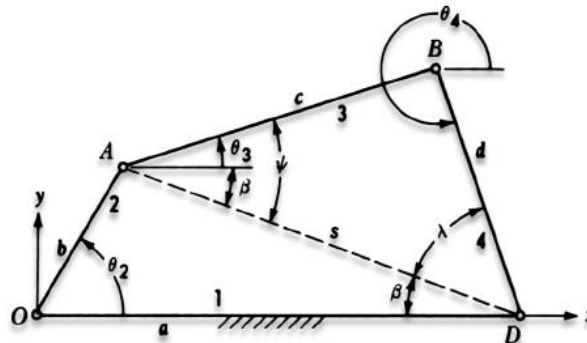
Fig. 35 Mecanismo de cuatro barras [15]
