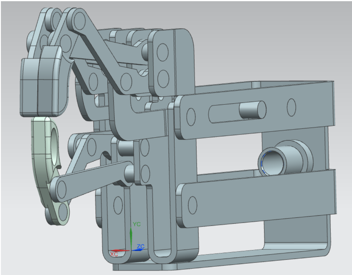
Fig. 45 Diseño prototipo prótesis mecánica de mano
