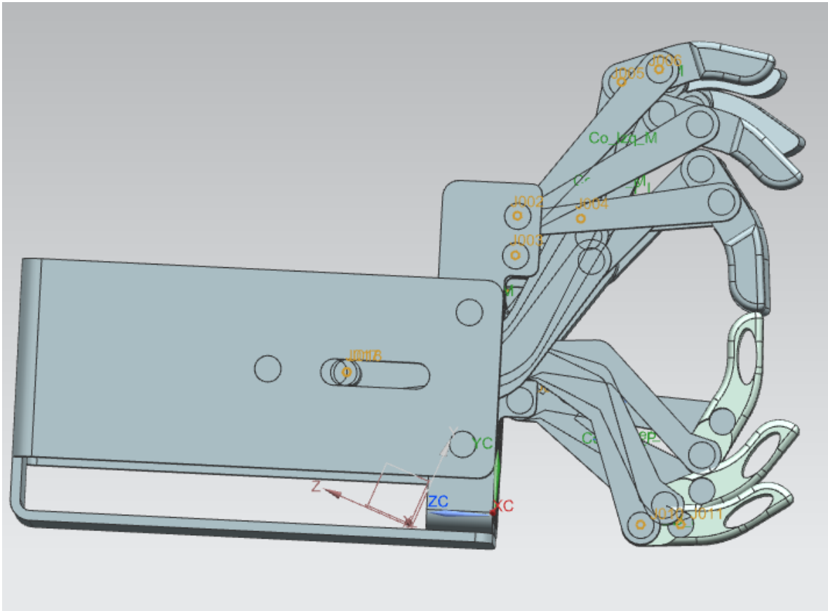
Fig.49 Movimiento de la prótesis simulado en NX
