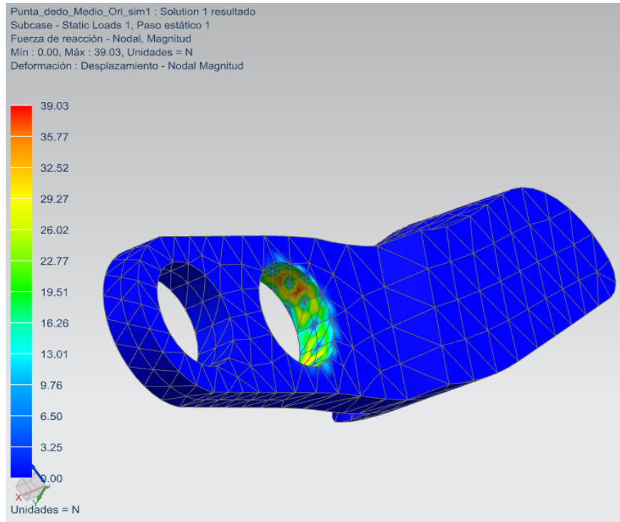
Fig. 47 Esfuerzo de reacción NX
