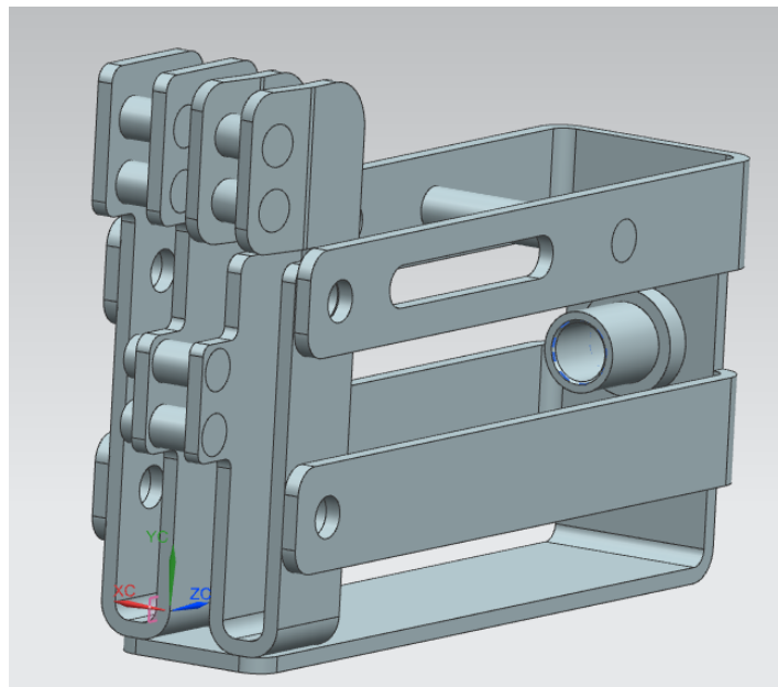
Fig. 44 Base prototipo 2 final de lámina diseñada en NX
