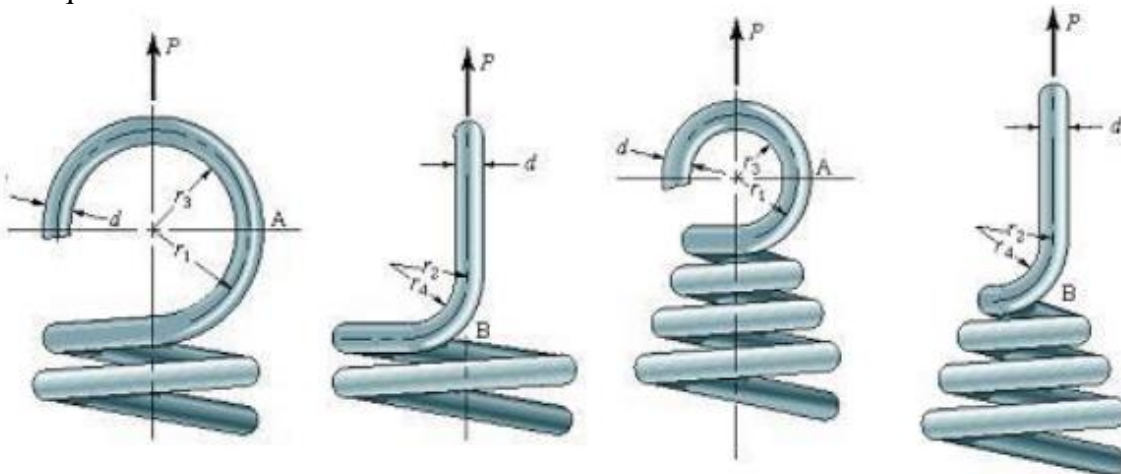
Fig. 39 Resorte helicoidales con extensión.
