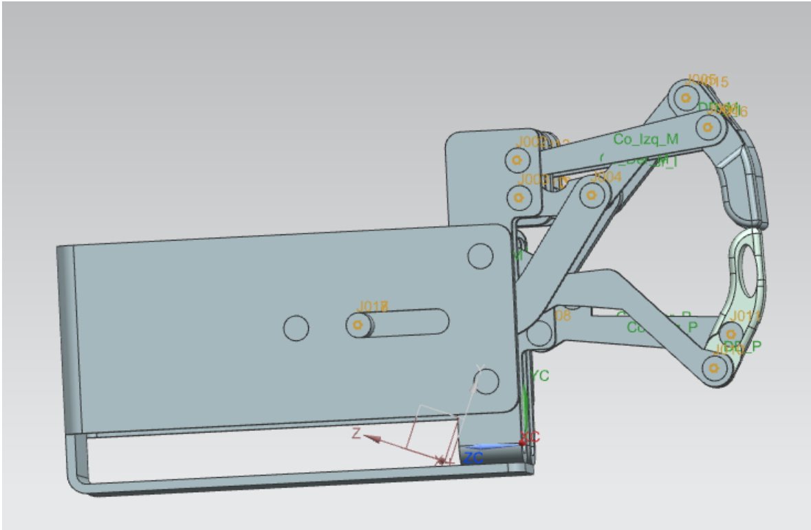
Fig. 48 Diseño de la prótesis normalmente cerrado
