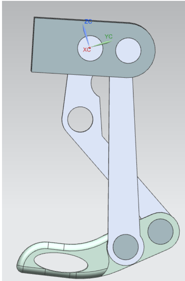
Fig. 42 Mecanismo dedo en reposo realizado en NX
