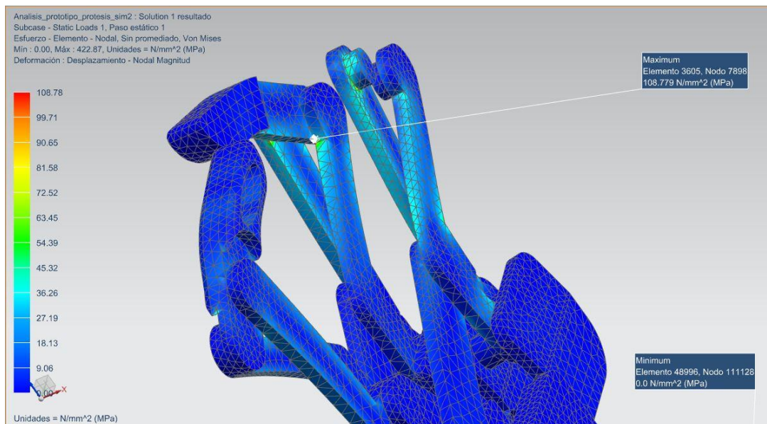
Fig. 52 Análisis esfuerzo del prototipo en NX con carga (sin el dedo Índice)
