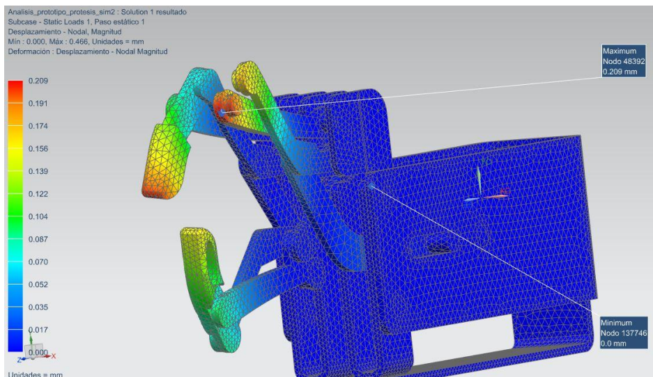
Fig. 52 Análisis desplazamiento del prototipo en NX con carga (sin el dedo Índice)
