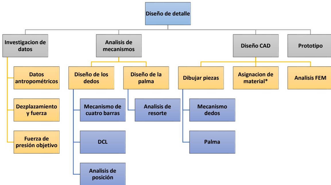
Fig. 3.1 Proceso de diseño para el prototipo de prótesis.
