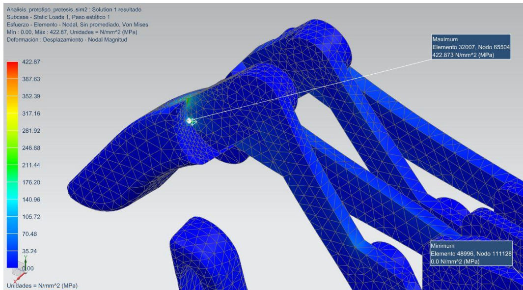
Fig. 51 Análisis esfuerzo del prototipo en NX con carga (completa)
