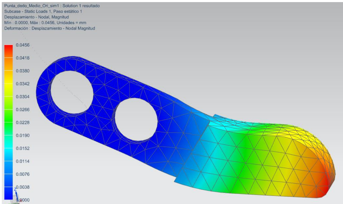
Fig.45 Desplazamiento aplicando fuerza en NX
