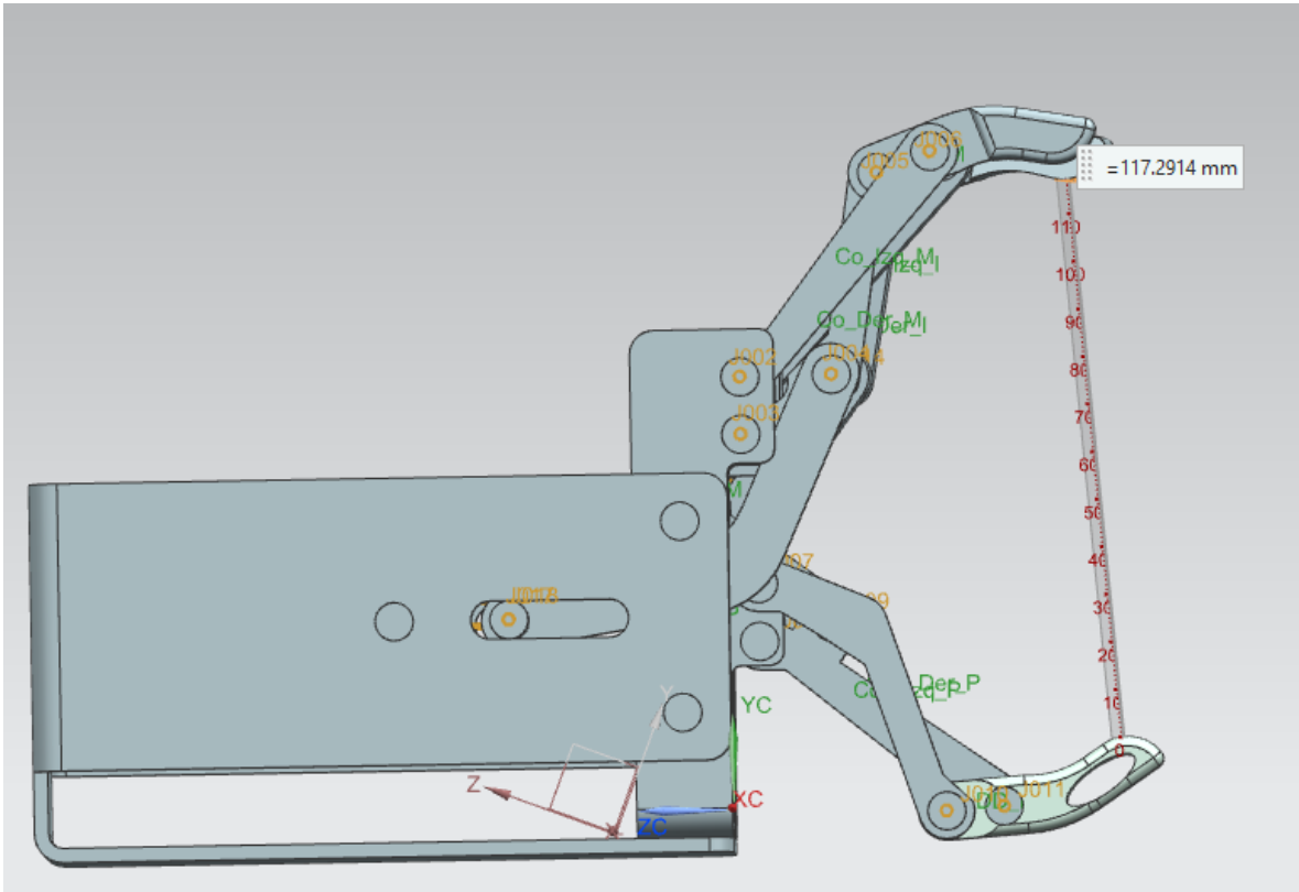
Fig. 50 Apertura máxima funcional
