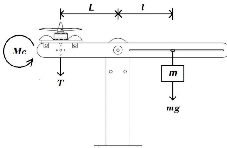
Figura A.4-2. Diagrama del sistema para determinar k .
