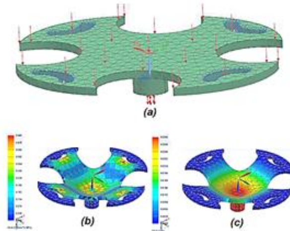
Figura 3-36. Análisis estructural estático de la placa inferior del dron durante sustentación en vuelo. (a) Configuración de cargas. (b) Distribución de esfuerzos. (c) Distribución de deformaciones.
