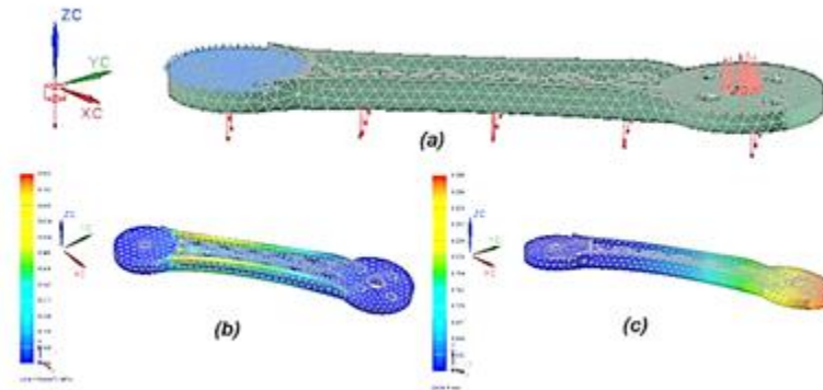
Figura 3-31. Análisis estructural estático de un brazo durante reposo. (a) Configuración de cargas. (b) Distribución de esfuerzos. (c) Distribución de deformaciones.
