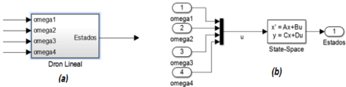
Figura 5-5. (a) Bloque de subsistema que representa al dron lineal. (b) Interior del bloque de subsistema.
