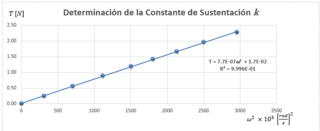
Figura A.4-6. Gráfica de empuje contra el cuadrado de la velocidad angular para el par motor-propela.
