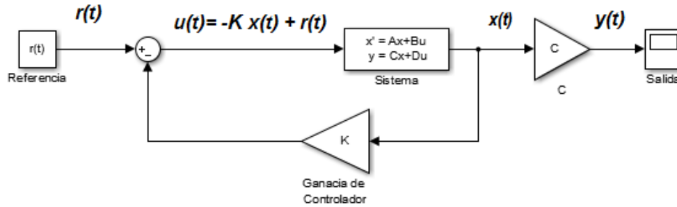
Figura 5-3. Sistema de control por retroalimentación de estados.
