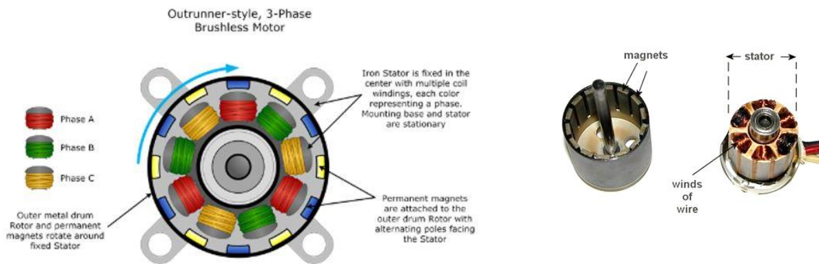
Figura 3-14. Motor Brushless en configuración outrunner.
