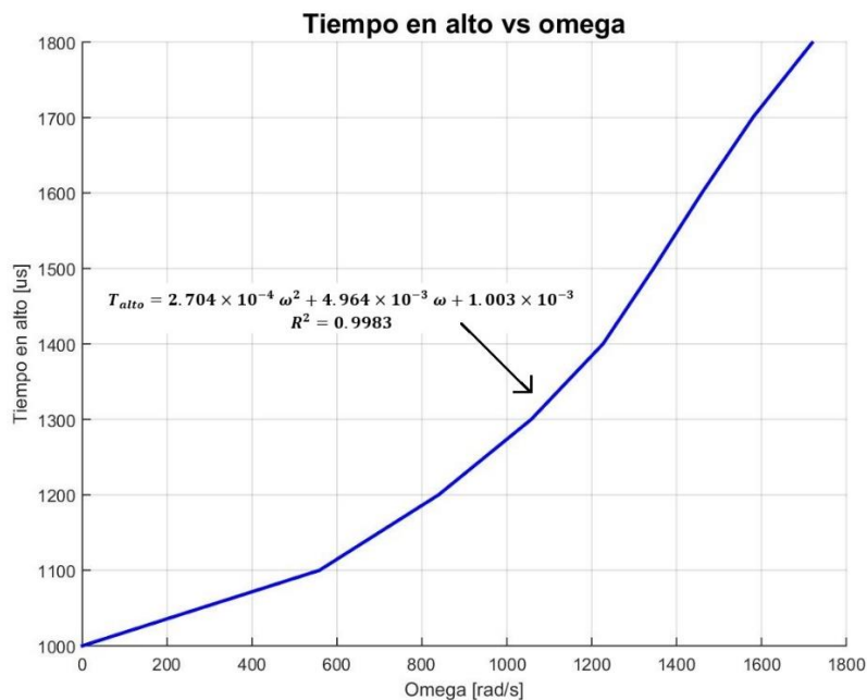
Figura 5-1. Gráfica de T_{alto} vs \omega .
