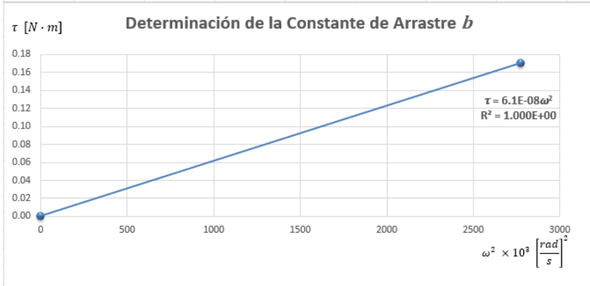
Figura A.4-7. Gráfica de empuje contra el cuadrado de la velocidad angular para el par motor-propela.
