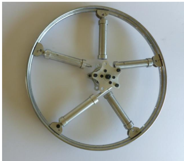
Figura 63. Diseño final de la rueda, hecha en aluminio con cinco amortiguadores finales como brazos.
