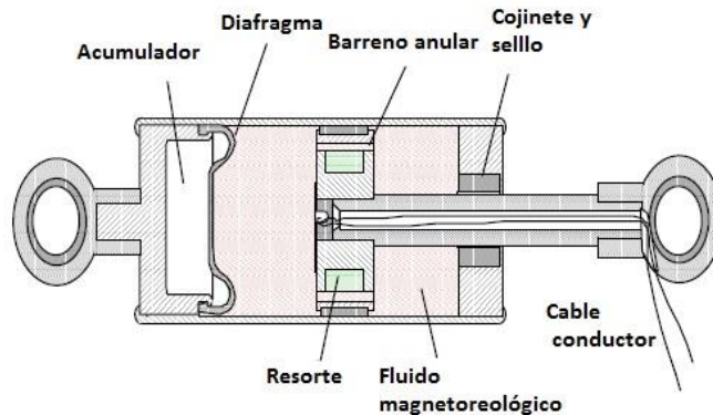
Figura 6. Esquema de un amortiguador magnetoreológico [13].
