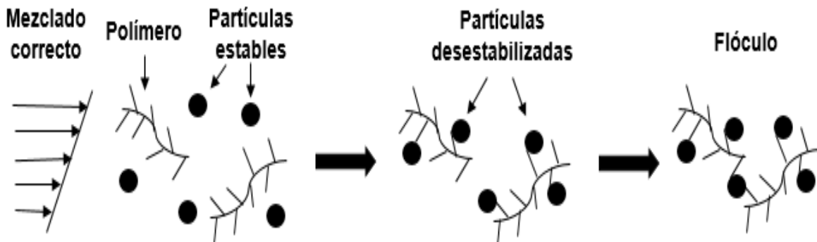
Figura 1. 9. Mecanismo de formación de puentes para la desestabilización de partículas por polímeros orgánicos (Montgomery, 2005).
