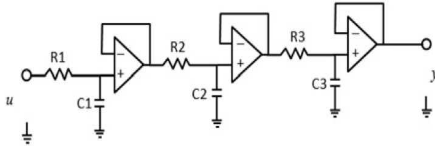
Figura 4.2: Circuito RC
