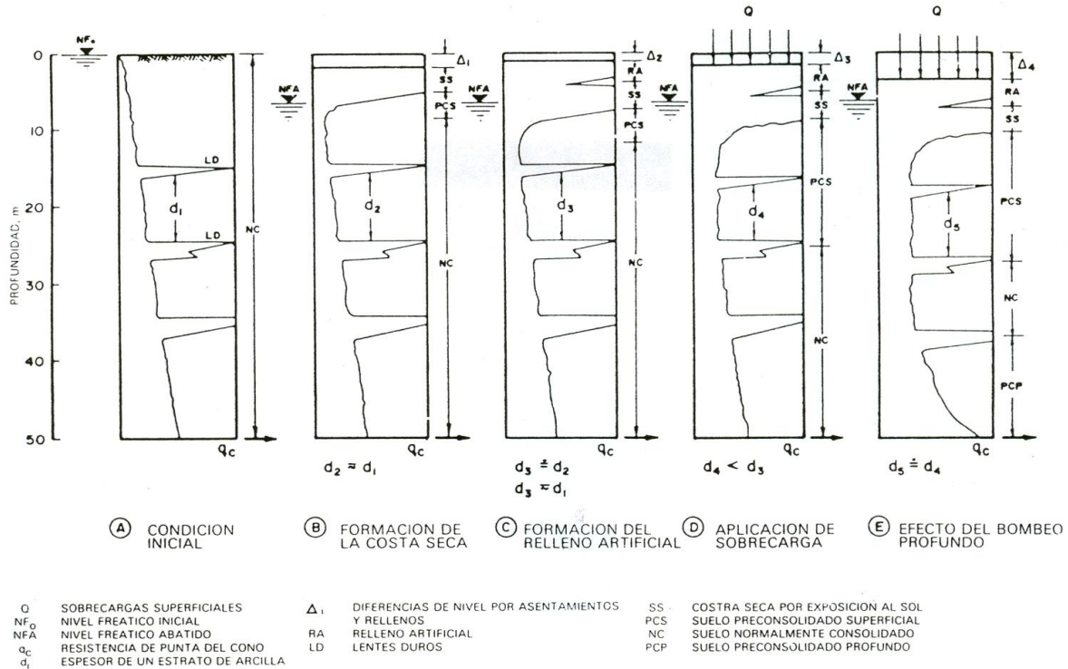
Figura 1.9 Evolución de la resistencia al corte.
