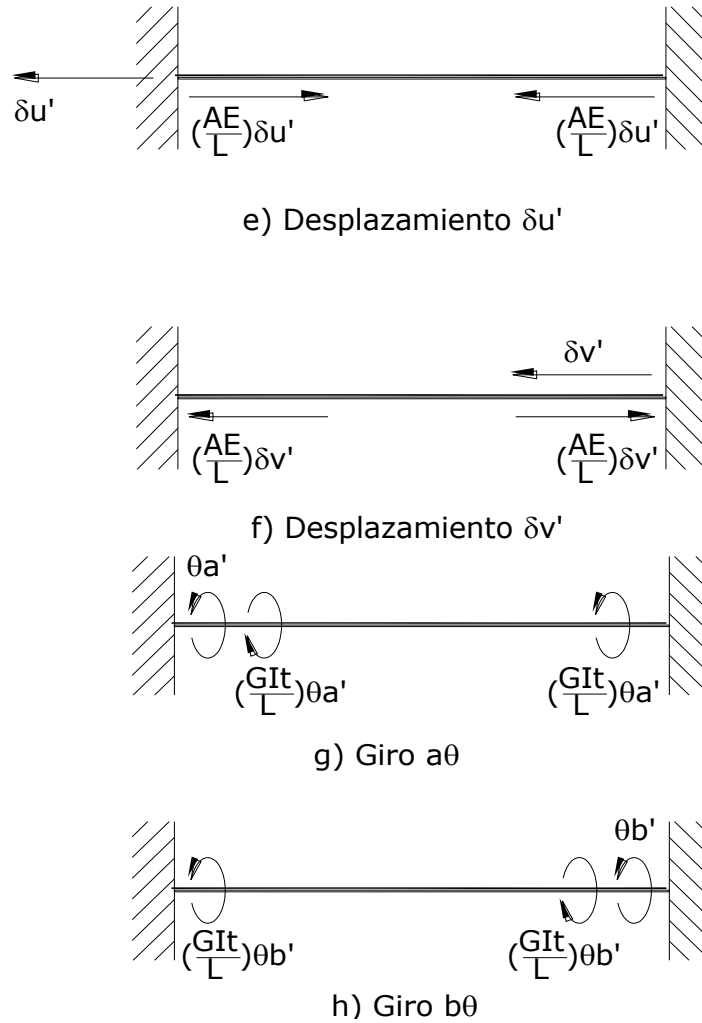
Figura 3.5. Elementos mecánicos ocasionados por desplazamientos angulares y lineales.
