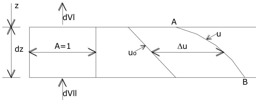
Figura 3. Flujo vertical a través de un elemento de suelo.
