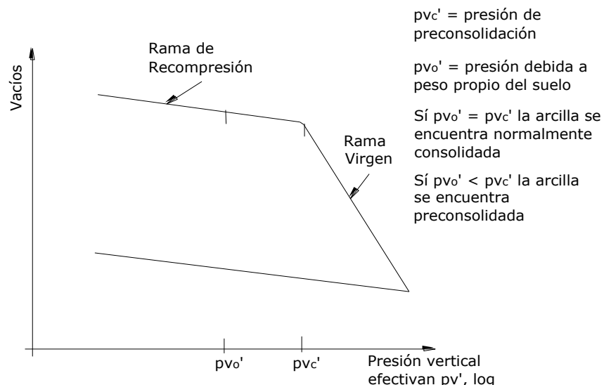
Figura 2.16 Curva de compresibilidad.
