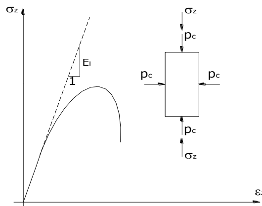
Figura 2.9 Curva esfuerzo-deformación unitaria de un suelo.
