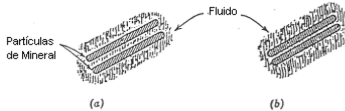
Figura 2.4 Capa de fluido rodeando una muy pequeña partícula de suelo. (a) Antes de la carga. (b) Partículas comprimidas, juntándose debido a la carga. (Lambe y Whitman, 1969)
