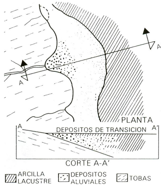
Figura 1.16 Transición estratificada ancha.
