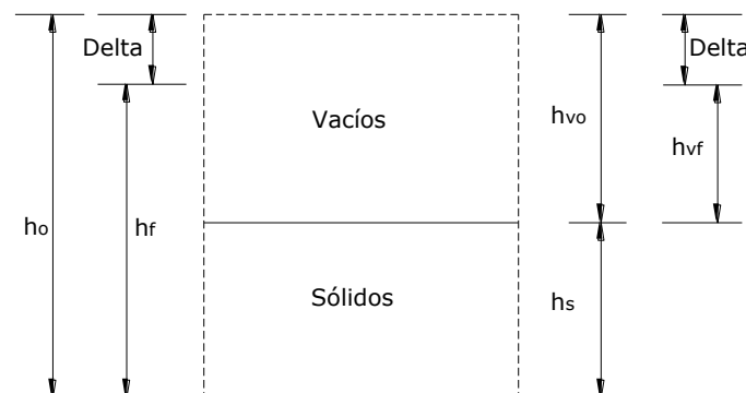
Figura 2.15 Deformación de un elemento de suelo.
