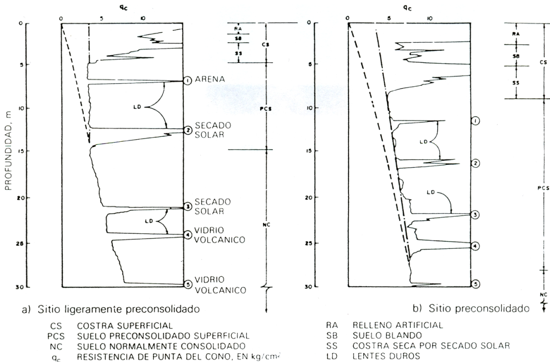
Figura 1.10 Perfiles tipo de los suelos de la zona del lago, en función de la resistencia al corte determinada con cono.
