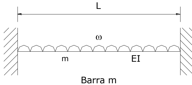
Figura 3.3. Barra empotrada con apoyos continuos, sometida a una carga uniformemente repartida.
