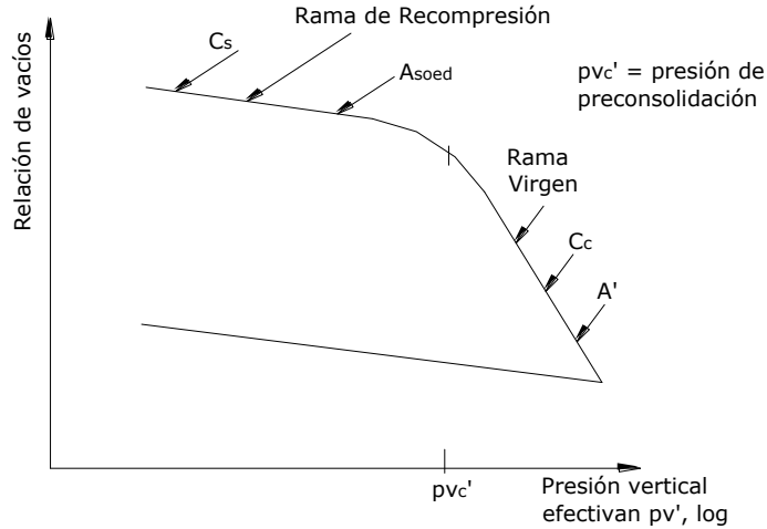
Figura 2.19 Curva de compresibilidad de una arcilla no sensitiva.
