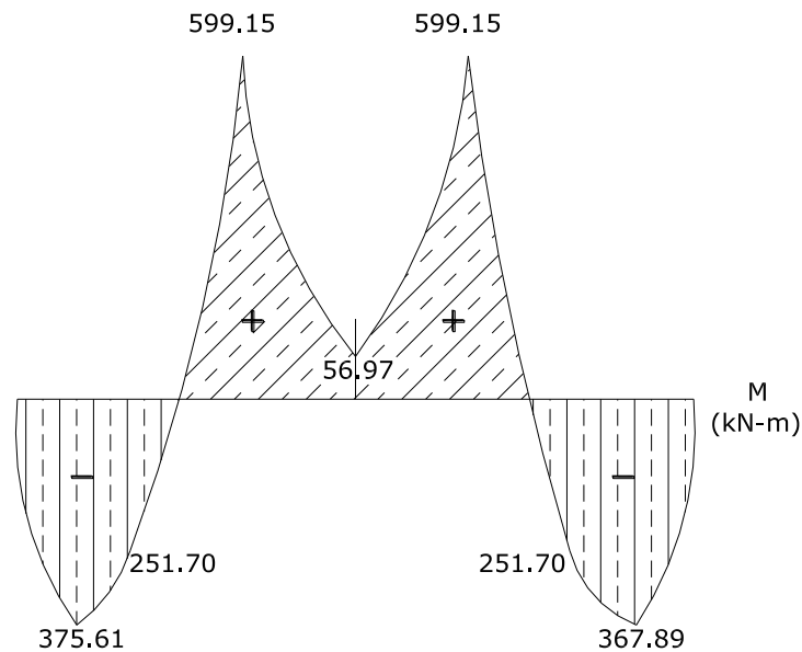
Diagrama de Momento Flexionante.
