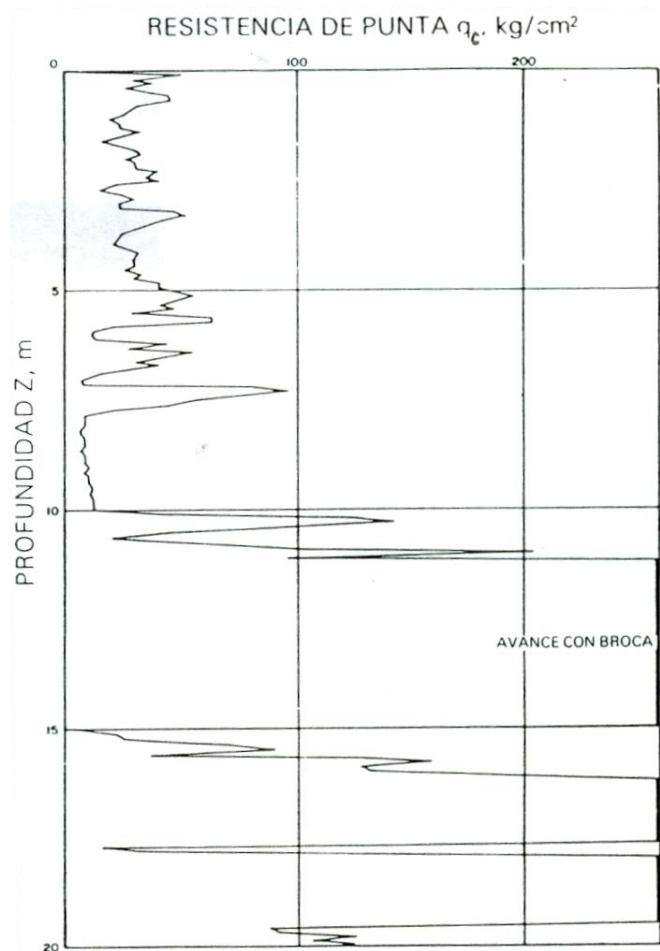
Figura 1.19 Sondeo de cono eléctrico en la subzona de transición alta.
