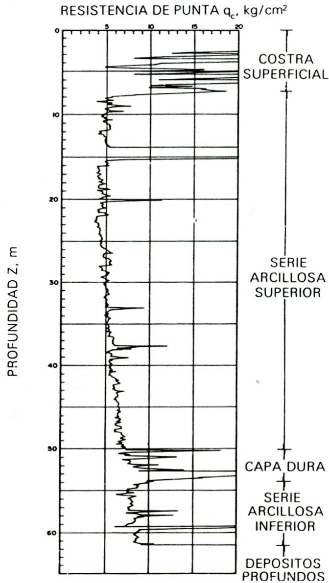
Figura 1.11 Sondeo de cono eléctrico en la zona del lago.
