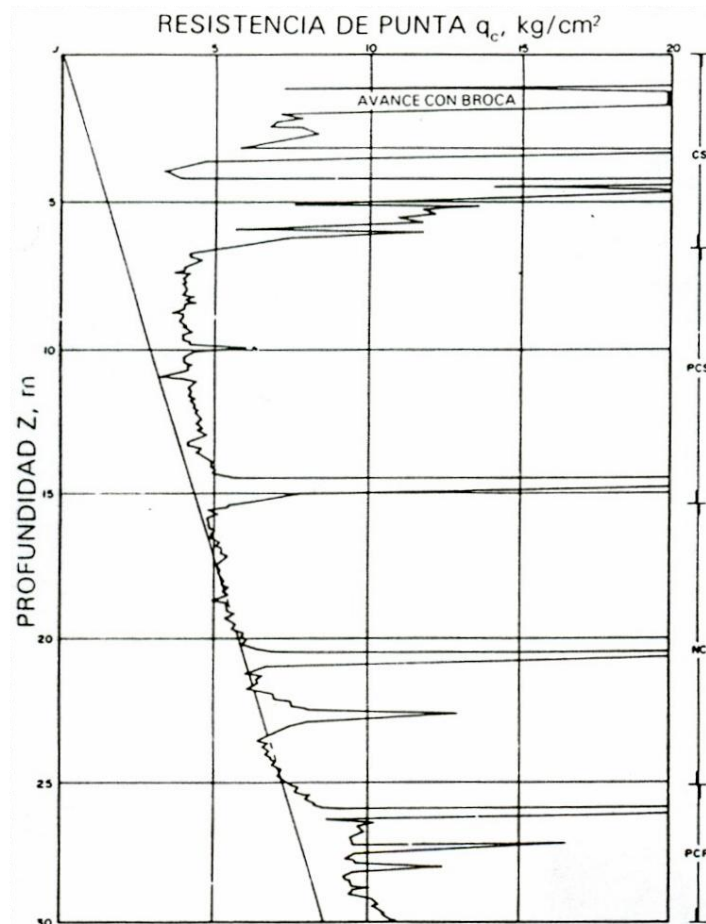
Figura 1.14 Sondeo de cono eléctrico en la subzona del Lago Centro II.
