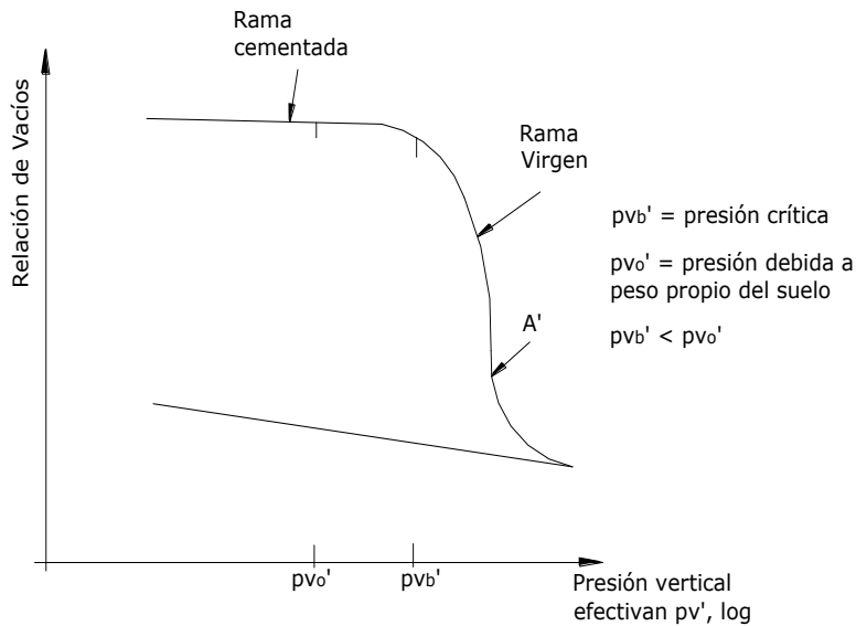
Figura 2.17 Curva de Compresibilidad, Arcilla Sensitiva.
