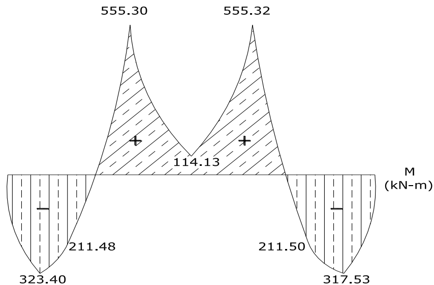
Diagrama de Momento Flexionante.
