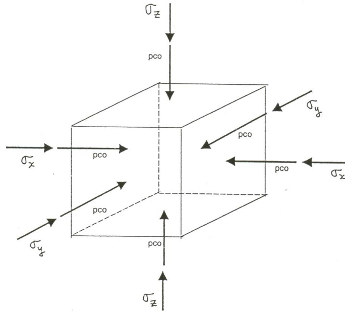
Figura 2.12 Esfuerzos en un elemento de suelo. Incrementos de esfuerzo por la presencia de una obra de ingeniería.
