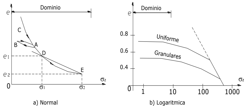
Figura 2.8 Curvas de Compresión.
