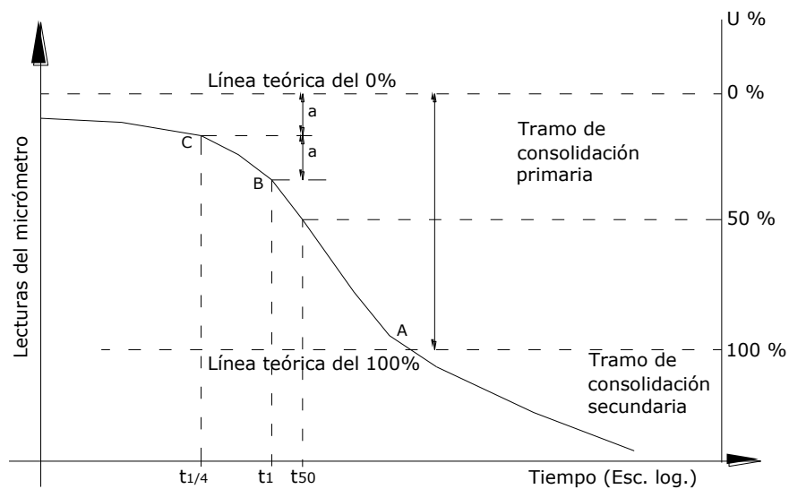
Figura 2.14 Determinación del 0% y del 100% de consolidación primaria en una curva de consolidación.
