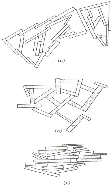
Figura 2.6 Estructura sedimentada. (a) Floculación salada. (b) Floculación no salada. (c) Dispersión. (Lambe y Whitman, 1969)
