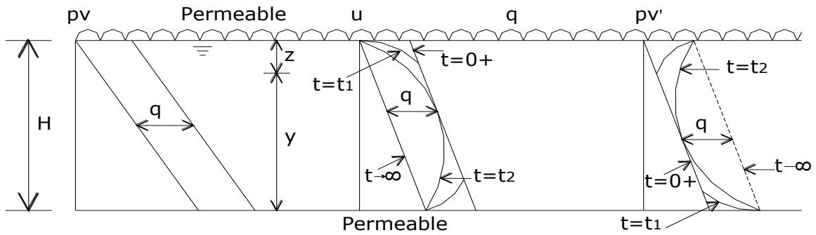
b) Diagramas de presión con un incremento de carga repartida q.
