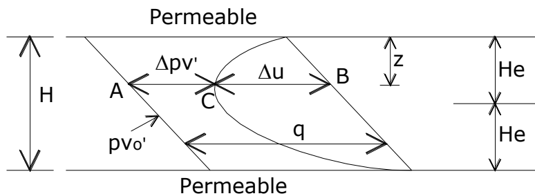
Figura 4. Grado de consolidación de un estrato de arcilla de espesor H.
