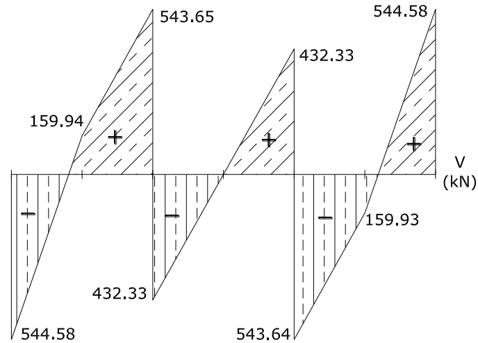
Diagrama de Fuerza Cortante.
