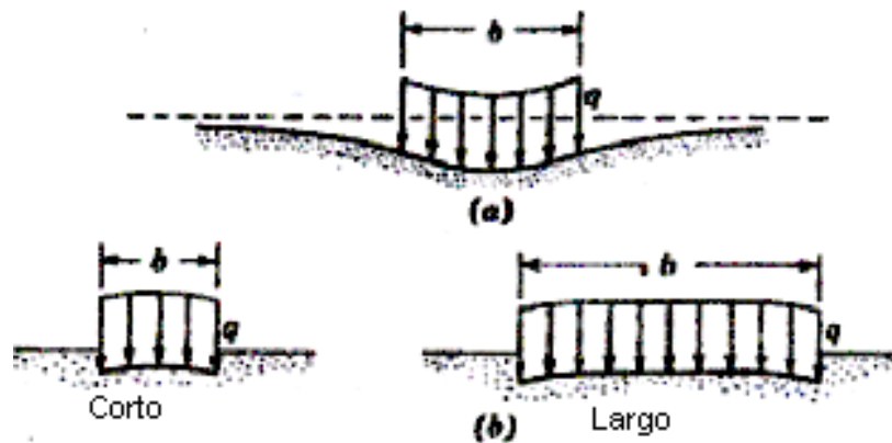
Figura 3.1. Perfil de distorsión que genera una carga uniforme en la superficie de una masa de suelo. (a) Material isotrópico elástico homogéneo, tales el caso de una arcilla saturada.; (b) Material elástico homogéneo el cual aumenta su rigidez con el confinamiento, tal es el caso de una arena de poca cohesión u una grava.
