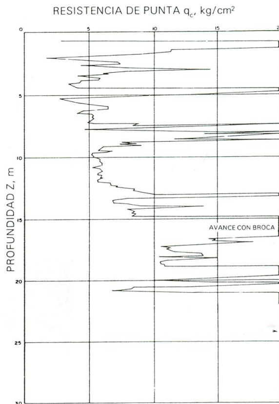
Figura 1.20 Sondeo de cono eléctrico en la subzona de transición baja.
