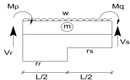
Elementos mecánicos en la barra m.
