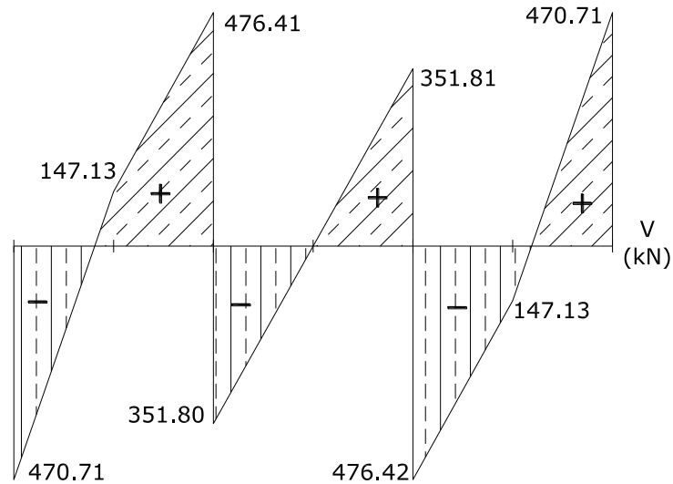
Diagrama de Fuerza Cortante.
