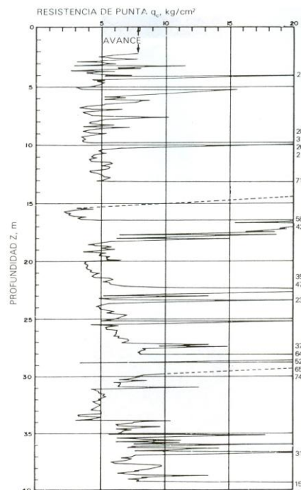
Figura 1.22 Sondeo de cono eléctrico cercano al Peñón de los Baños
