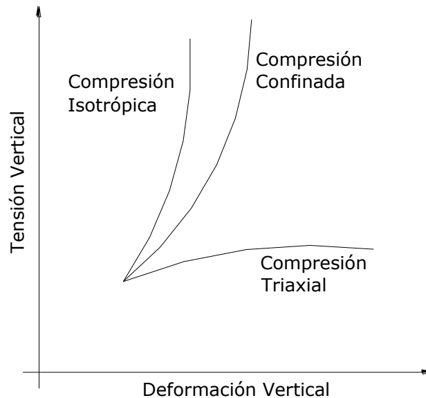
Figura 2.7 Comparación de las curvas tensión-deformación, para los tres tipos de compresión. (Lambe y Whitman, 1969)
