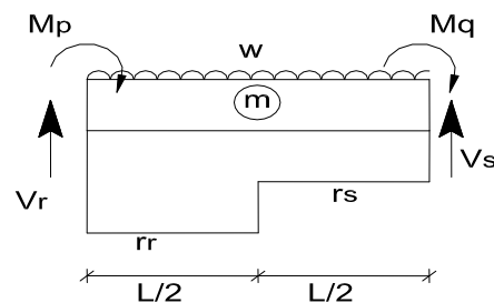
Elementos mecánicos de la barra m.
