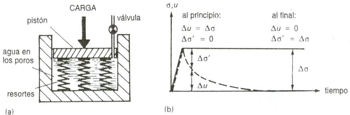
Figura 2.13 Consolidación unidimensional. (a) Modelo de Terzaghi. (b) Curva esfuerzo/tiempo.
