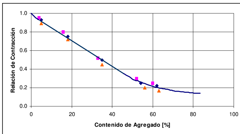
Figura V.4. Influencia del contenido de agregado del concreto (por volumen) en la Relación de la contracción del concreto y la contracción de la pasta pura de cemento.
