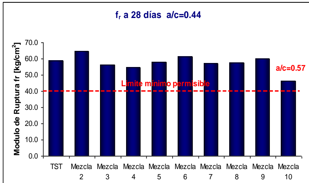
Figura VI.4. Comparativa de módulo de ruptura obtenido a 28 días.
