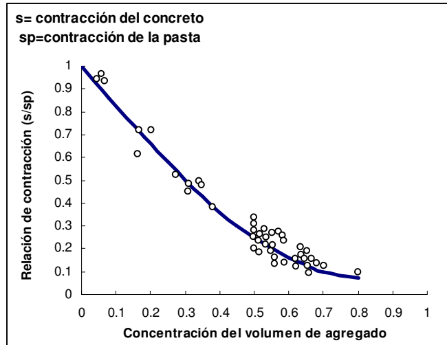
Figura IV.1 Efecto de la concentración del volumen de agregado en la contracción.
