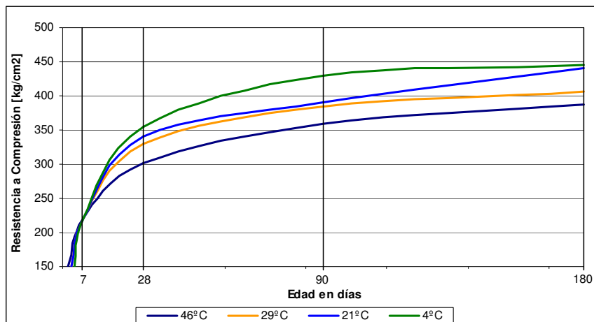
Figura V.2. Efecto de la temperatura del colado de concreto en el desarrollo de resistencia
