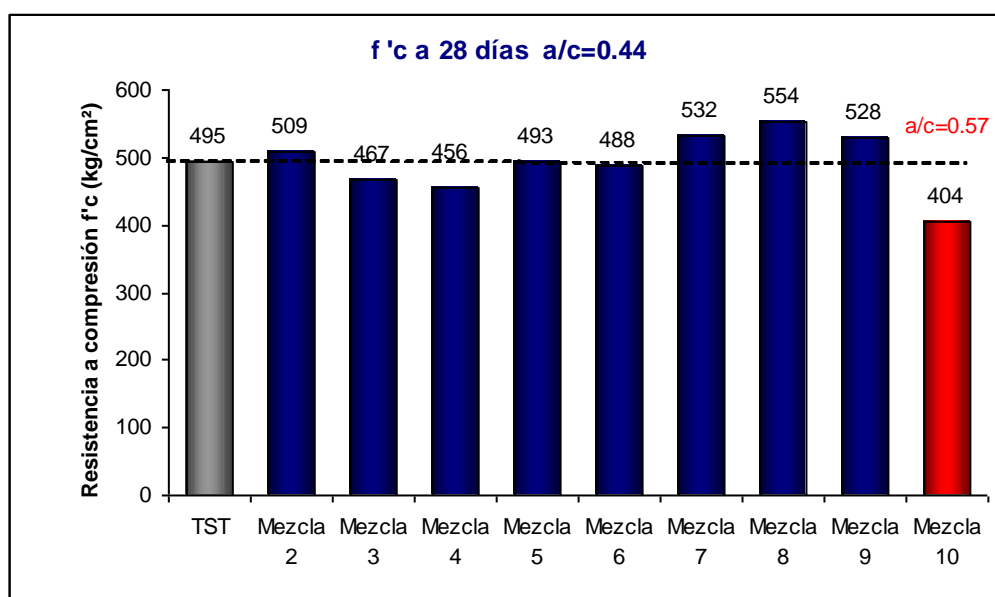
Figura VI.3. Comparativa de resistencia a compresión a 28 días de las mezclas en estudio.
