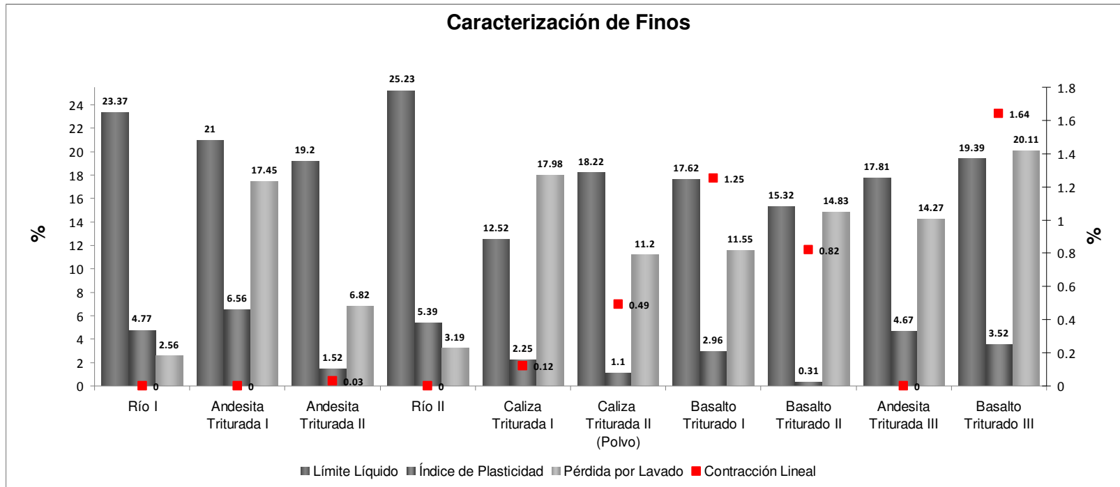
Figura IV.2 Comparativa de las propiedades de las partículas finas de los agregados empleados
