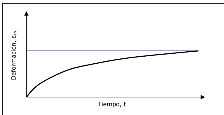
Figura V.3. Curva contracción - tiempo.
