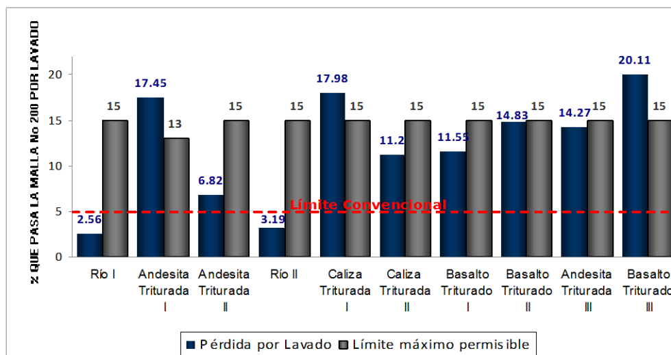
Figura VI.2. Comparativa del porcentaje de partículas menores a la criba 0.075mm Obtenido con el Límite Convencional y el Máximo permisible con base en resultados de plasticidad.
