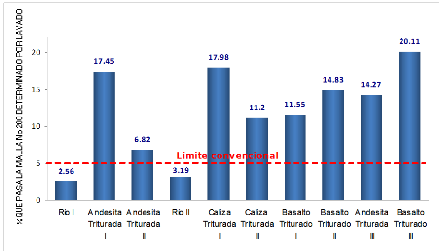
Figura VI.1. Comparativa del % de pérdida por lavado de las distintas arenas analizadas.
