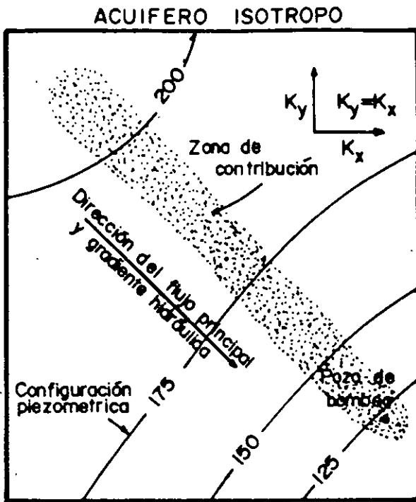
A. Efecto de la anisotropía en la orientación de la zona de contribución.
