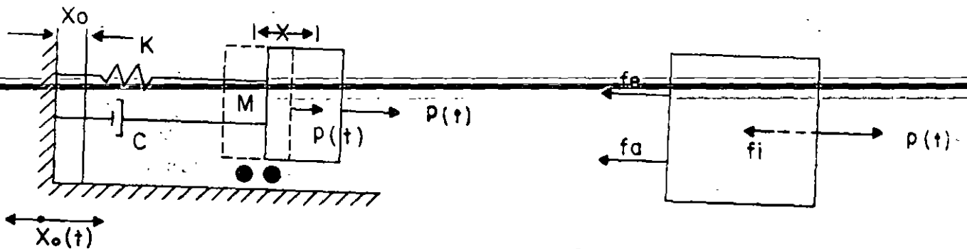
DIAGRAMA DE CUERPO LIBRE
