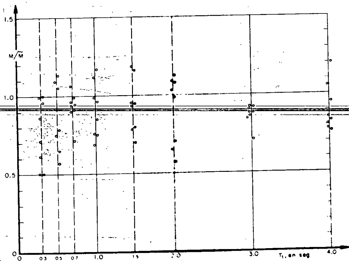
Fig 12. Resultados de los momentos sordionantes para \eta = 1.0 , y \zeta = 0.10 . Método 2
