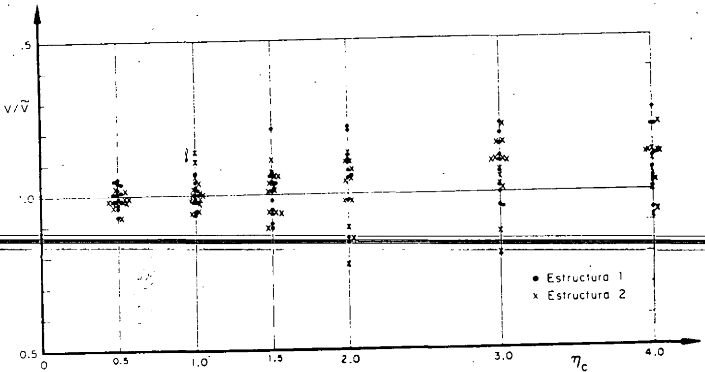
Fig 21. Fuerzas cortantes normalizadas estimadas con el método 2, para \zeta = 0.10 . Problema de cabeceo
