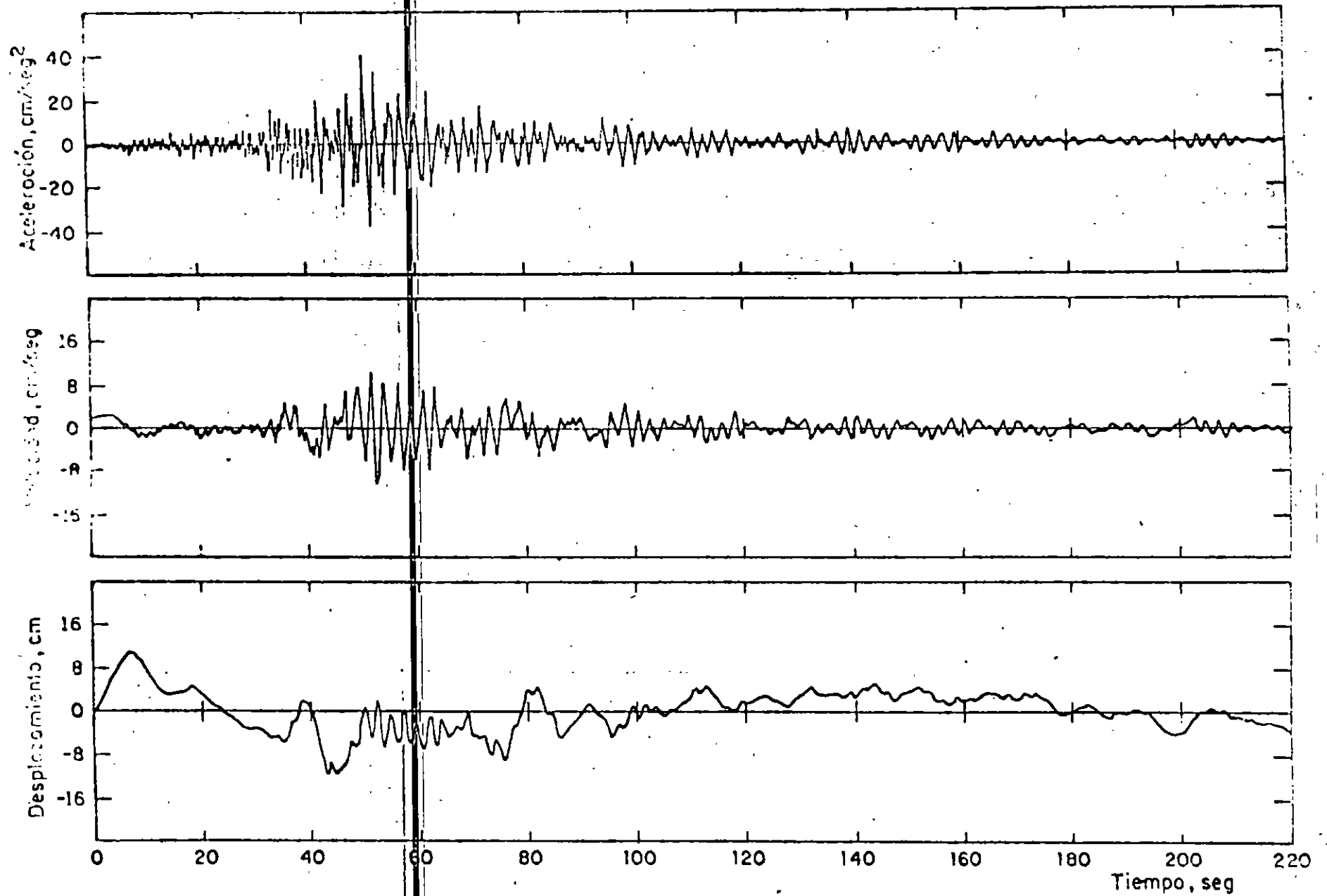
CF Fig 8 Movimiento del terreno. Alameda Central, 11 de mayo de 1962
