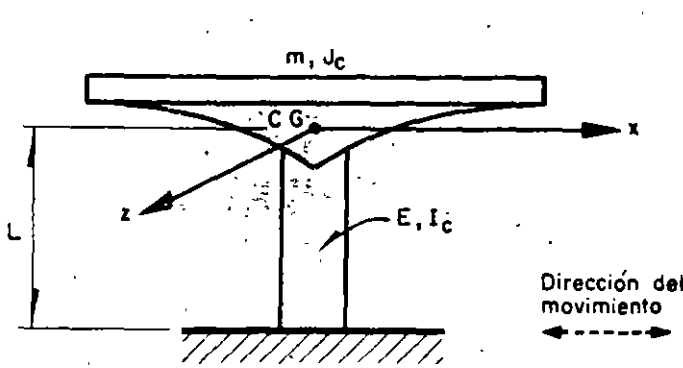
Fig A.2. Estructura en forma de péndulo invertido (vista lateral)
