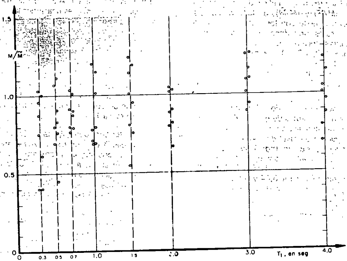
Fig 11. Resultados de los momentos sordionantes para \eta = 1.0 , y \zeta = 0.05 . Método 2
