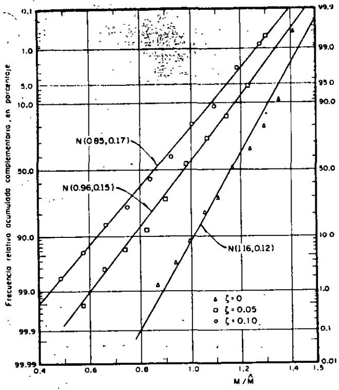
Fig 17. Resultados de los momentos torsionantes para \eta = 1.5, 2.0, 2.5, 3.0 y 4.0 mezclados. Papel de probabilidades normal, método 1
