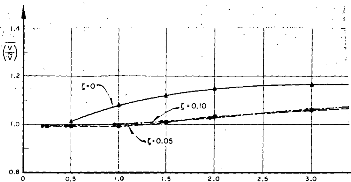
Fig. 22. Variación con T_1 de los promedios de las fuerzas cortantes estimadas con el método 2. Problema 1
