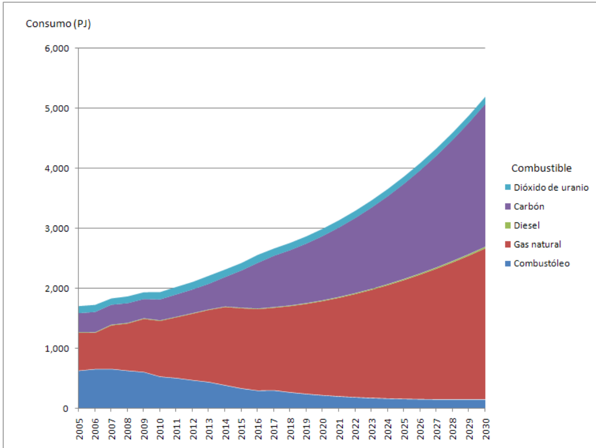
Figura 5.3 Consumo de combustibles para la generación de energía eléctrica en el servicio público al año 2030 para el escenario de referencia (PJ)
