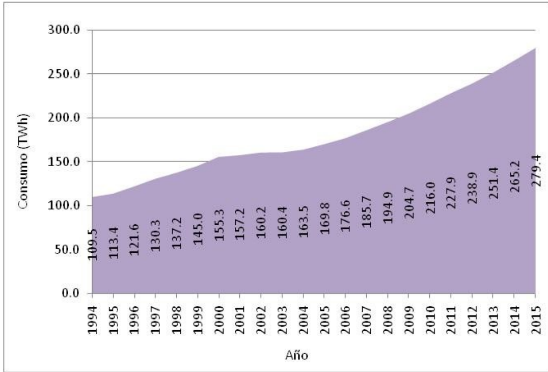
Figura 4.7 Consumo de energía eléctrica en el servicio público (escenario de planeación)
