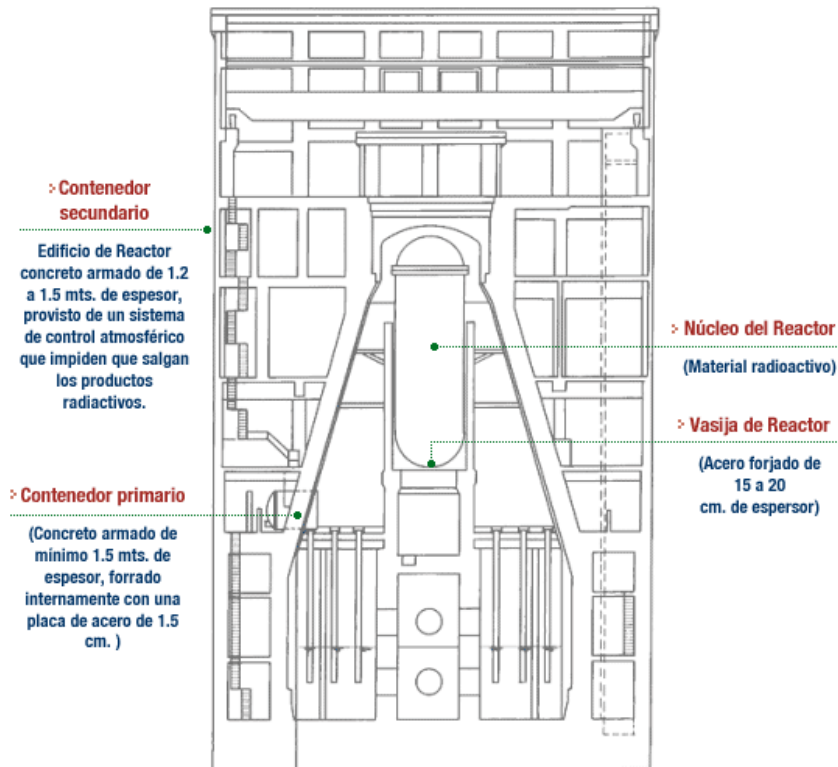
Figura 4.6 Barreras de contención de radiaciones y material radiactivo de la central Laguna Verde
