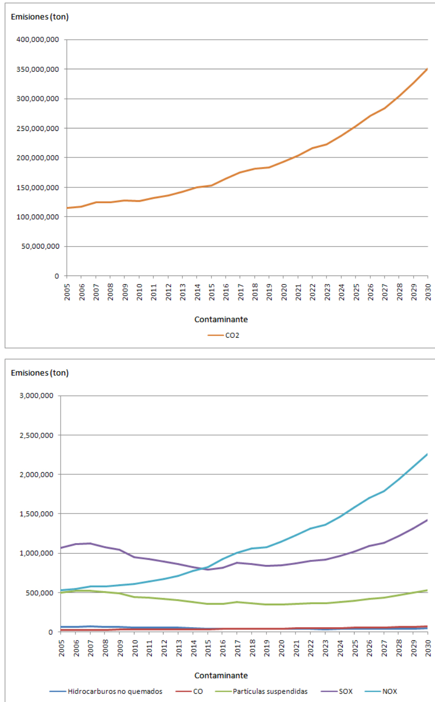
Figura 5.8 Emisiones contaminantes producidas por la generación de energía eléctrica en el servicio público al año 2030 para el escenario medio (ton)
