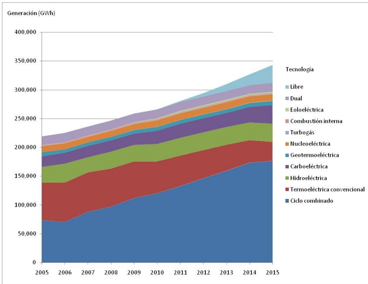
Figura 4.10 Contribución de cada tecnología a la generación bruta en el servicio público
