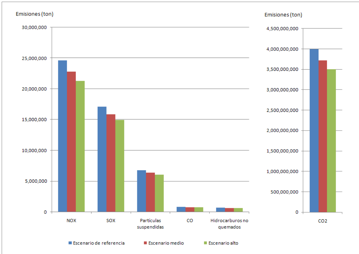
Figura 5.14 Comparación de emisiones contaminantes acumuladas por la generación de electricidad entre los años 2015 y 2030 para los tres escenarios estudiados (servicio público)
