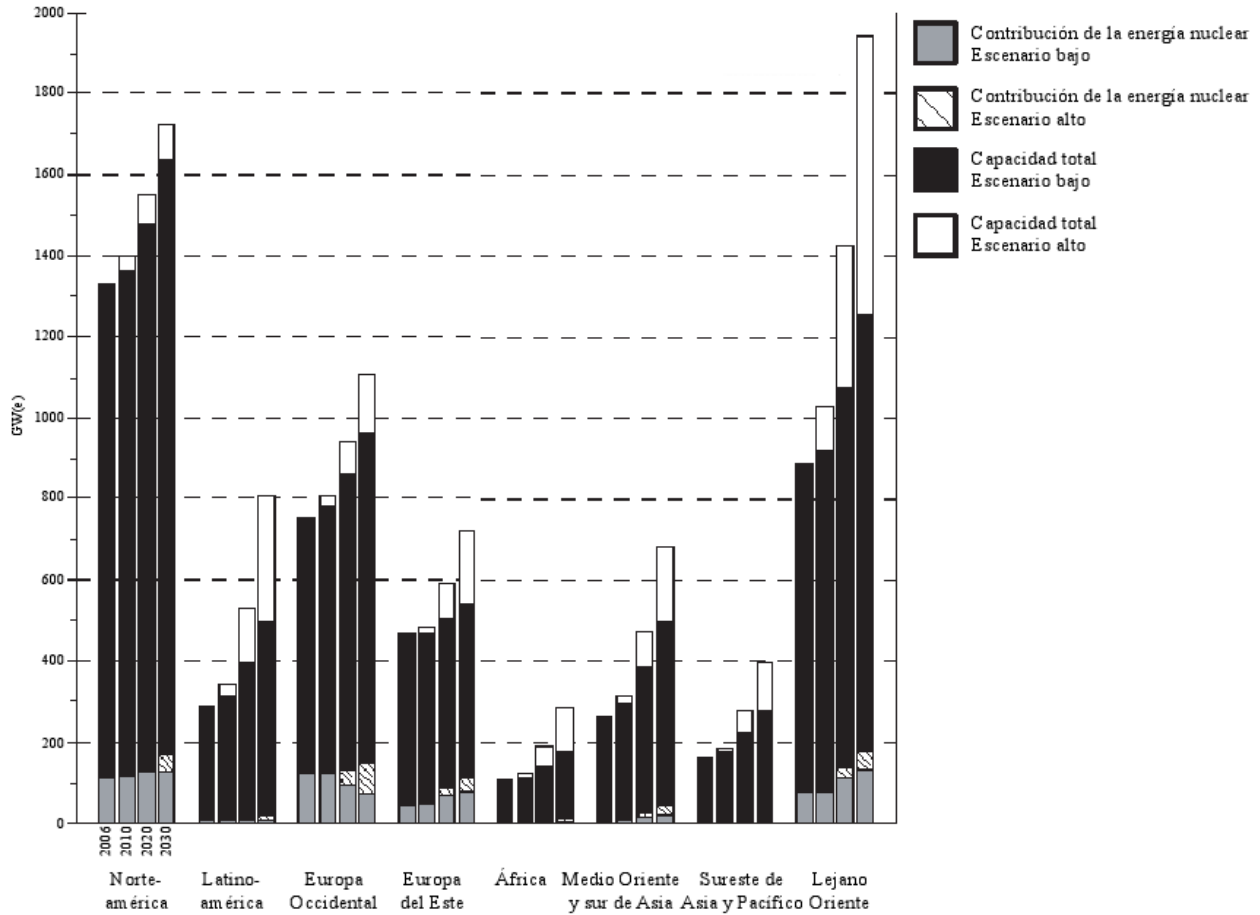
Figura 3.10 Capacidad de generación total y nuclear al final de cada año
