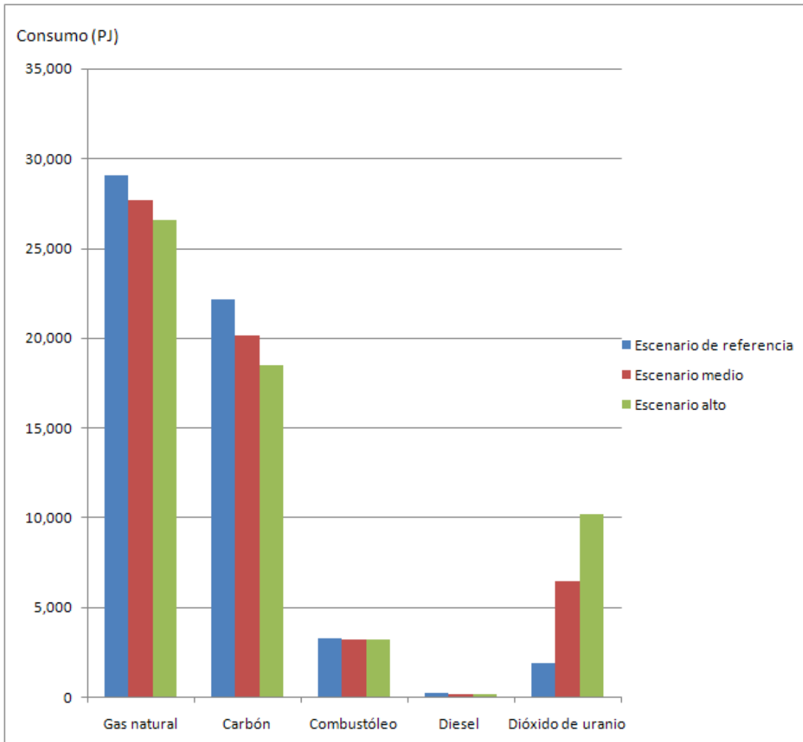
Figura 5.13 Comparación del consumo acumulado de combustibles para la generación eléctrica entre los años 2015 y 2030 para los tres escenarios estudiados (servicio público)
