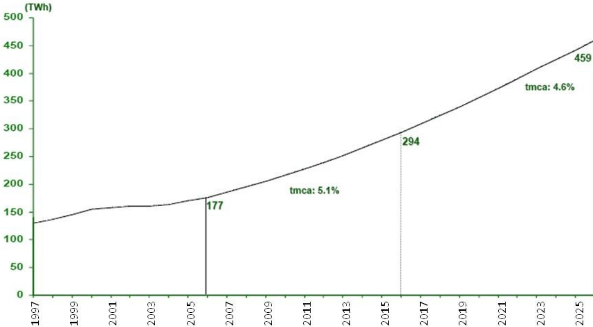
Figura 4.12 Historia y estimación de las ventas de energía eléctrica (escenario de planeación)
