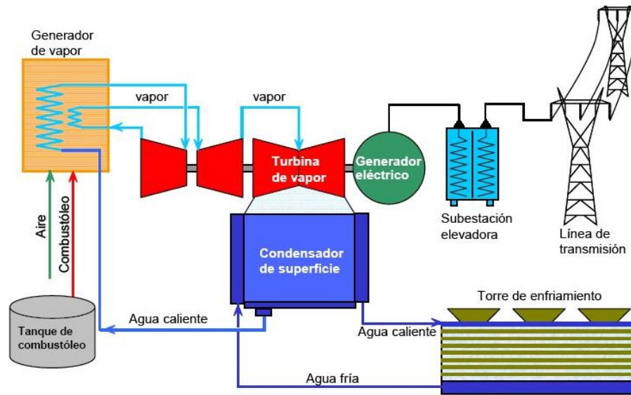
Figura 1.1 Central termoeléctrica convencional
