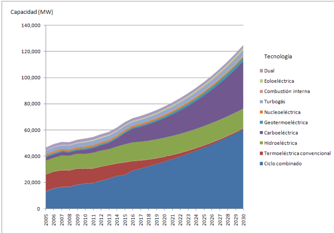
Figura 5.1 Evolución de la capacidad instalada en el servicio público al año 2030 para el escenario de referencia (MW)
