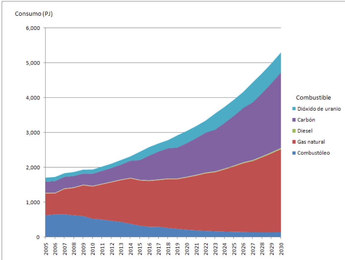
Figura 5.7 Consumo de combustibles para la generación de energía eléctrica en el servicio público al año 2030 para el escenario medio (PJ)
