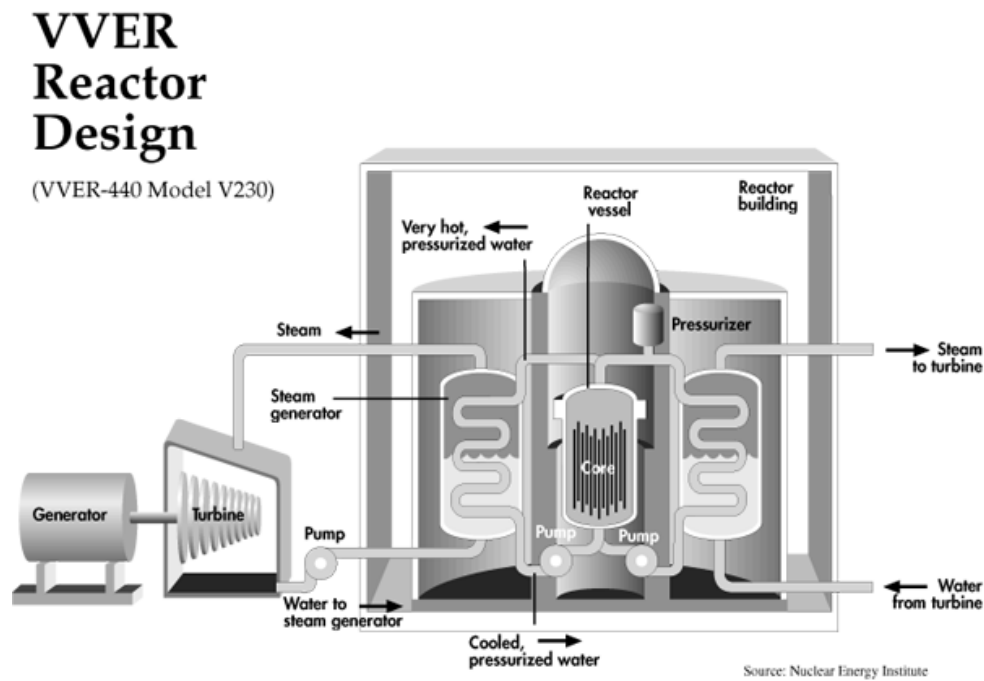
Figura 2.9 Reactor VVER
