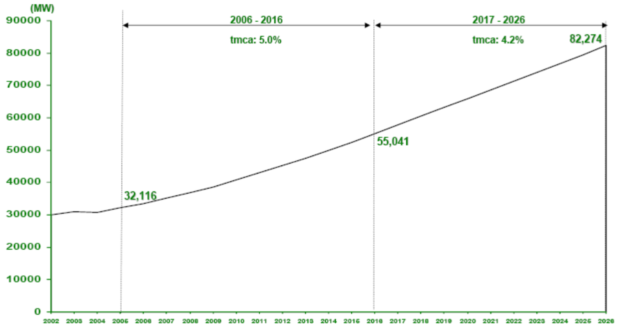
Figura 4.13 Historia y estimación de la demanda del sector eléctrico (escenario de planeación)
