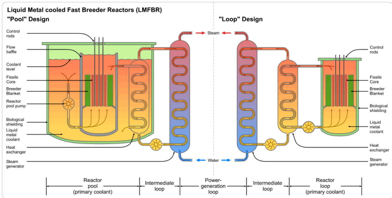
Figura 2.11 Dos diseños diferentes de reactor LMFBR
