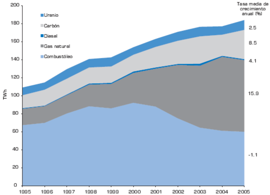
Figura 4.4 Generación bruta en el servicio público por tipo de combustible utilizado entre los años 1995 y 2005 (TWh)
