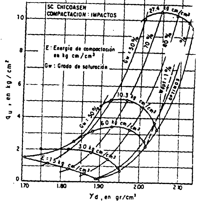
Fig 6. Resistencia no confinada en función de \gamma_d para valores diferentes de G_w .
