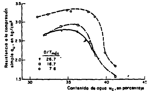
Fig. 11 Variación de la resistencia q_u p el efecto de escala
