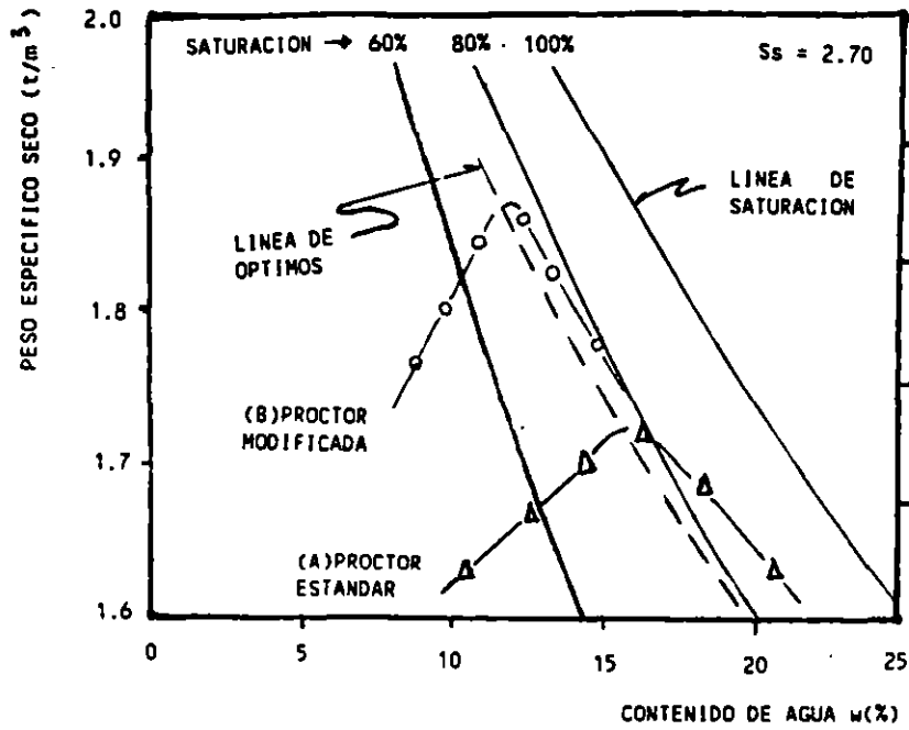
FIG 1 CURVAS DE COMPACTACION PROCTOR ESTANDAR Y PROCTOR MODIFICADA.
