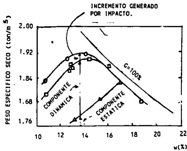
FIG 15 RESULTADOS DE LA COMPACTACION DE ARENA LIMOSA EN CAPAS DE 30 cm, CON Y SIN VIBRACION USANDO UN RODILLO VIBRATORIO REMOLCADO DE 7700 kg.
