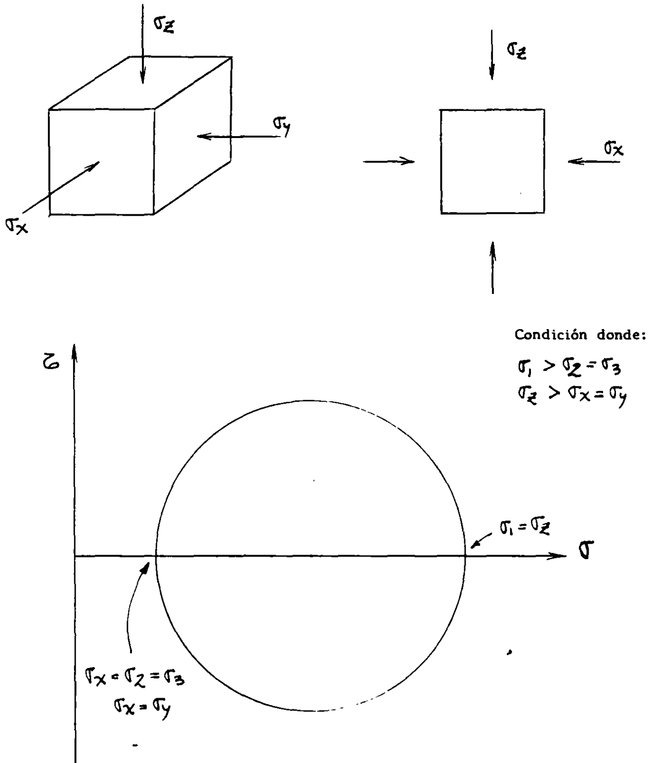
Fig. 7.1.4 Representación tridimensional de Mohr en Análisis plano
