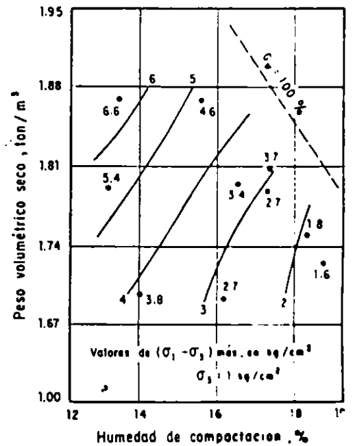
Fig 10. Líneas de igual resistencia a 1 compresión en prueba rápida, si saturación previa y con presión confinante de 1 \text{ kg/cm}^2 .
