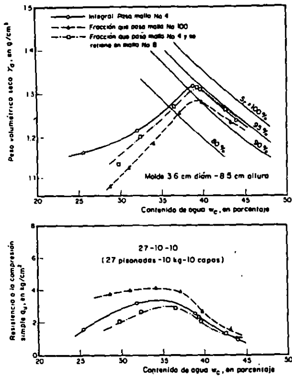
Fig. 8 Efecto de la granulometría de grumos del suelo MH-Necaza secado al ambiente, sobre el \gamma_d y la resistencia q_u . Compactación por amasado
