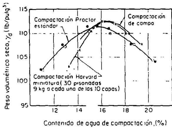
Fig. 1 Comparación de curvas de compactación de laboratorio y campo (ref. 4)
