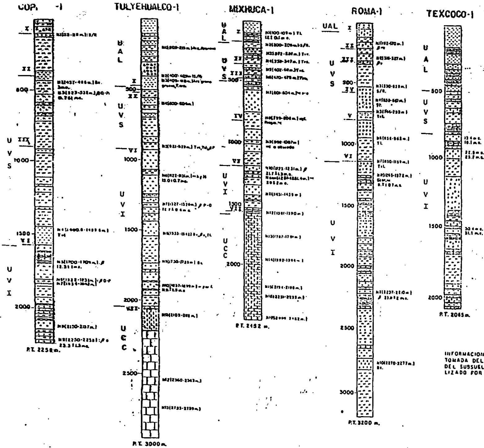
FIG. COLUMNAS GEOLOGICAS DE LOS POZOS PROFUNDOS DE LA CIUDAD DE MEXICO
