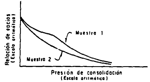
b) Curvas relación de vacíos - presión
