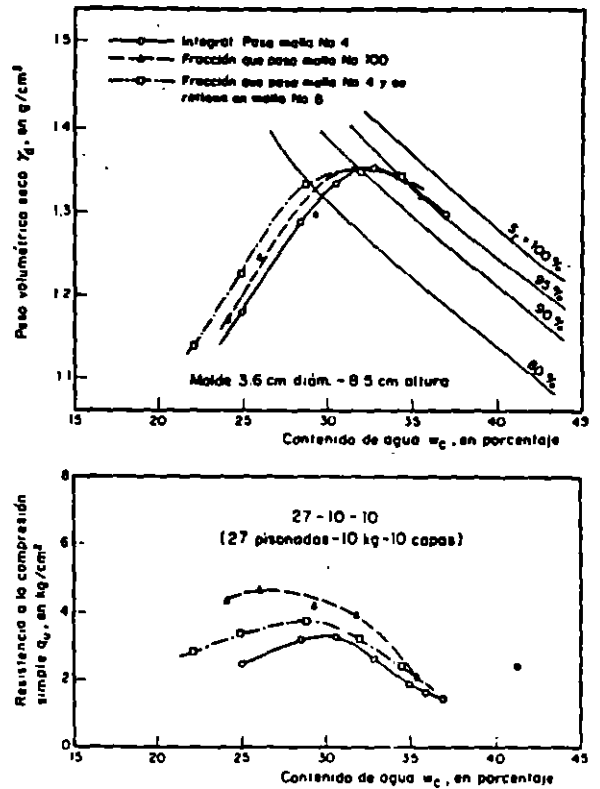
Fig. 9 Efecto de la granulometría de grumos del suelo CH-La Peña secado al ambiente, sobre el \gamma_d y la resistencia q_u . Compactación por amasado
