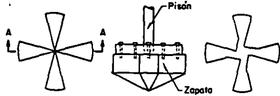
a) Geometría original de la zapata en planta
