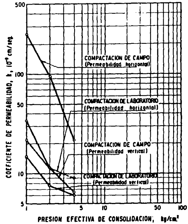
Figura 6 Diferencias de permeabilidad vertical y horizontal en muestras compactadas en el campo y en el laboratorio
