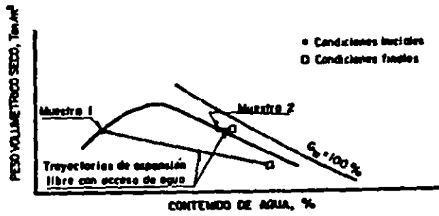
a) Condiciones de compactación y trayectorias de expansión libre con exceso de agua
