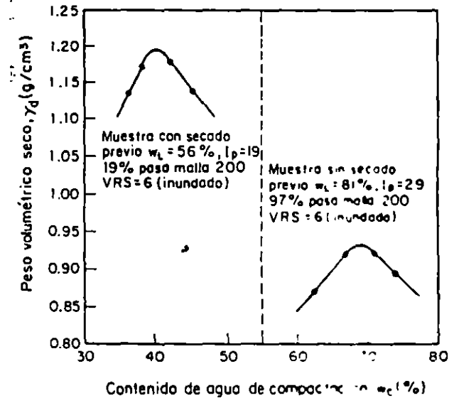
Fig. 16 Comparación de propiedades físicas de especímenes compactados con y sin secado previo
