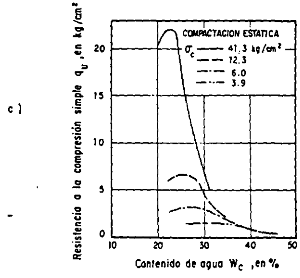
Fig 7. Resistencia a la compresión simple q_u para distintos tipos de compactación en función del contenido de agua de compactación w_c (Ref. 1).
