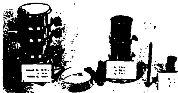
Fig. 4 Vista de moldes y pisonas de compactación de diferentes tamaños
