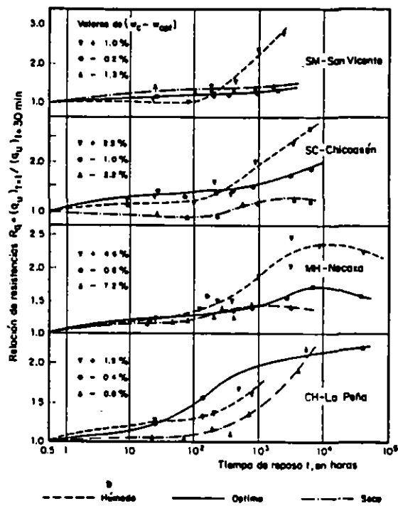
Fig. 17 Efecto del tiempo de reposo sobre la resistencia a la compresión no confinada de suelos compactados por amasado (25-10-10)
