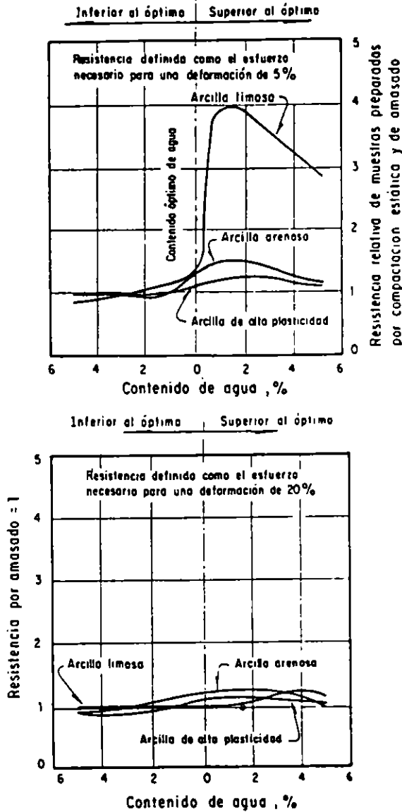
Fig 11. Efectos de procedimientos de compactación en la resistencia en prueba rápida (saturación previa de muestras compactadas a mismos \gamma_c y w ) con compactación estática y de amasado.
