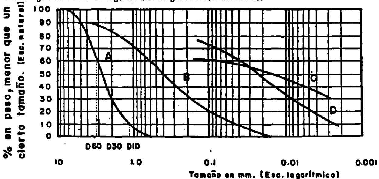
Figura 1 Curvas granulométricas de algunos suelos. A) Arena muy uniforme de Ciudad Cuauhtémoc, México. B) Suelo bien graduado, Puebla, México. C) Arcilla del Valle de México (curva obtenida con hidrómetro) D) Arcilla del Valle de México (curva obtenida con hidrómetro).
