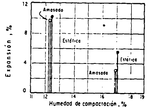
Fig 3. Compresibilidad y expansividad de un suelo arcilloso compactado a una misma relación de vacíos con contenidos de agua a ambos lados del óptimo.
