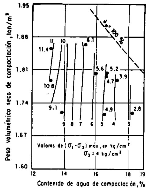
Fig 9. Líneas de igual resistencia a 1 compresión en prueba rápida, si saturación previa y con presión confinante de 4 \text{ kg/cm}^2 .
