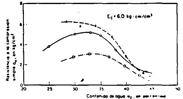
Fig. 7 Efecto de la granulometría del suelo MH-Necaxa seco sobre el \gamma_d y la resistencia en compresión simple. Compactación por impacto
