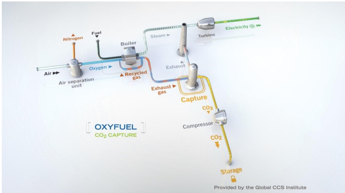
Figura 3.5 Sistema de Oxi-Combustión, (Global CCS institute, 2015)
