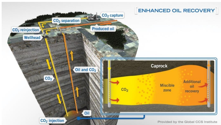
Figura 3.12 Almacenamiento de CO 2 por EOR, (Global CCS Institute, 2015)
