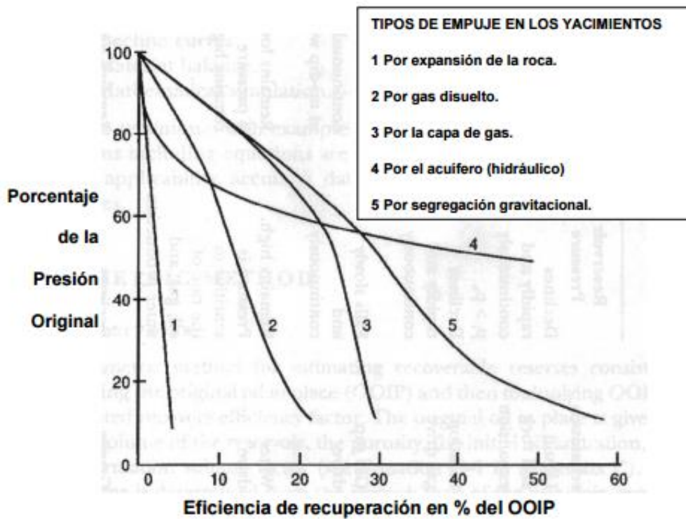
Figura 1.3 Influencia de los mecanismos de empuje, (Documento técnico 1 CNH, 2010)
