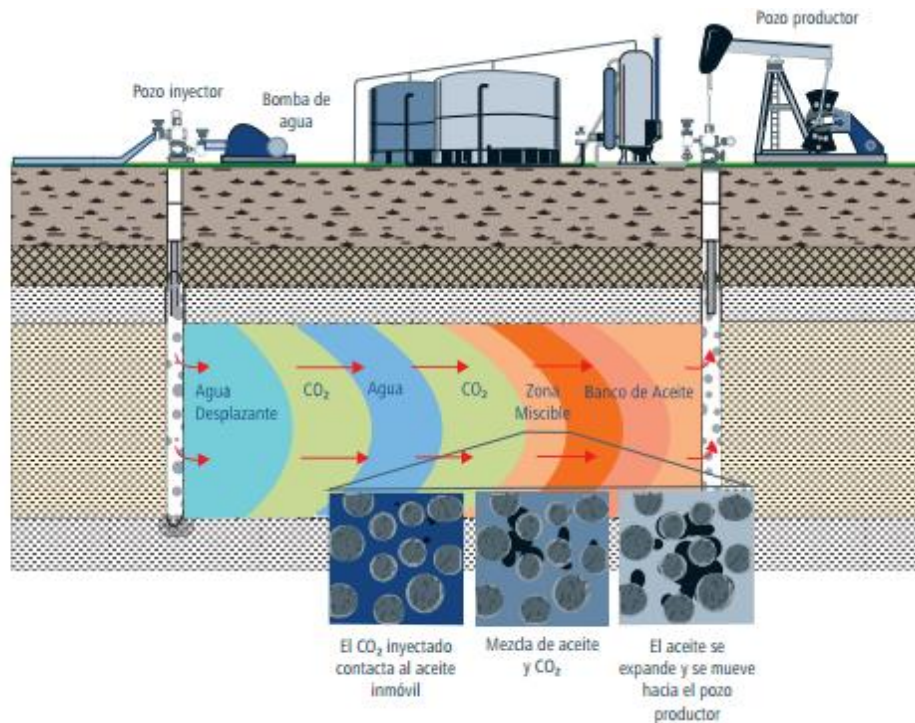
Figura 3.17 Inyección de CO 2 , (National Energy Technology Laboratory, 2010)
