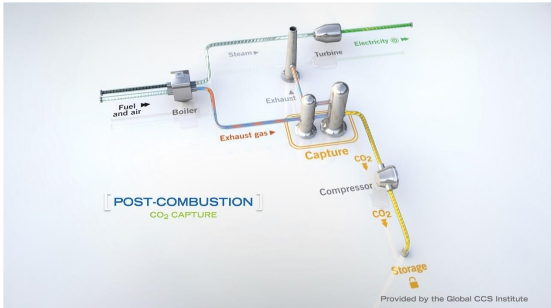
Figura 3.3 Sistema de Post-Combustión, (Global CCS Institute, 2015)
