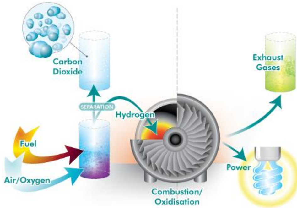
Figura 3.2 Esquema de la captura de CO 2 por pre-combustión, (CO 2 Cooperative Research Centres, 2014).
