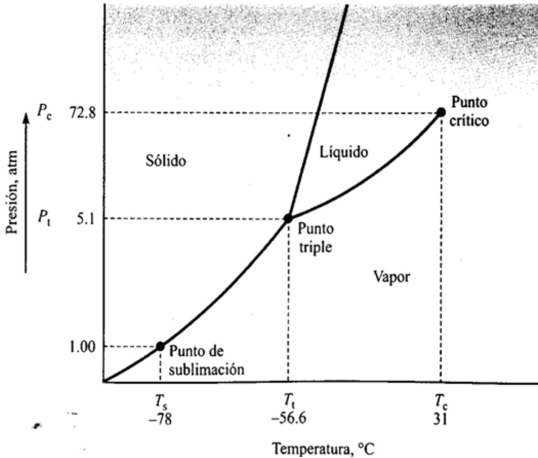
Figura 1.1 Diagrama de fases del CO 2 , (www.iaea.org 2007).
