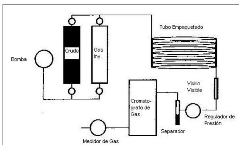
Figura 3.19 Esquema del slim tube
