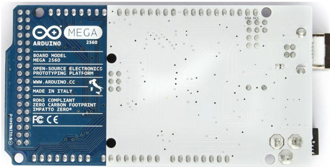
Figura 2.3.2 Placa de Arduino Mega 2560 trasera, en la parte superior derecha se encuentran la posición de los pines SDA y SCL
