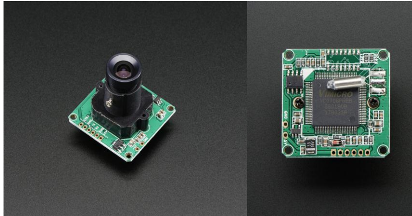
Figura 3.4.7 Cámara VC0706 vista ambos lados
