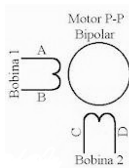
Figura 3.4.10 Modelo de motor bipolar
