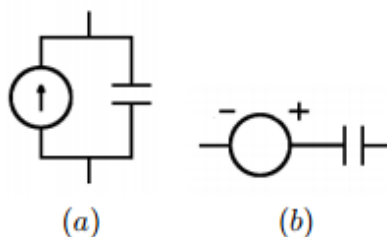
Figura 2.4. 2. Modelos de un sensor piroeléctrico.
