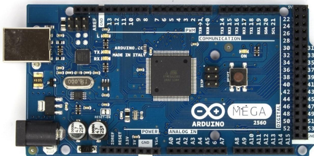
Figura 2.3.1 Placa de Arduino Mega 2560 frontal
