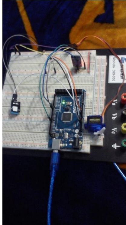
Figura 4.1.5 Tarjeta Arduino y los componentes en su fase inicial.
