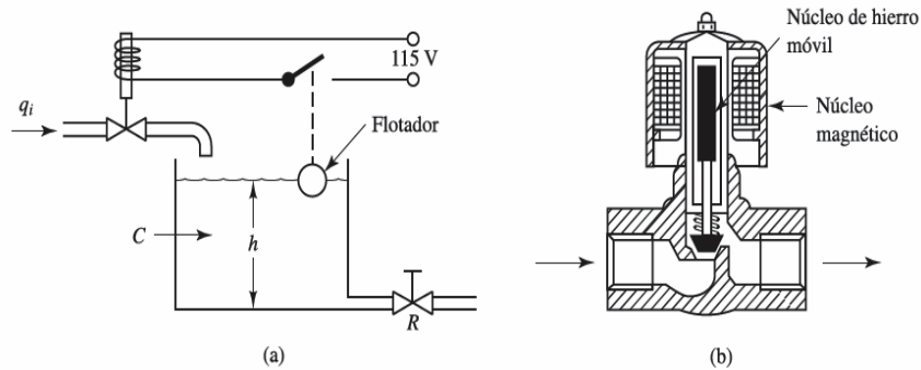
Figura 2.2.2 (a) Sistema de control de nivel de líquidos; (b) válvula electromagnética.
