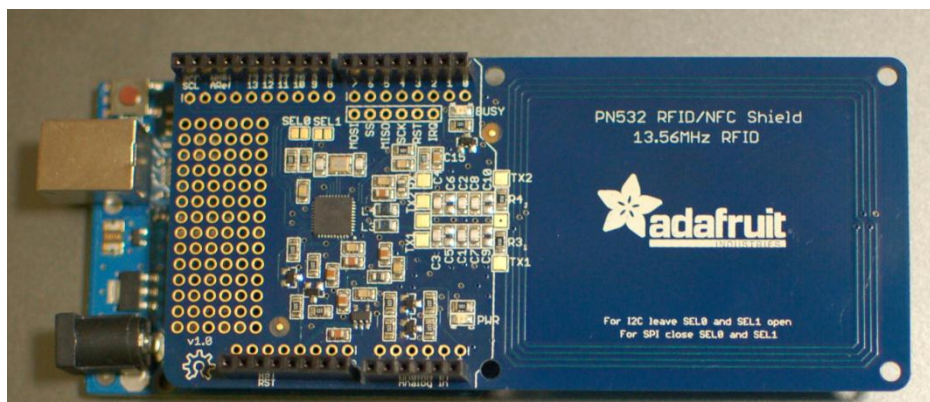
Figura 4.1.8 Módulo PN532 colocado sobre tarjeta Arduino
