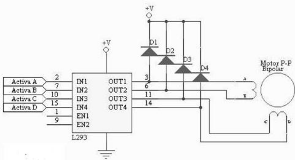
Figura 3.4.13 Conexión de motor a pasos bipolar con circuito L293
