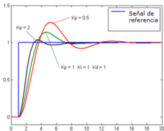
Figura 2.2.4. Ganancia proporcional aplicada a una señal.
