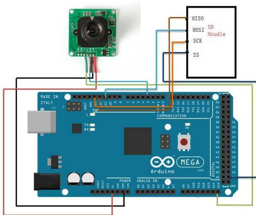
Figura 4.1.9 Diagrama de conexión para la cámara
