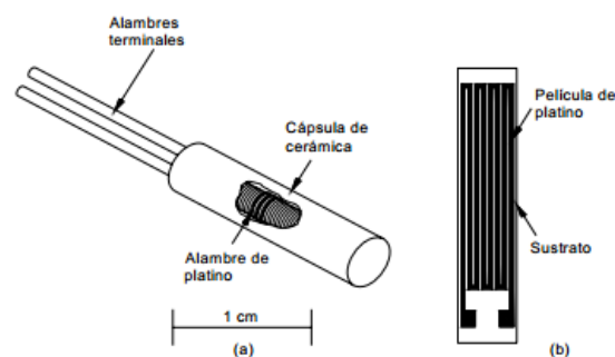
Figura 2.4. 3. Sensor RTD.
