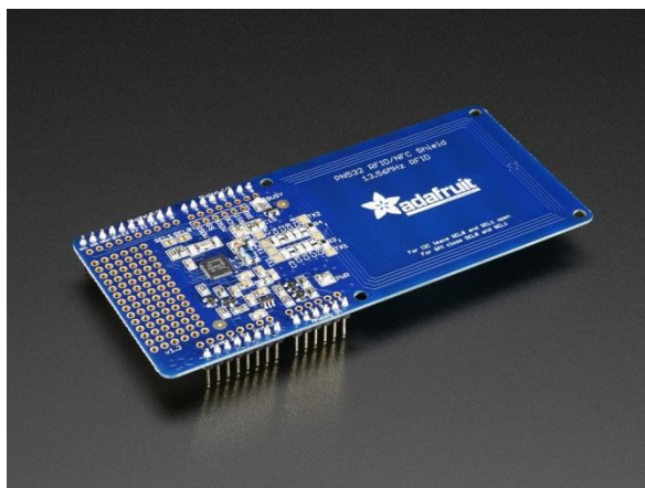
Figura 3.4. 10 Modulo RFID y NFC.
