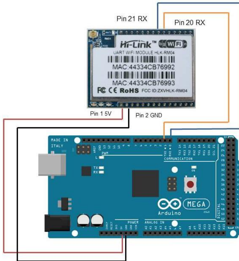
Figura 4.1.12 Esquema de conexiones para el módulo WiFi
