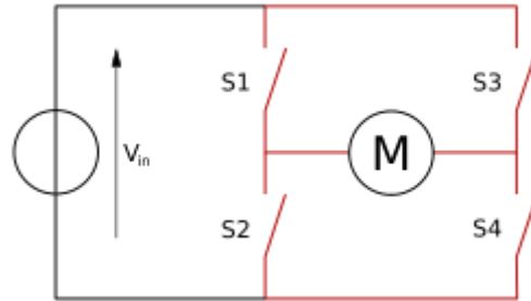
Figura 3.4.15 Conexión en Puente H
