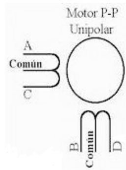
Figura 3.4.11 Modelo de motor unipolar
