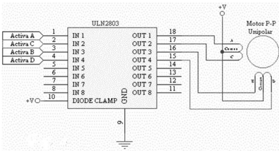
Figura 3.4.14 Conexión de motor a pasos unipolar con circuito ULN2803
