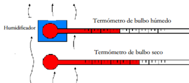
Figura 2.4. 5. Diferencia de psicometría entre bulbo húmedo y seco.
