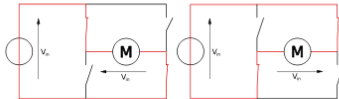
Figura 3.4.16 Los 2 estados básicos del circuito.
