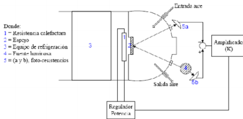
Figura 2.4. 6 Sensor por condensación.
