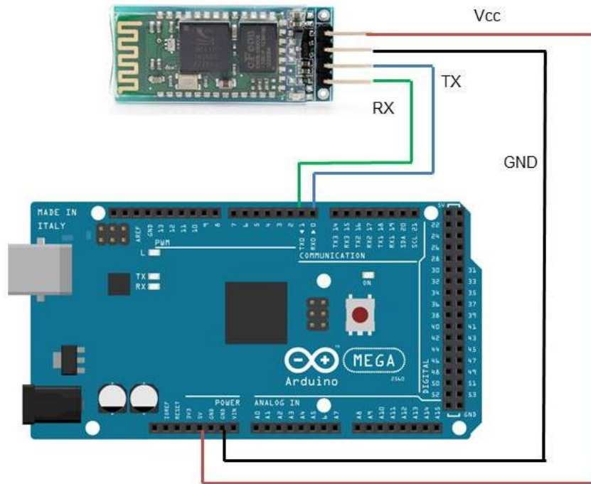
Figura 4.1.3 Esquema de conexión módulo HC-06
