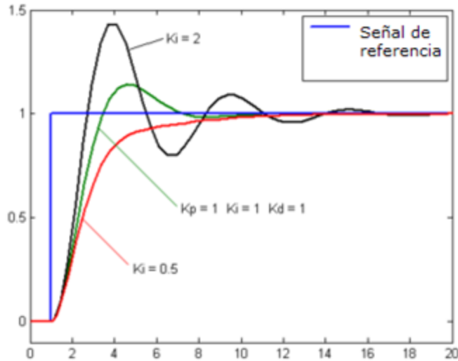
Figura 2.2.5. Control integral aplicado a una señal.
