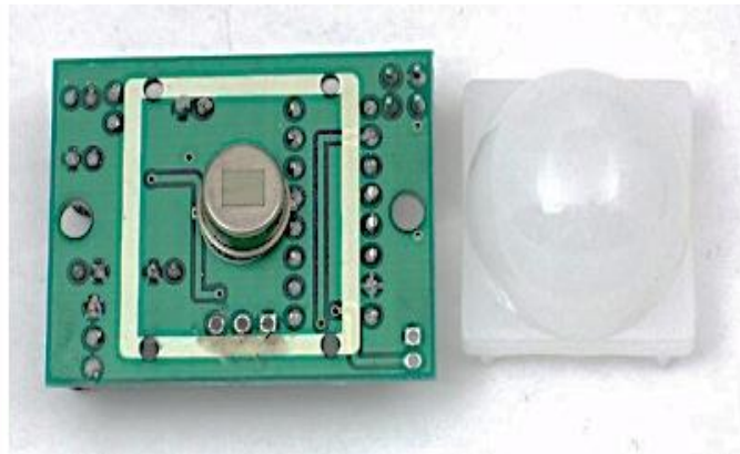
Figura 4.3.3 Sensor PIR.
