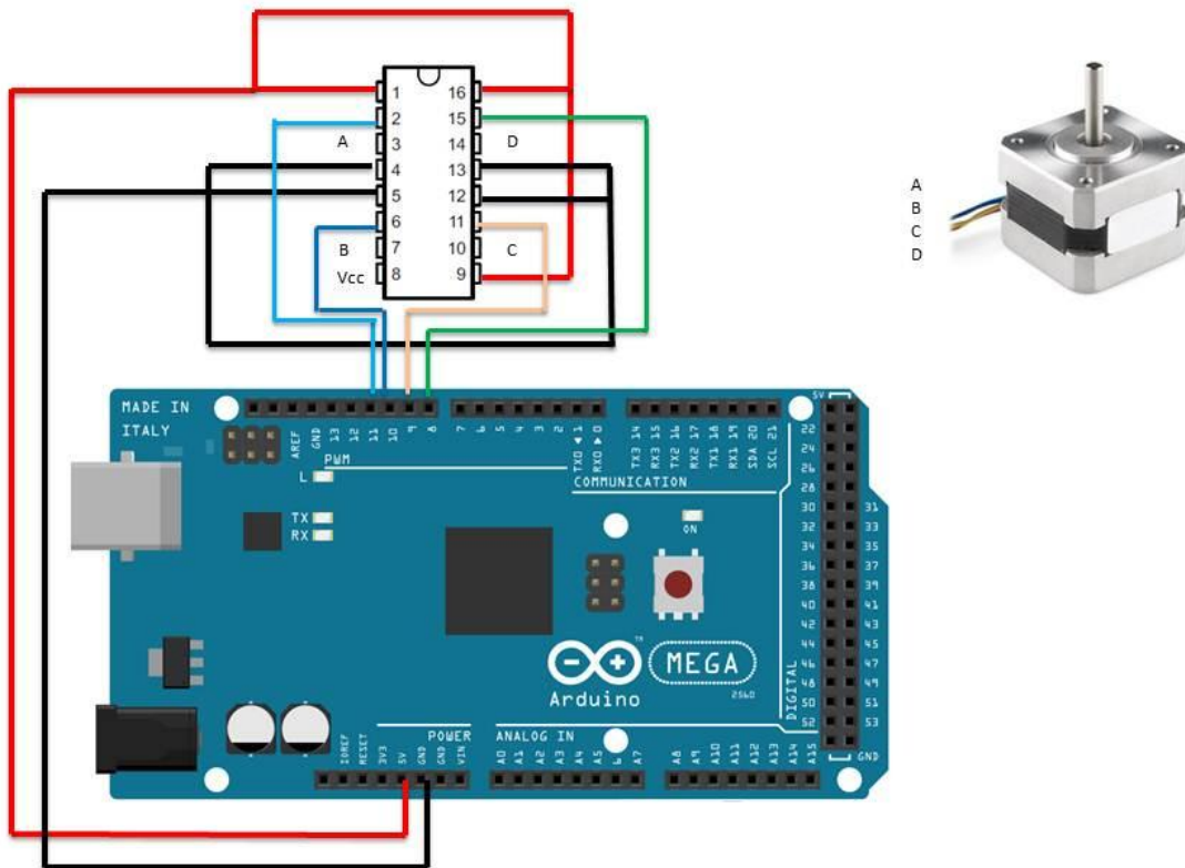
Figura 4.1.6 Tarjeta Arduino y la conexión con el motor a pasos con un puente H
