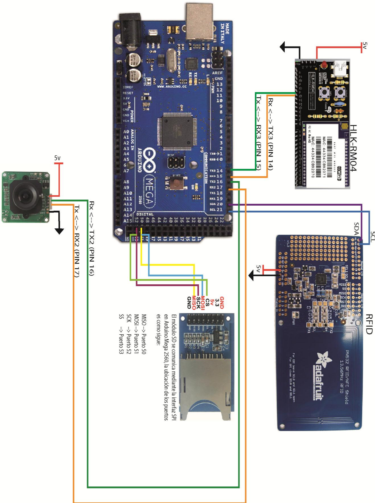
Diagrama de Bloques del sistema de monitoreo y control.
