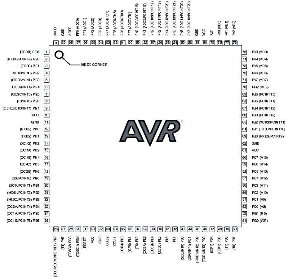
Figura 2.3.3 Circuito ATmega 2560 y su distribución de pines en la tarjeta.
