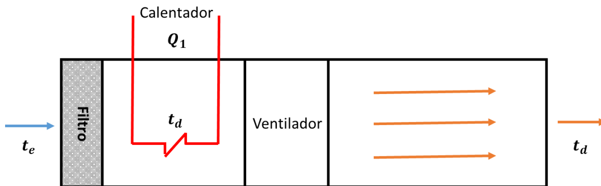
Fig. 3. 15 Calefacción central, funcionamiento general
