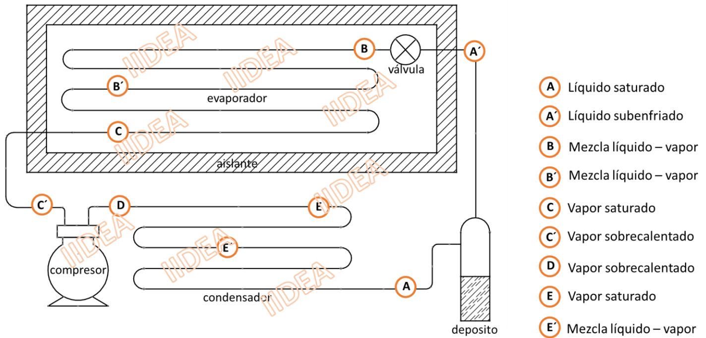
Fig. 3. 17 Sistema típico de refrigeración vapor - compresión
