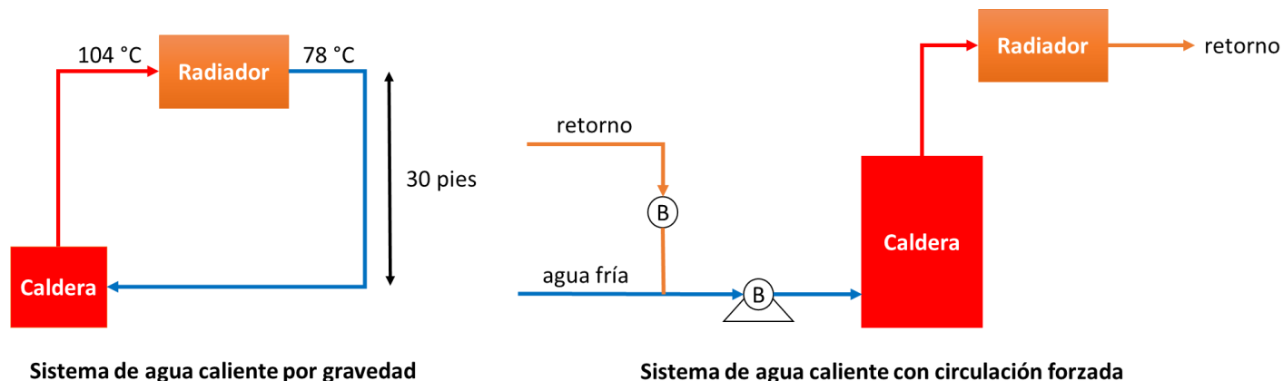
Fig. 3. 14 Sistemas de calefacción, mediante agua caliente
