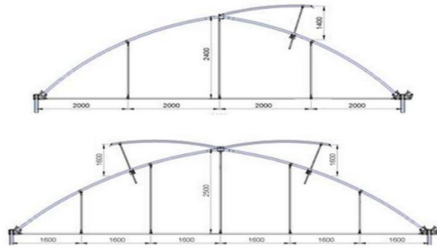
Arcos ojivales galvanizados
