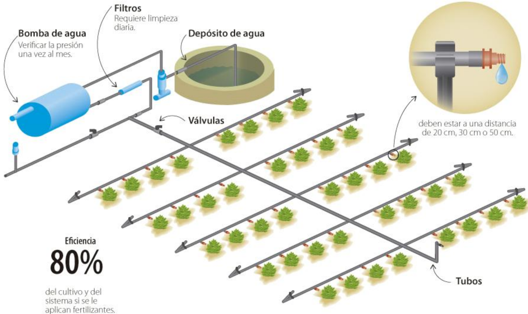
Fig. 3. 7 Sistema de Riego localizado automatizado
