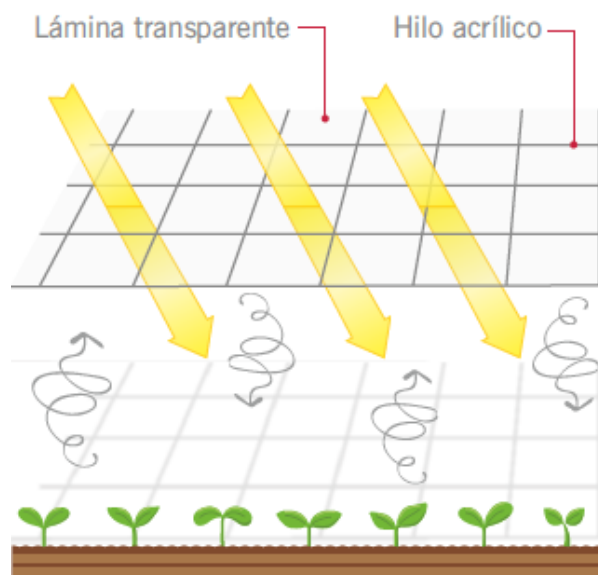
Fig. 3. 10 Pantalla térmica [47]
