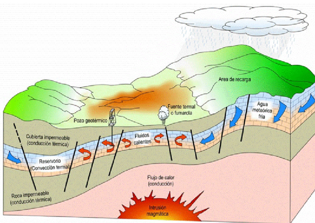
Fig. 1. 9 Representación esquemática del modelo de yacimiento geotérmico [2]
