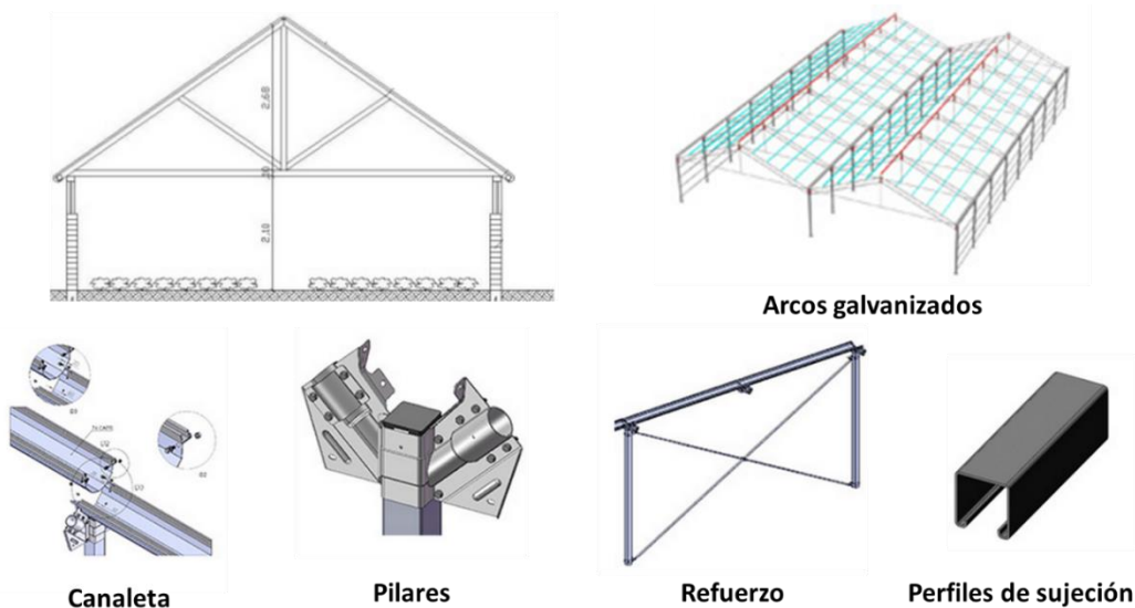
Fig. 2. 8 Estructura de un Invernadero tipo capilla a dos aguas
