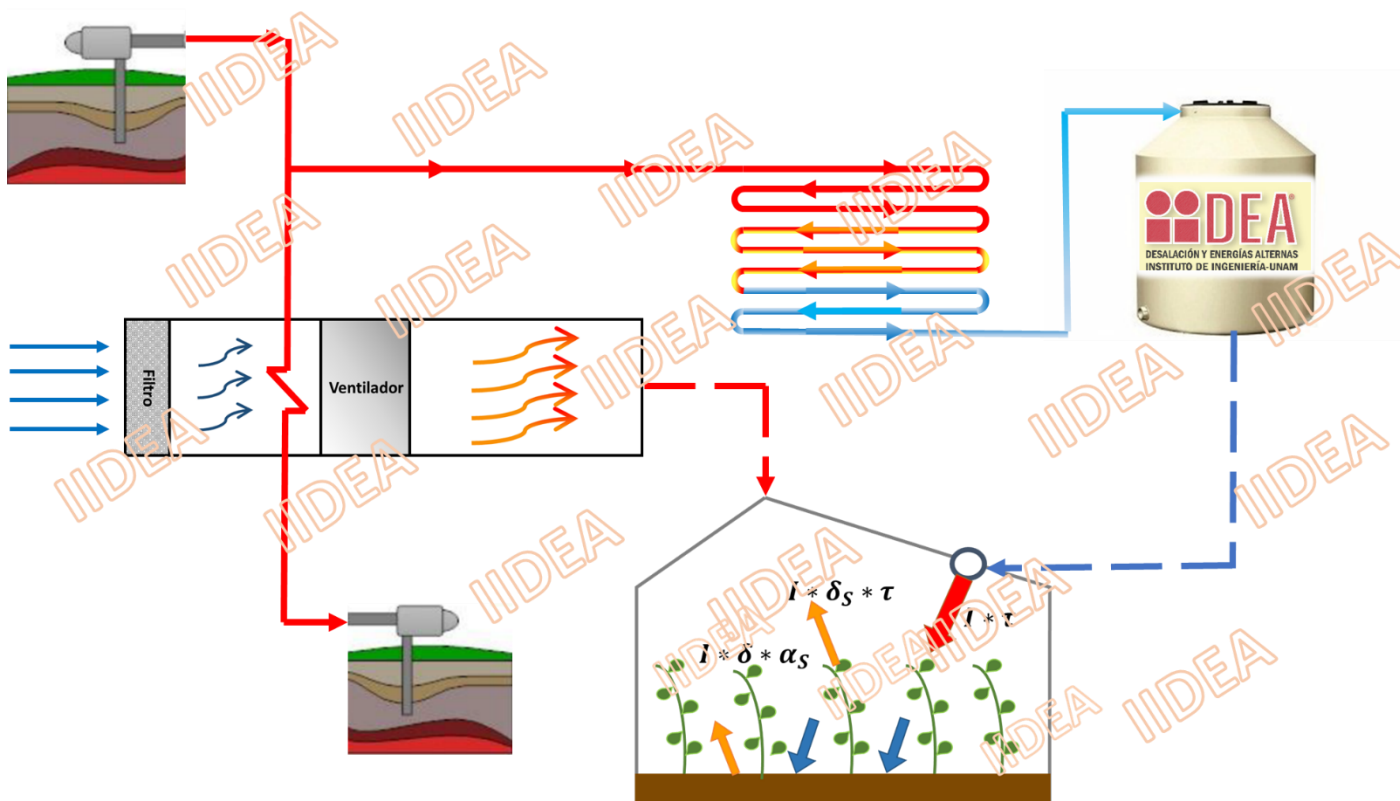
Fig. 4 1 Diagrama de los procesos térmicos involucrados dentro del invernadero
