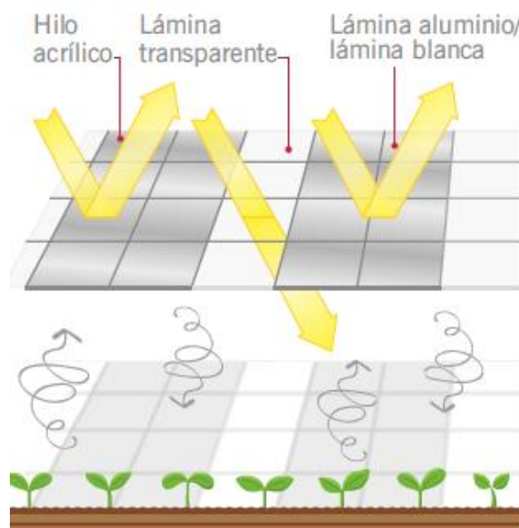
Fig. 3. 11 Pantalla termorefectiva [47]
