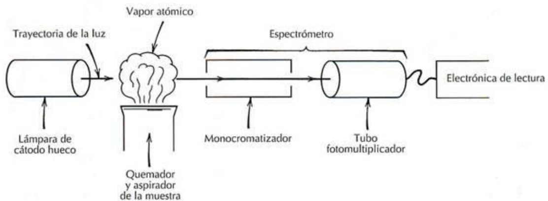
FIGURA 3.5 ESQUEMA DEL EQUIPO DE ESPECTROSCOPIA DE ABSORCIÓN ATÓMICA
