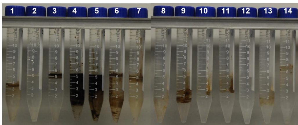
FIGURA 4.2 FLUIDOS PRODUCIDOS DURANTE INYECCIÓN DE SALMUERA BS (AS DILUIDA A 1/100)
