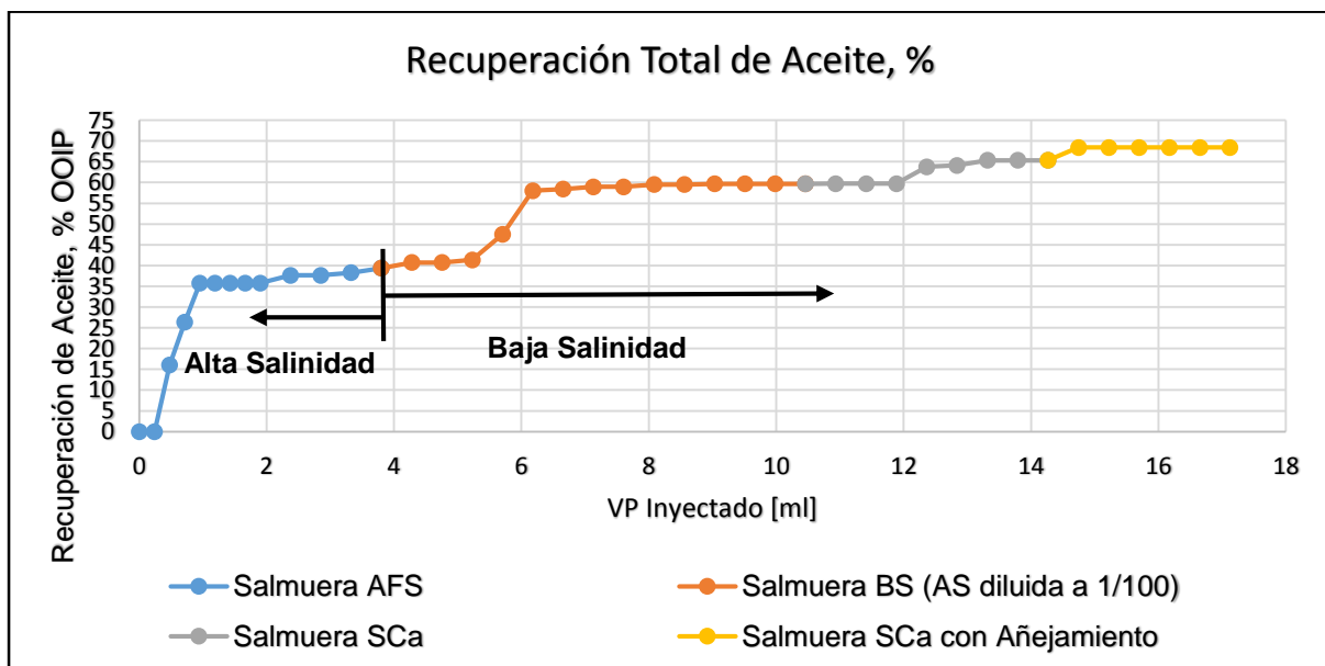
FIGURA 4.6 PORCENTAJE DE ACEITE ACUMULADO POR ETAPA
