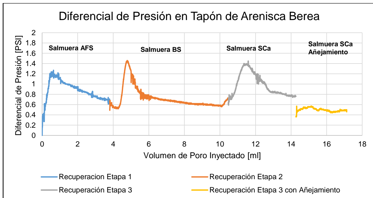
FIGURA 4.9 COMPORTAMIENTO DE LA DIFERENCIAL DE PRESIÓN DURANTE CADA ETAPA DE LA PRUEBA DE DESPLAZAMIENTO
