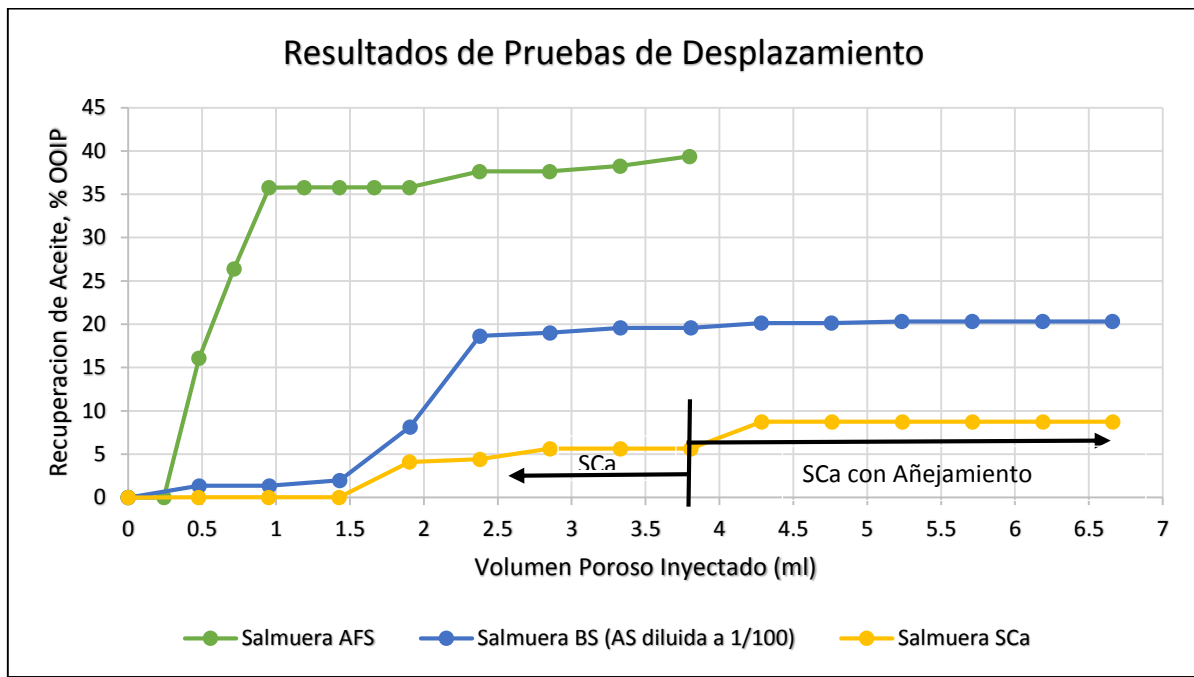
FIGURA 4.5 VOLUMEN DE ACEITE RECUPERADO EN PORCENTAJE POR ETAPA DE INYECCIÓN
