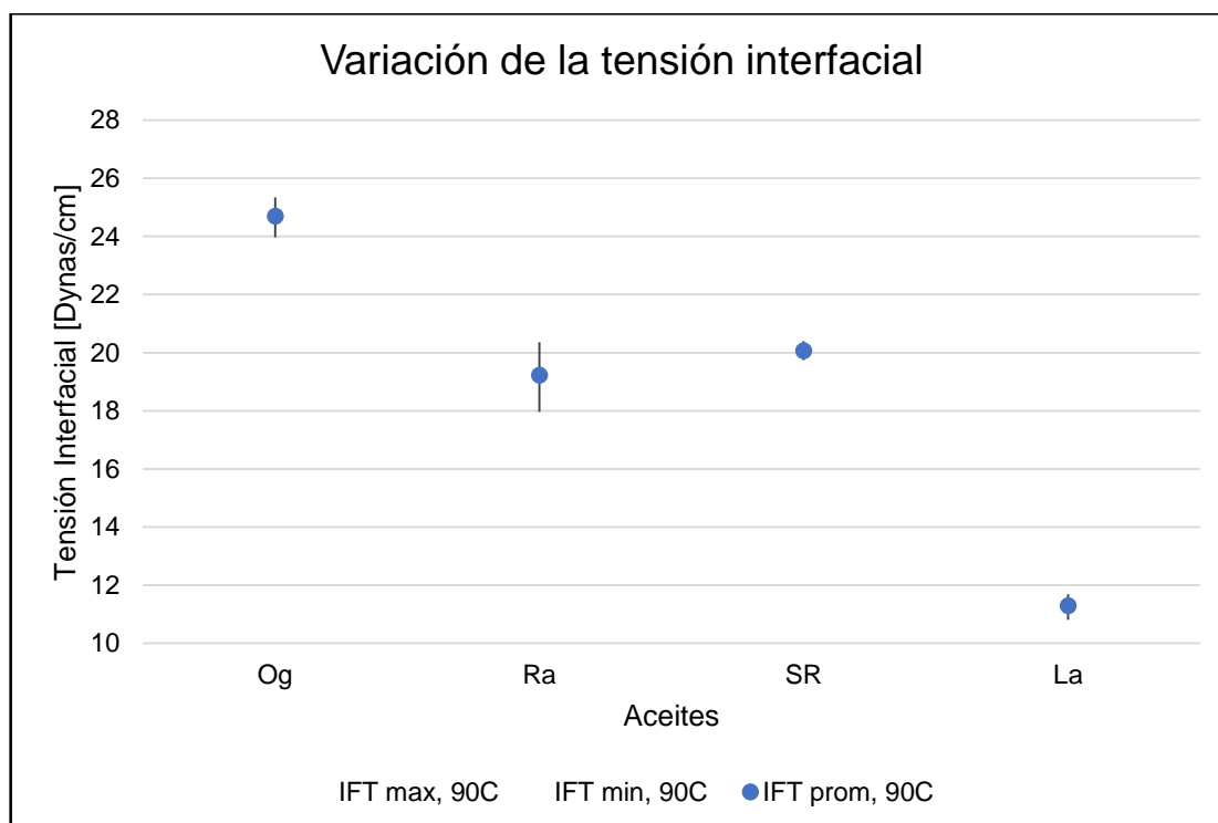
FIGURA 4.7 VARIACIÓN DE LA TIF (MIN, MAX Y PROMEDIO) ENTRE SALMUERAS Y ACEITES A 90° C
