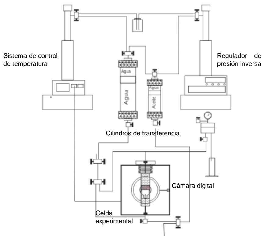
FIGURA 3.2 EQUIPO PARA TOMA DE MEDICIONES DE TENSIÓN INTERFACIAL
