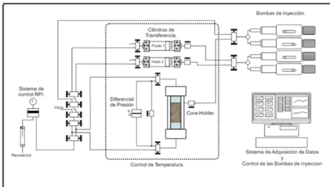
FIGURA 3.3 ESQUEMA DEL SISTEMA DE INYECCIÓN UTILIZADO PARA PRUEBA DE DESPLAZAMIENTO
