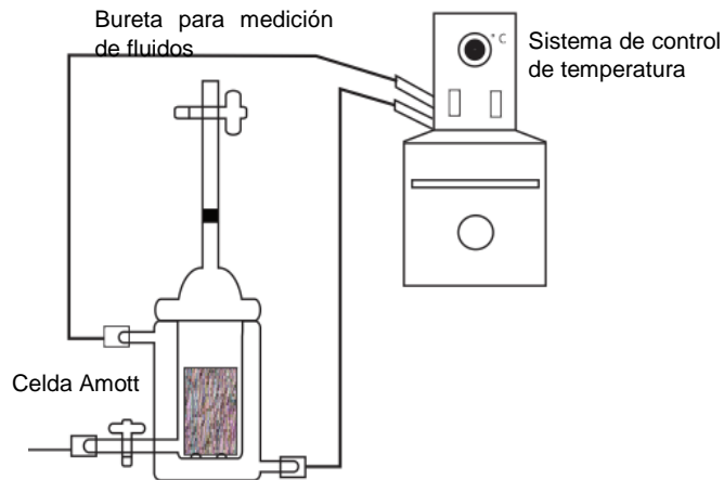
FIGURA 3.4 EQUIPO AMOTT UTILIZADO PARA PRUEBA DE IMBIBICIÓN ESPONTÁNEA
