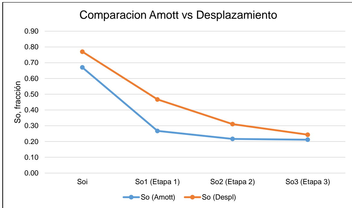
FIGURA 4.8 COMPARACIÓN DE LA SATURACIÓN RESIDUAL DE ACEITE POR ETAPA ENTRE PRUEBAS DE IMBIBICIÓN ESPONTÁNEA Y DE DESPLAZAMIENTO
