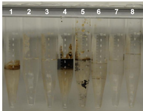
FIGURA 4.3 FLUIDOS PRODUCIDOS DURANTE INYECCIÓN DE SALMUERA SCA
