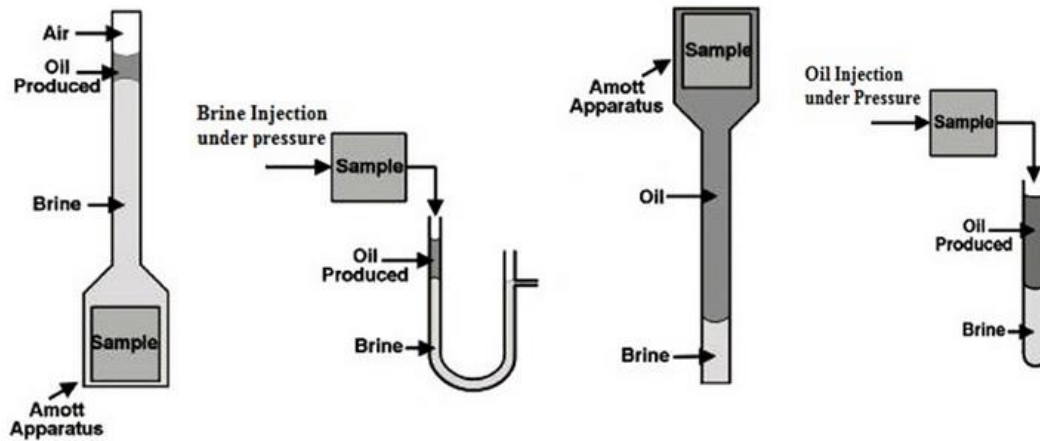
FIGURA 3.7 MEDICIONES OBTENIDAS DURANTE PRUEBA DE AMOTT
