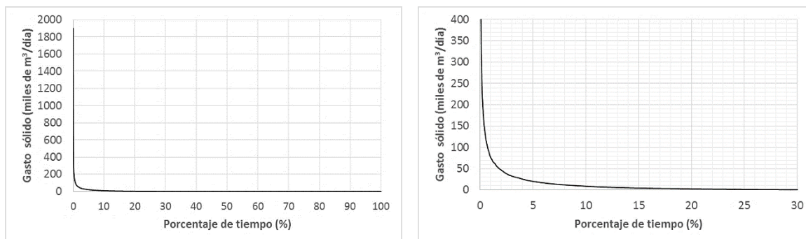
Figura 5.8. Curva de duración
