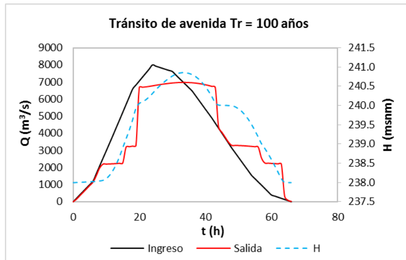
Figura 4.23. Tránsito de avenida Tr = 100 años
