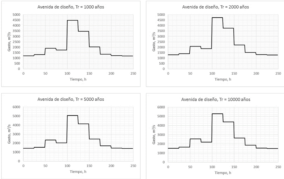
Figura 4.7. Avenida de diseño para diferentes períodos de retorno
