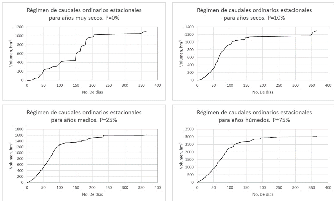
Figura 6.1. Regímenes de caudales ordinarios estacionales
