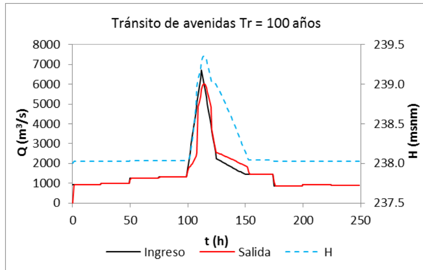
Figura 4.19. Tránsito de avenida Tr = 100 años
