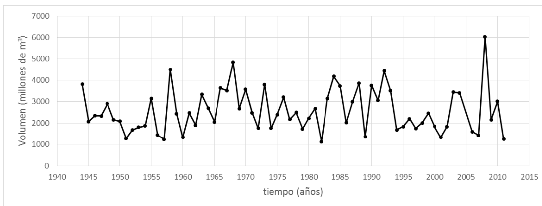
Figura 7.2. Volumen total anual en la P.H. Las Cruces
