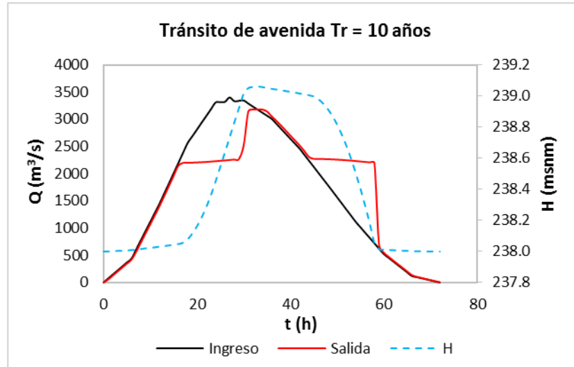
Figura 4.22. Tránsito de avenida Tr = 10 años
