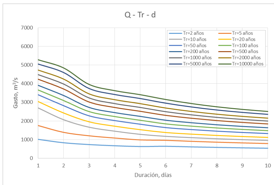
Figura 4.6. Curva Q-Tr-d
