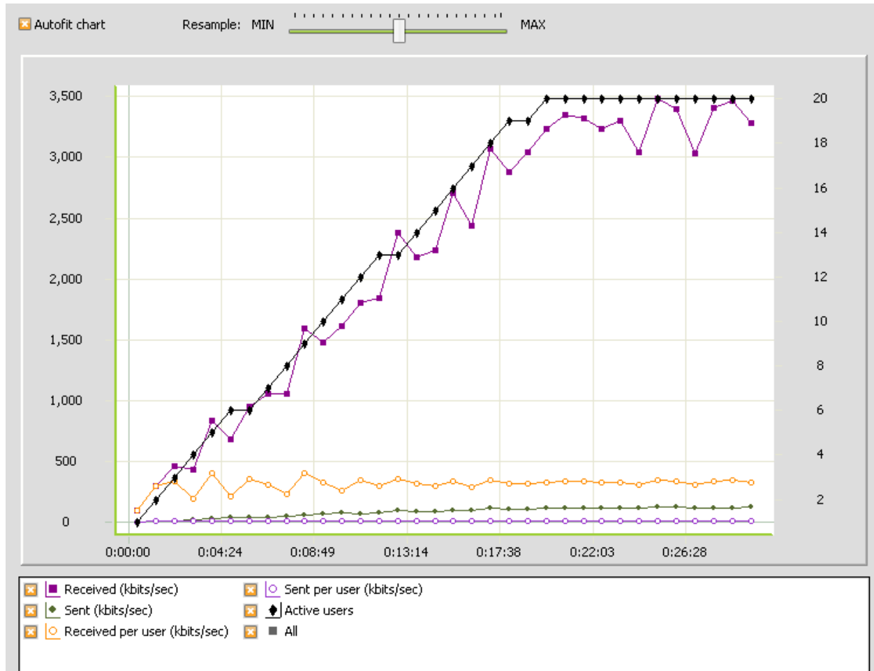
Figura 6—5 Gráfica con mayor detalle del ancho de banda utilizado durante la prueba.
