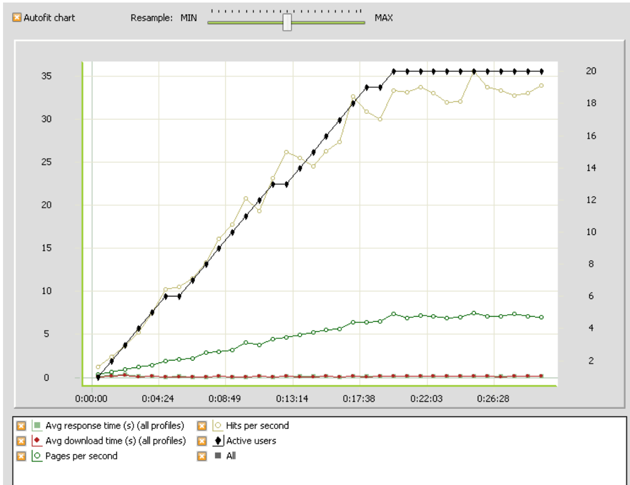
Figura 6—4 Gráfica con mayor detalle del desempeño durante la prueba.
