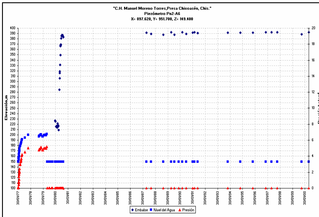
Gráfica 3.8 Nivel de agua en piezómetro neumático Pn2-A6
