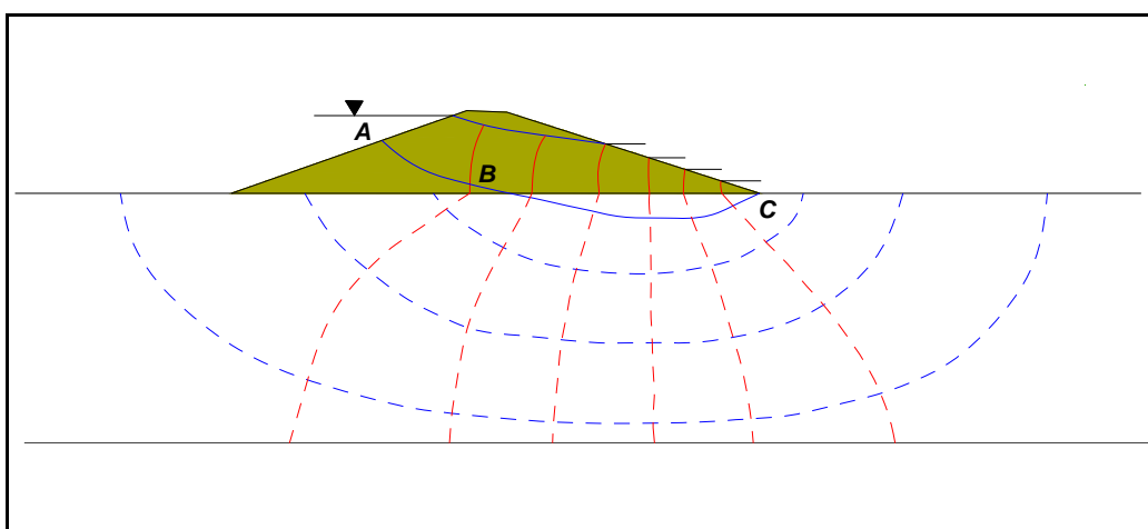
Figura 2.11 Ajuste de líneas equipotenciales y de flujo para el balance de la red dibujada
