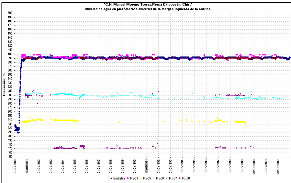
Gráfica 1.7 Niveles de agua en piezómetros abiertos de la Margen Izquierda Pz-53 a Pz-58
