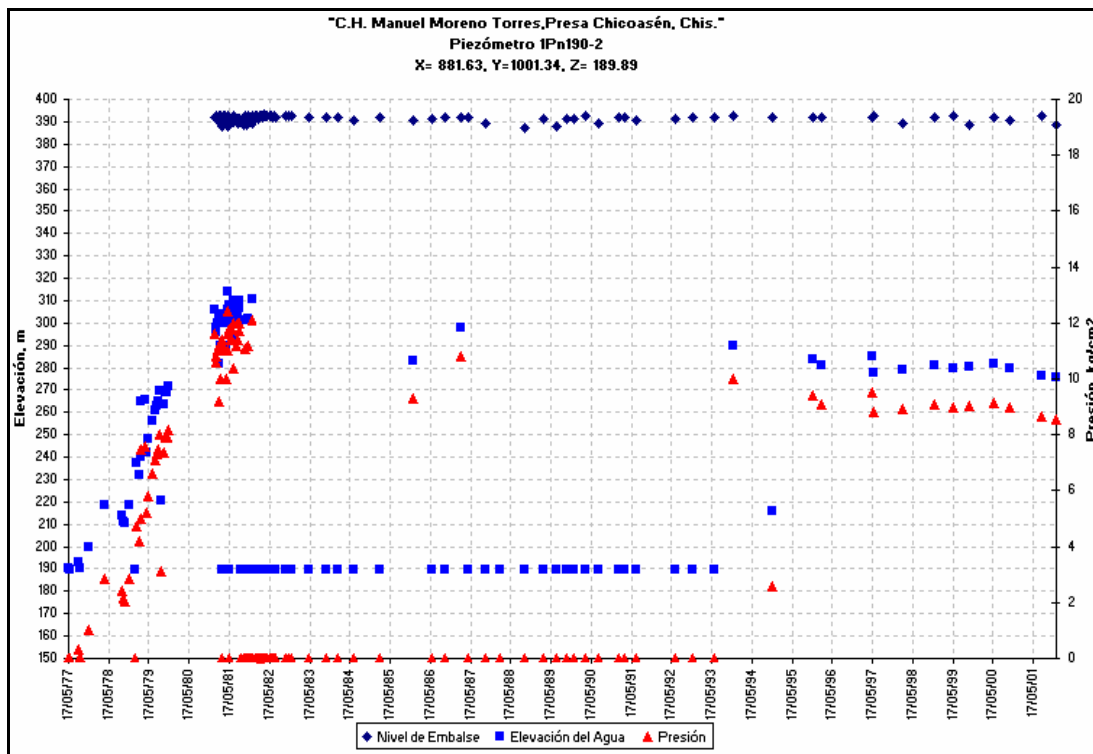
Gráfica 3.12 Nivel de agua en piezómetro neumático 1Pn190-2
