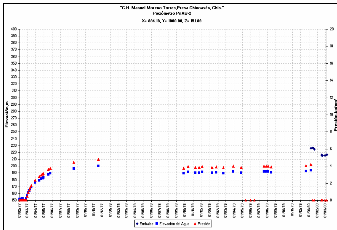
Gráfica 3.6 Nivel de agua en piezómetro neumático PnAB-2
