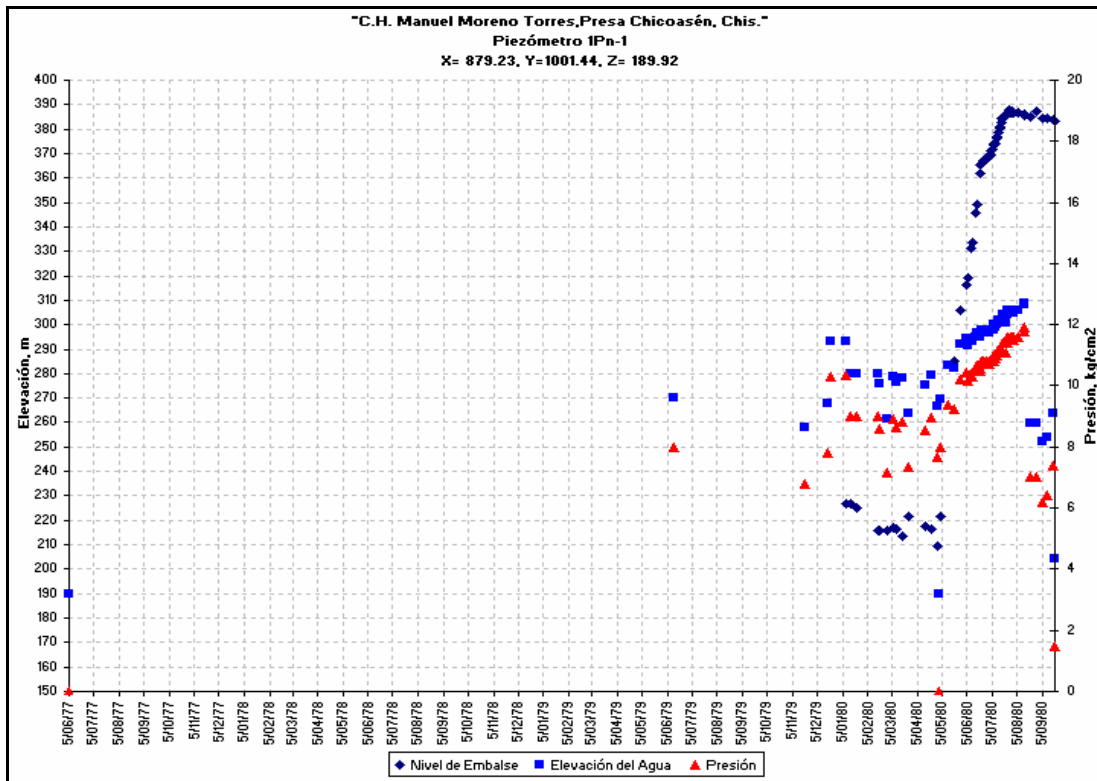
Gráfica 3.9 Nivel de agua en piezómetros neumáticos 1Pn-1
