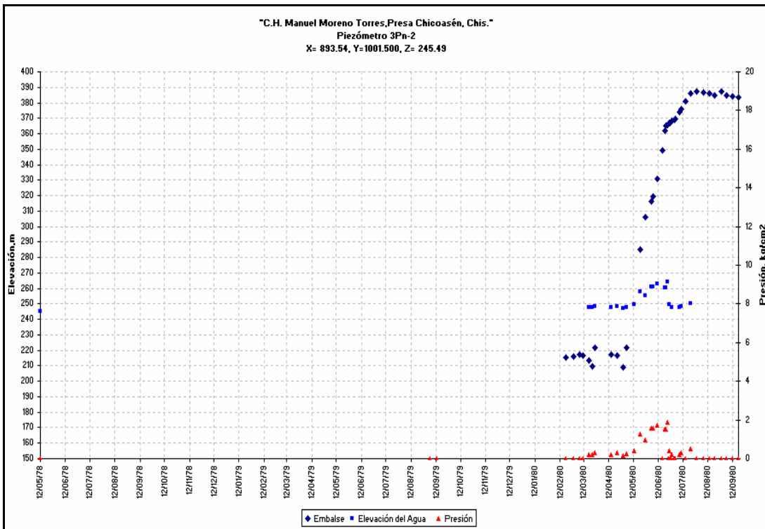
Gráfica 3.14 Nivel de agua en piezómetro neumático 3Pn-2
