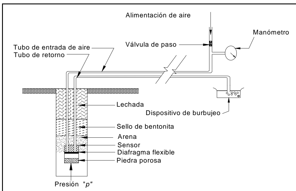
Figura 1.15 Principio de medición del piezómetro neumático
