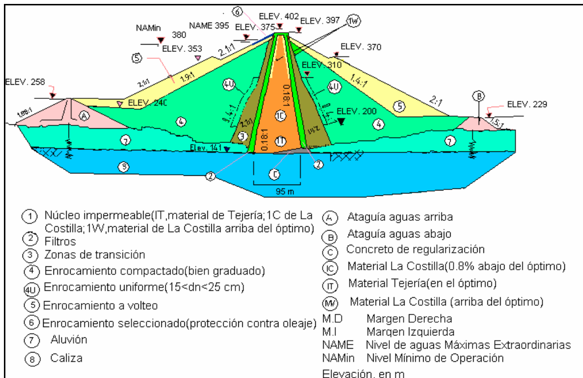
Figura 1.6 Sección transversal máxima
