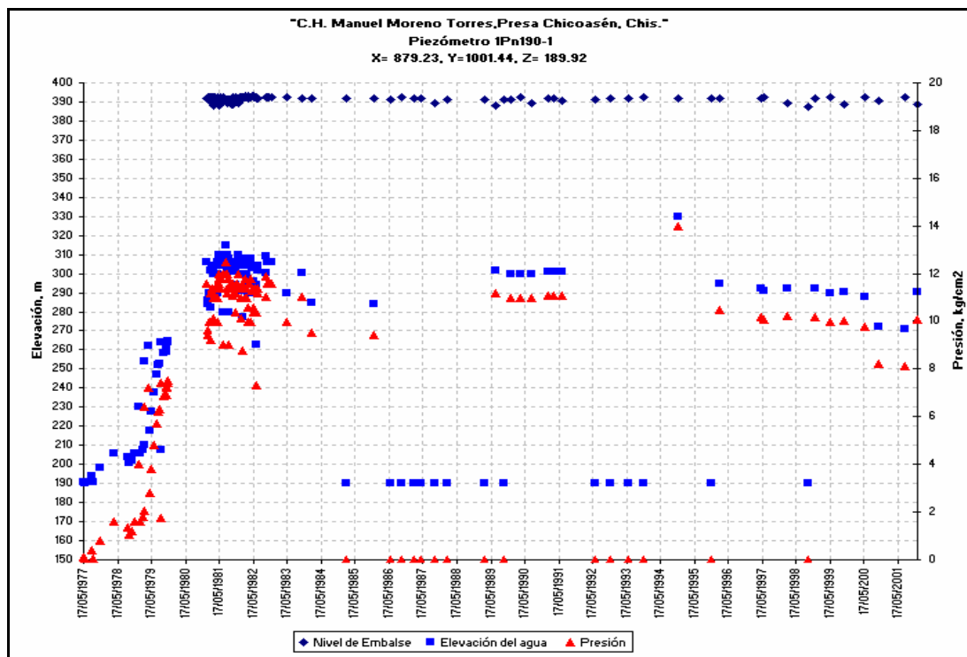
Gráfica 3.11 Nivel de agua en piezómetro neumático 1Pn190-1
