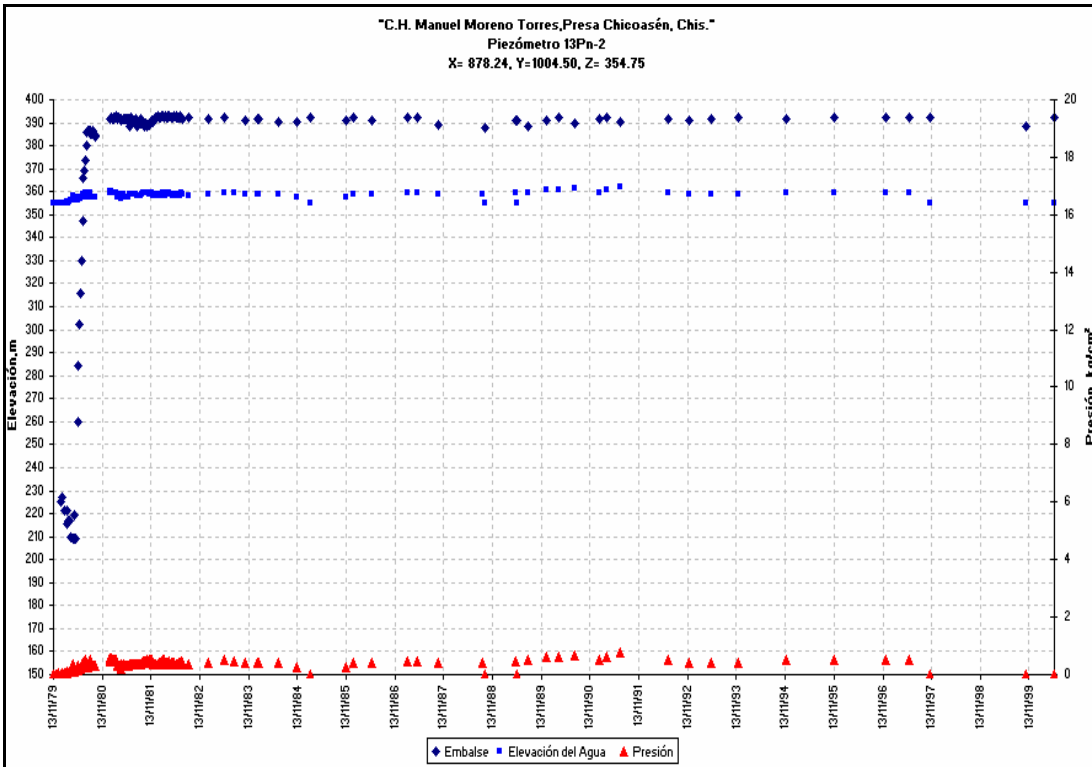
Gráfica 3.19 Nivel de agua en piezómetro neumático 13Pn-2
