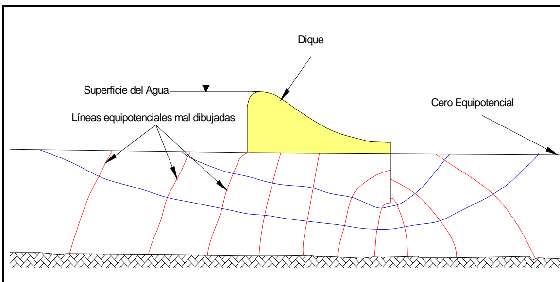
Figura 2.2 Líneas equipotenciales mal dibujadas
