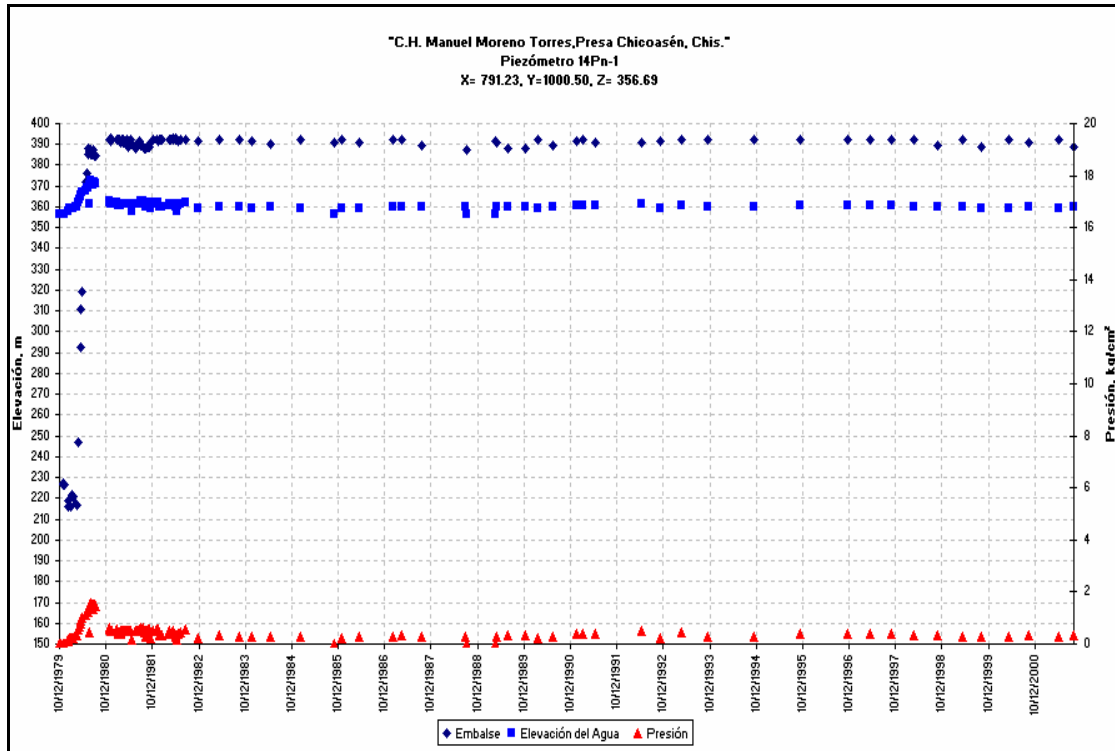
Gráfica 3.20 Nivel de agua en piezómetro neumático 14Pn-1
