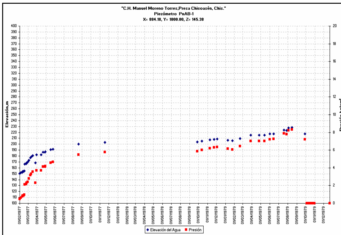
Gráfica 3.5 Nivel de agua en piezómetro neumático PnAB-1
