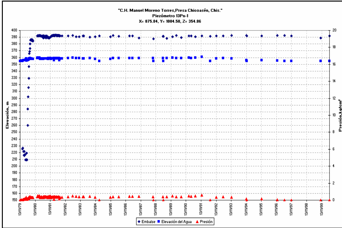
Gráfica 3.18 Nivel de agua en piezómetro neumático 13Pn-1
