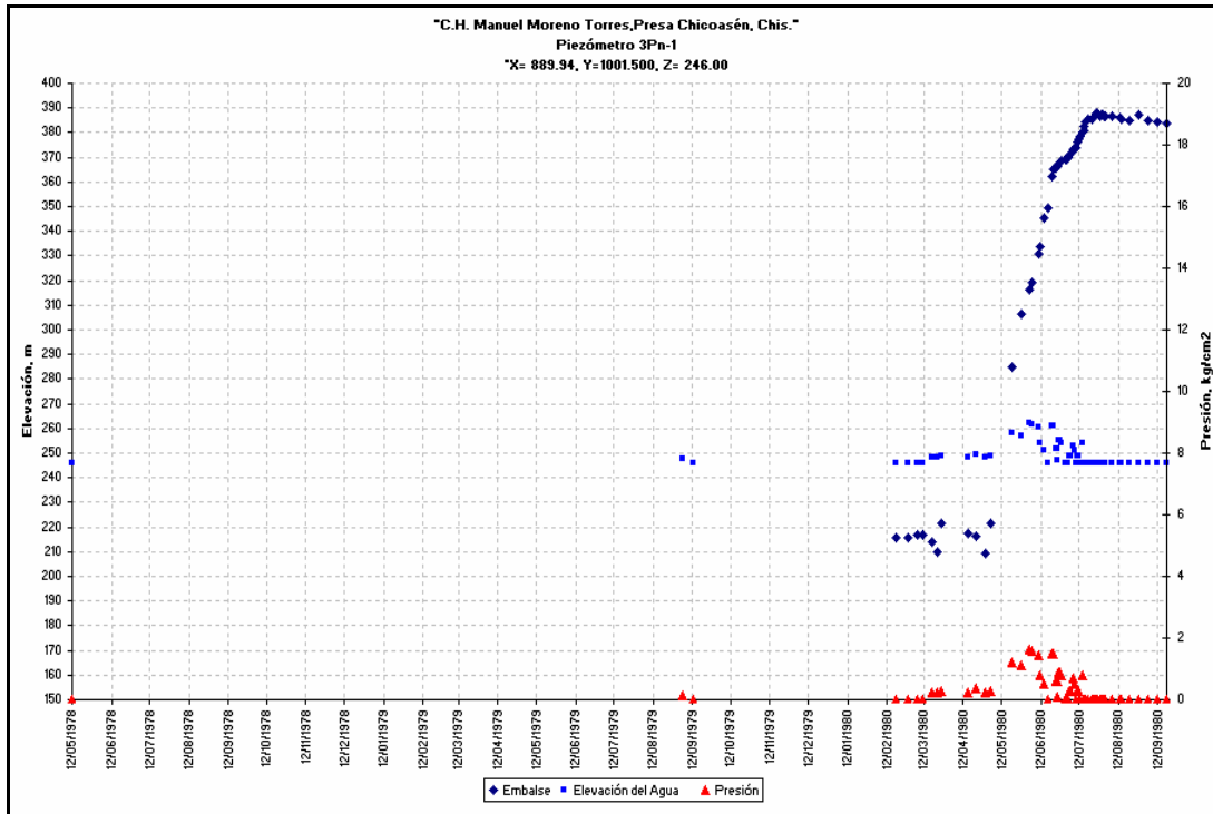
Gráfica 3.13 Nivel de agua en piezómetro neumático 3Pn-1
