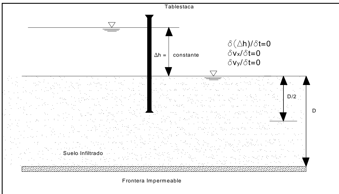
Figura 2.1 Flujo Establecido
