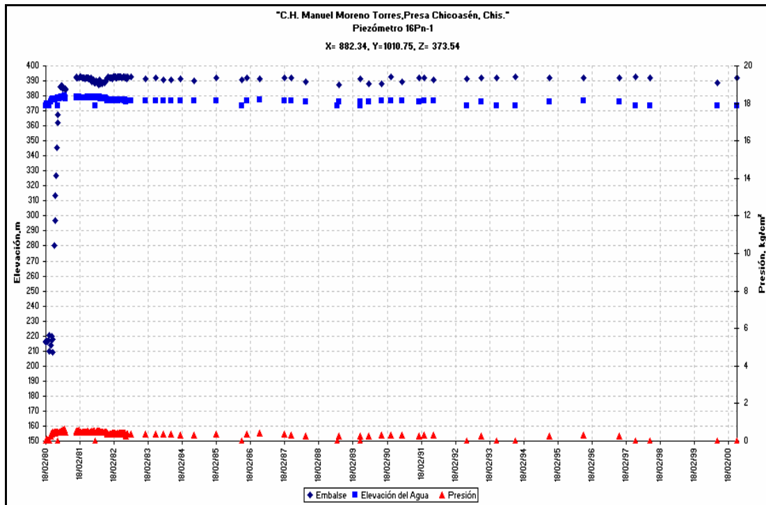
Gráfica 3.24 Nivel de agua en piezómetro neumático 16Pn-1
