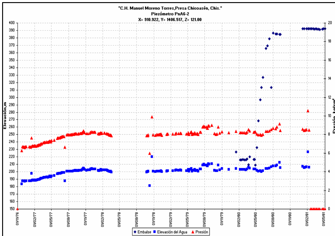
Gráfica 3.28 Niveles de agua en piezómetros neumáticos PnA6-2
