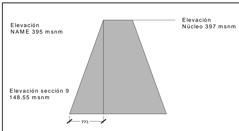
Figura 3.2 Primer paso para obtener la línea de corriente superior
