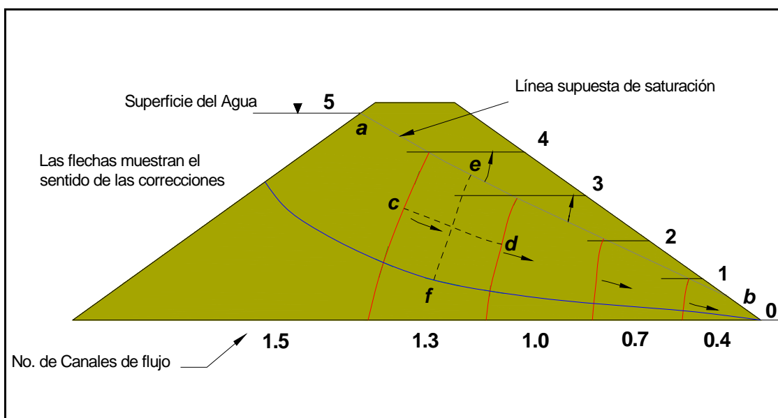
Figura 2.5 Suposición de la línea de saturación
