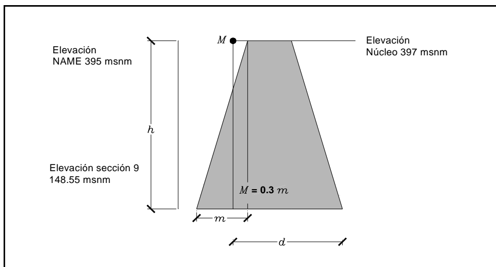
Figura 3.3 Segundo paso para obtener la línea de corriente superior
