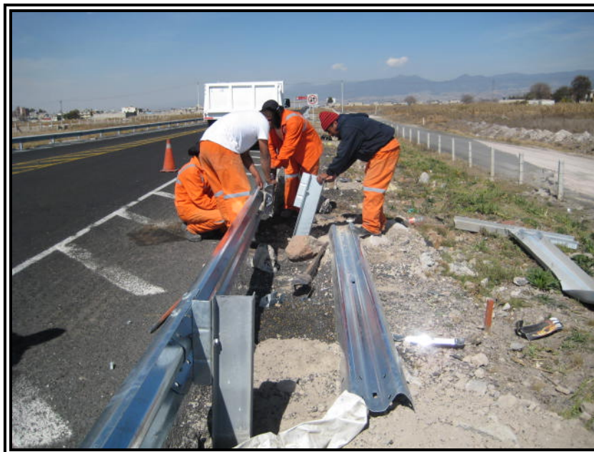
Figura 18. Reparación y sustitución de Defensa Metálica de Protección
